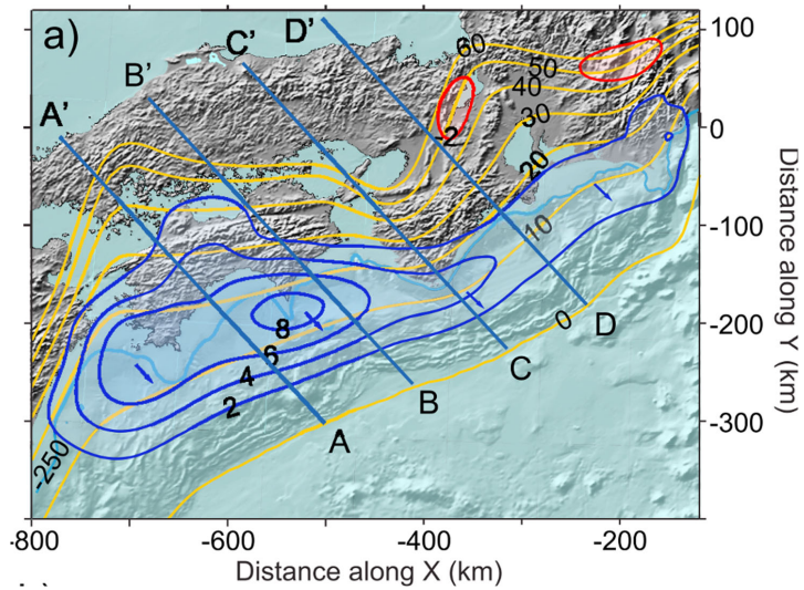
1 . . 2 図 3-36 陸上 GNSS データから推定したプレート間のすべり欠損速度 (Hok et al. , 2011) 3 観測データの期間は 1996~2000 年。すべり欠損速度を青色及び赤色 (forward slip) の等 4 値線 (等値線間隔年間 2 cm), フィリピン海プレート上面の深さを橙色の等値線 (等値線間 5 隔 10 km) 表す。
