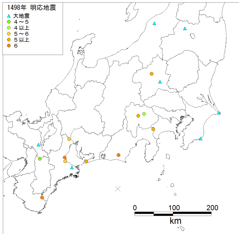
図3-13 1498年明応地震の震度
