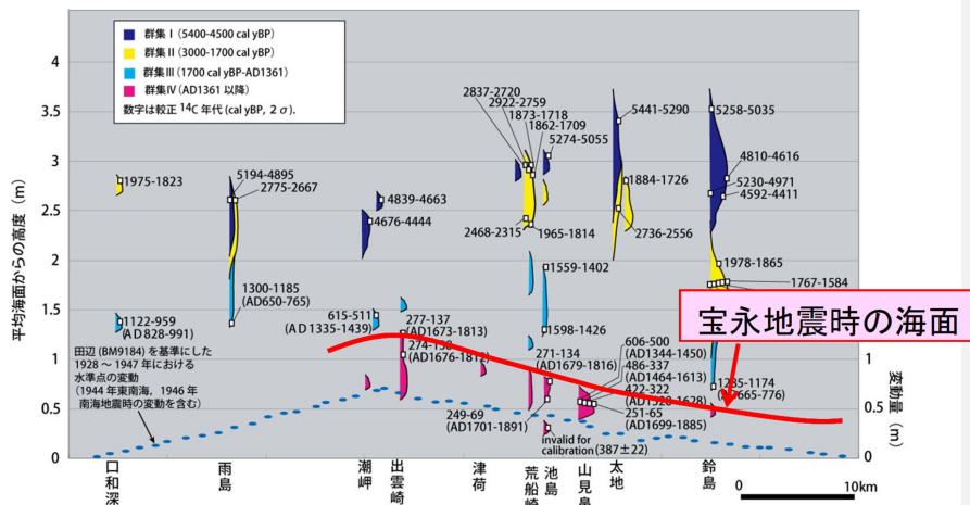
図 3-23 紀伊半島の生物遺骸調査結果（矢倉ほか，2008）
