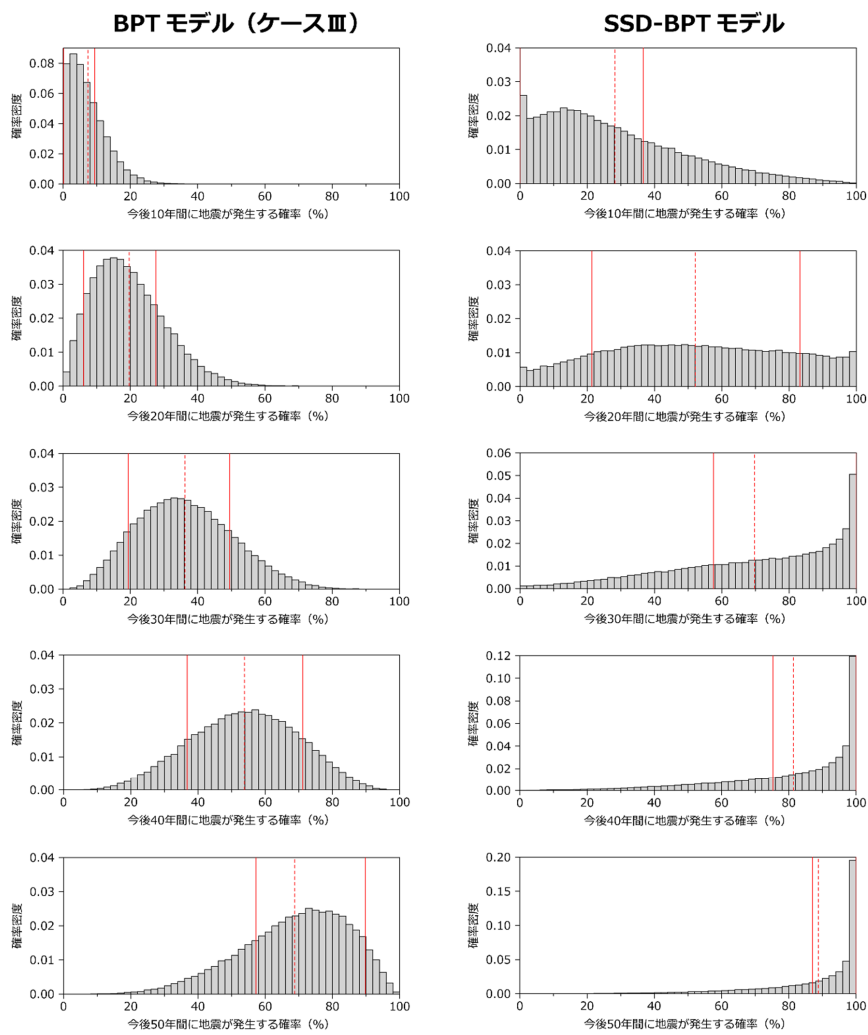
図 4-9 BPT モデルと SSD-BPT モデルによる発生確率の事後分布の比較
