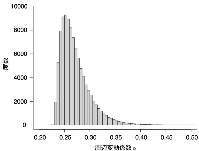
8 9 付図 A-1 : 周辺変動係数 \alpha の頻度分布 10
