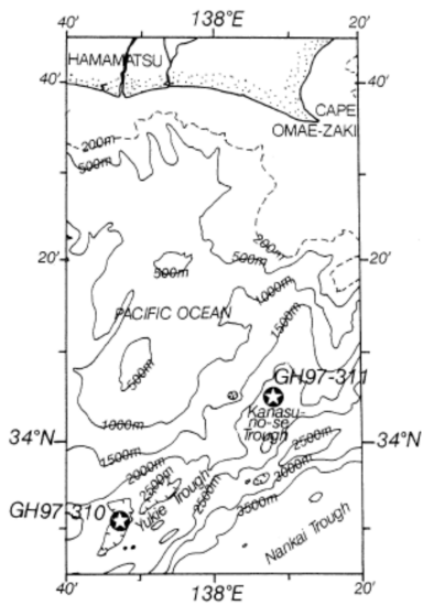
1 2 図 3-25 南海トラフ沿いにおけるタービダイトの採取地点（左）と研究対象試料の柱状図 3 及び浮遊性有孔虫を用いた放射性炭素年代値（ \delta^{13}\text{C} 補正年代）（池原，2001） 4 柱状図でハッチをつけた部分がタービダイト、白抜き部は通常時に堆積した半遠洋性泥。
