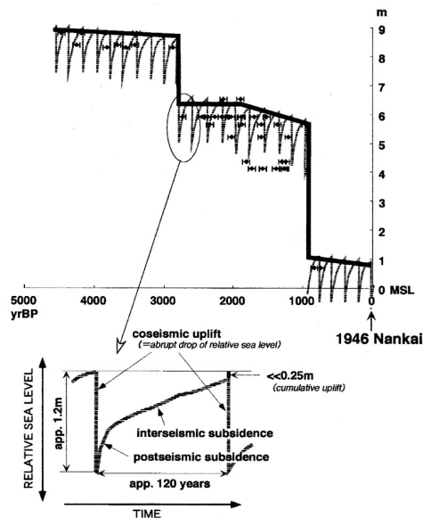
図 3-24 室戸半島における完新世地震性地殻変動 (前空, 2001)
