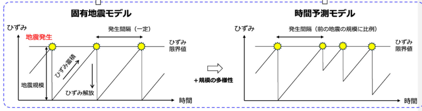
図 4-7 地震発生モデルの物理的背景
