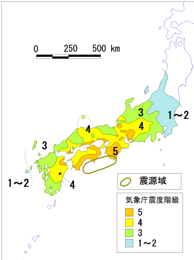
1 2 図3-9 1946年昭和南海地震の震度分布図（気象庁, 1968より作成） 3 図3-8及び図3-9は限られた震度観測結果を参照して等震度線を引いたもの。下図では、局 4 地的な震度分布も可能な範囲で表現した。なお、震度5弱及び5強は震度5と表現し、震 5 度6弱以上は震度6以上と表現した。また、当時の震度階級で表現しており、震度6は現 6 在の震度6弱以上に相当する。
