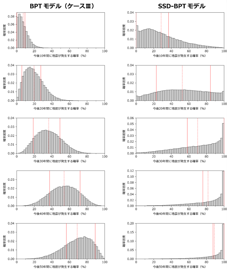
図 4-8 BPT モデルと SSD-BPT モデルによる発生確率の事後分布の比較 評価時点（2025 年 1 月 1 日）から今後 10、20、30、40、50 年間に地震が発生する確率の頻度分布。左側が BPT モデル（ケースⅢ）、右側が SSD-BPT モデルによる確率を表す。各分布において、赤色の実線は 70%信用区間、赤色の破線は期待値（平均値）を示す。
