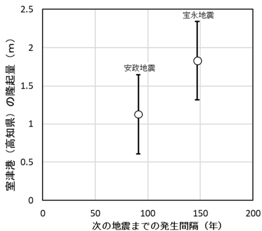
図5 室津港（高知県）における南海地震時の隆起量と次の地震までの期間との関係
