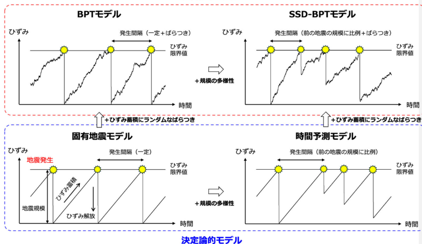
図 4-7 地震発生モデルの物理的背景
