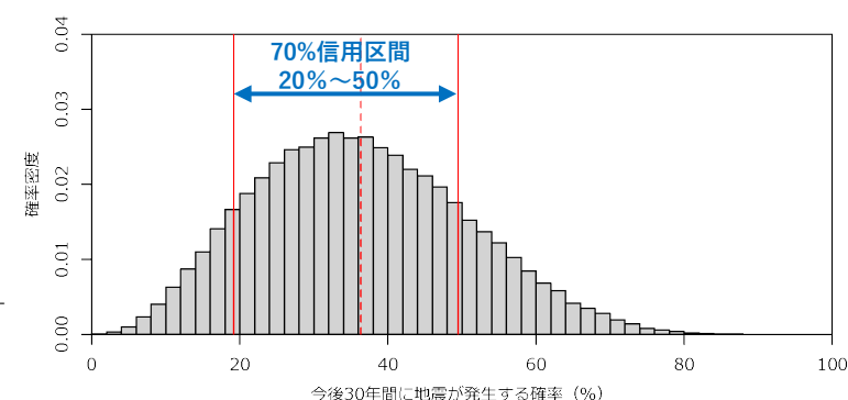
②'ベイズBPTモデルに基づく今後30年後の南海トラフ地震発生確率の確率分布（ケースⅢ）
