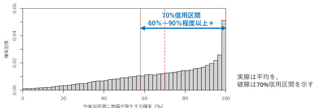
①'ベイズSSD-BPTモデルに基づく今後30年後の南海トラフ地震発生確率の確率分布
