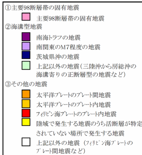
図3 今後30年以内に震度6弱以上の揺れをもたらす可能性のある地震の影響度
