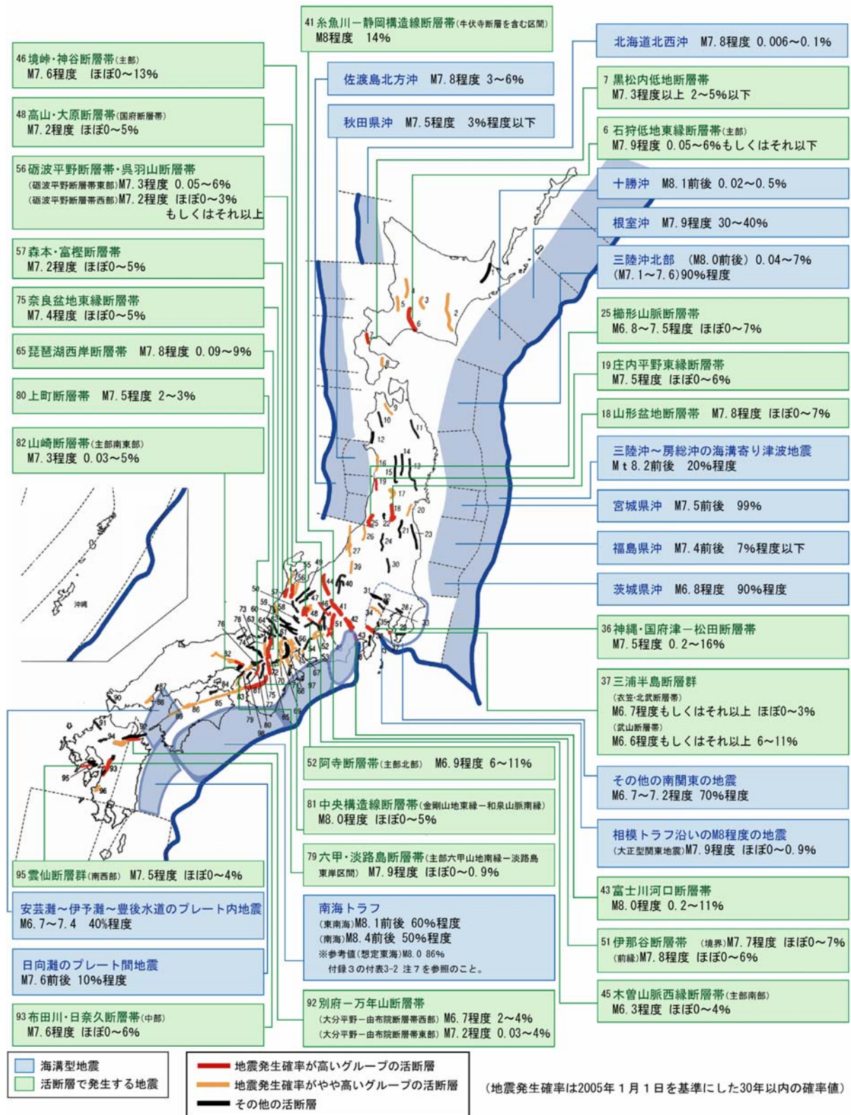
図1 主要98断層帯の位置及びおよび海溝型地震の発生領域と主な長期評価結果
