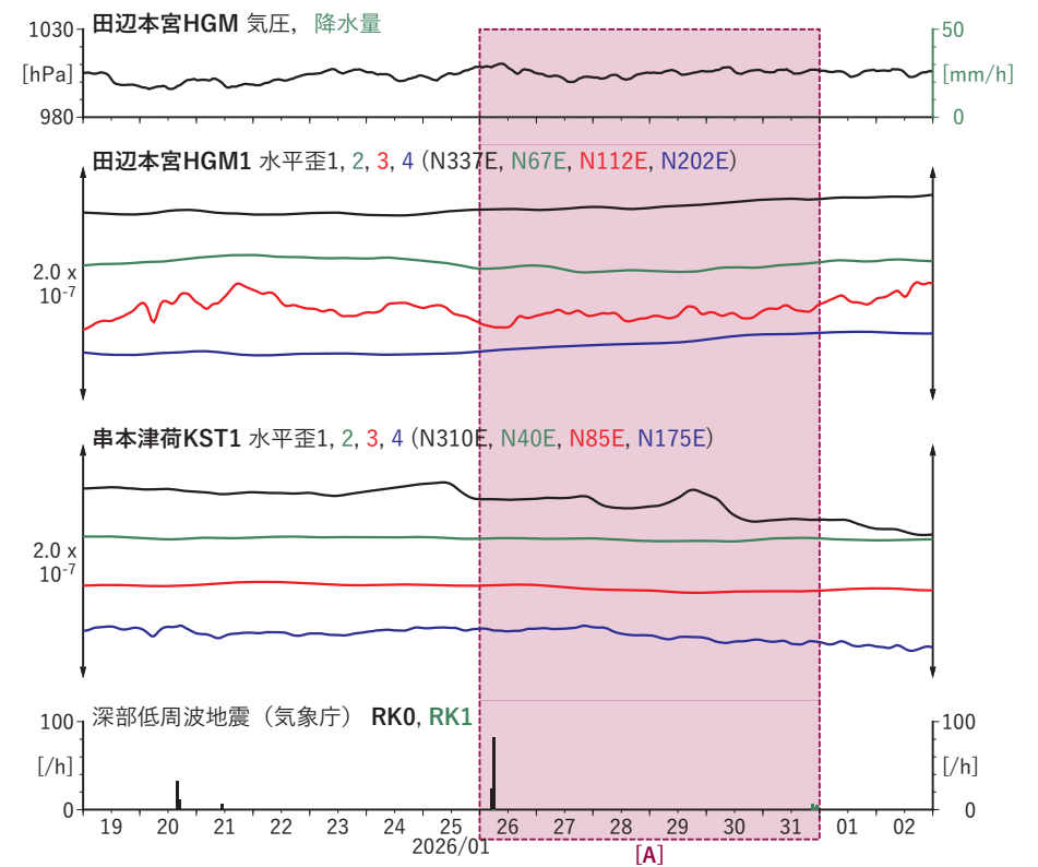
図2 歪の時間変化（2026/01/19 00:00–2026/02/03 00:00 (JST)）
