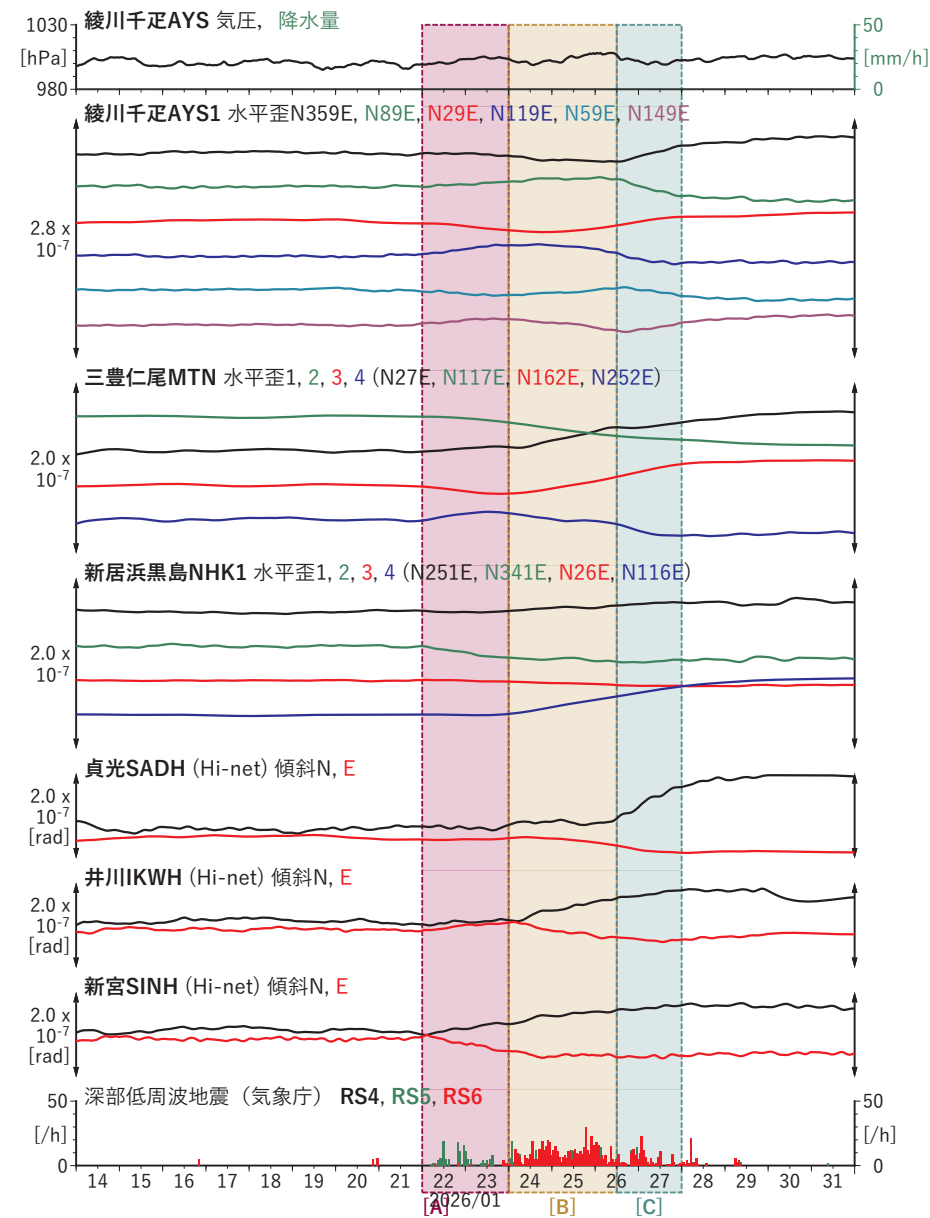
図9 歪・傾斜の時間変化（2026/01/14 00:00-2026/02/01 00:00 (JST)）
