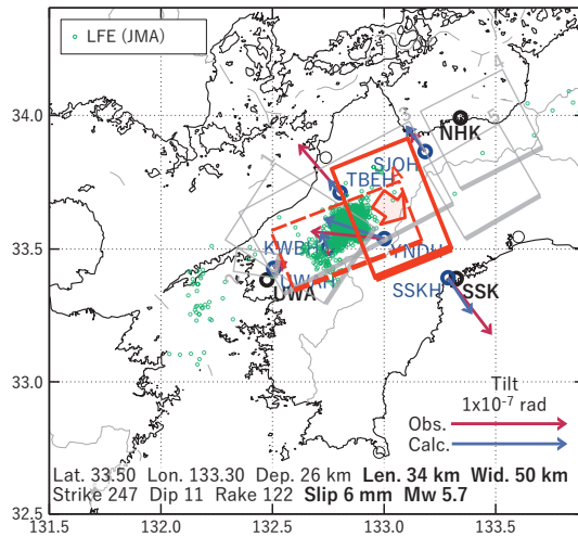
図11 2025/12/07-12の歪・傾斜変化 (図9[B]) を説明する断層モデル。
