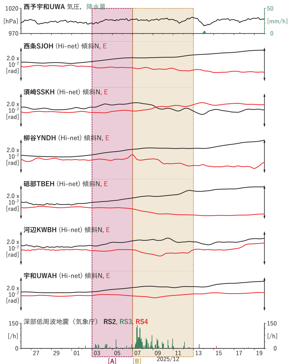
図9 歪・傾斜の時間変化(2) (2025/11/26 00:00-2025/12/20 00:00 (JST))
