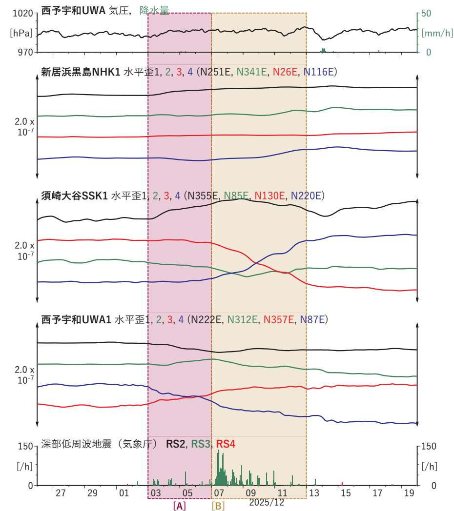
図9 歪・傾斜の時間変化(1) (2025/11/26 00:00–2025/12/20 00:00 (JST))
