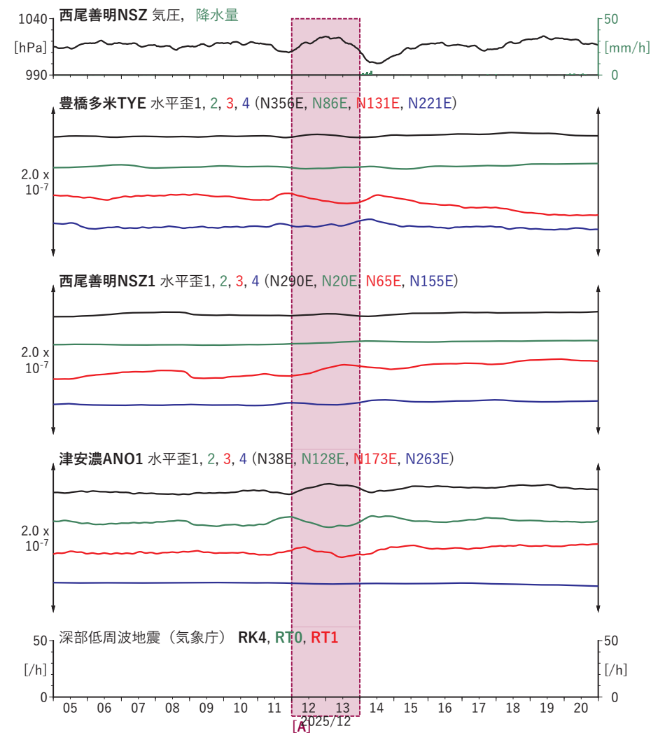
図6 歪の時間変化(1) (2025/12/05 00:00–2025/12/21 00:00 (JST))
