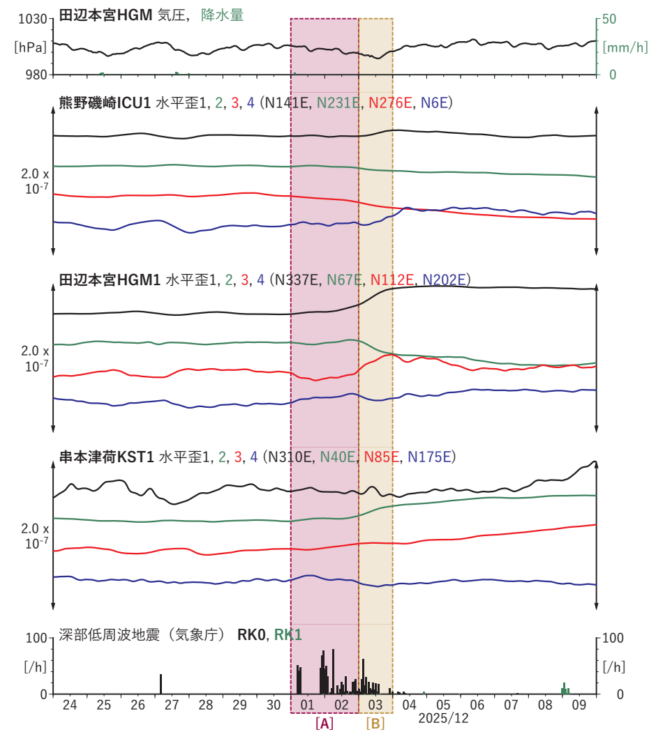
図2 歪の時間変化（2025/11/24 00:00–2025/12/10 00:00 (JST)）
