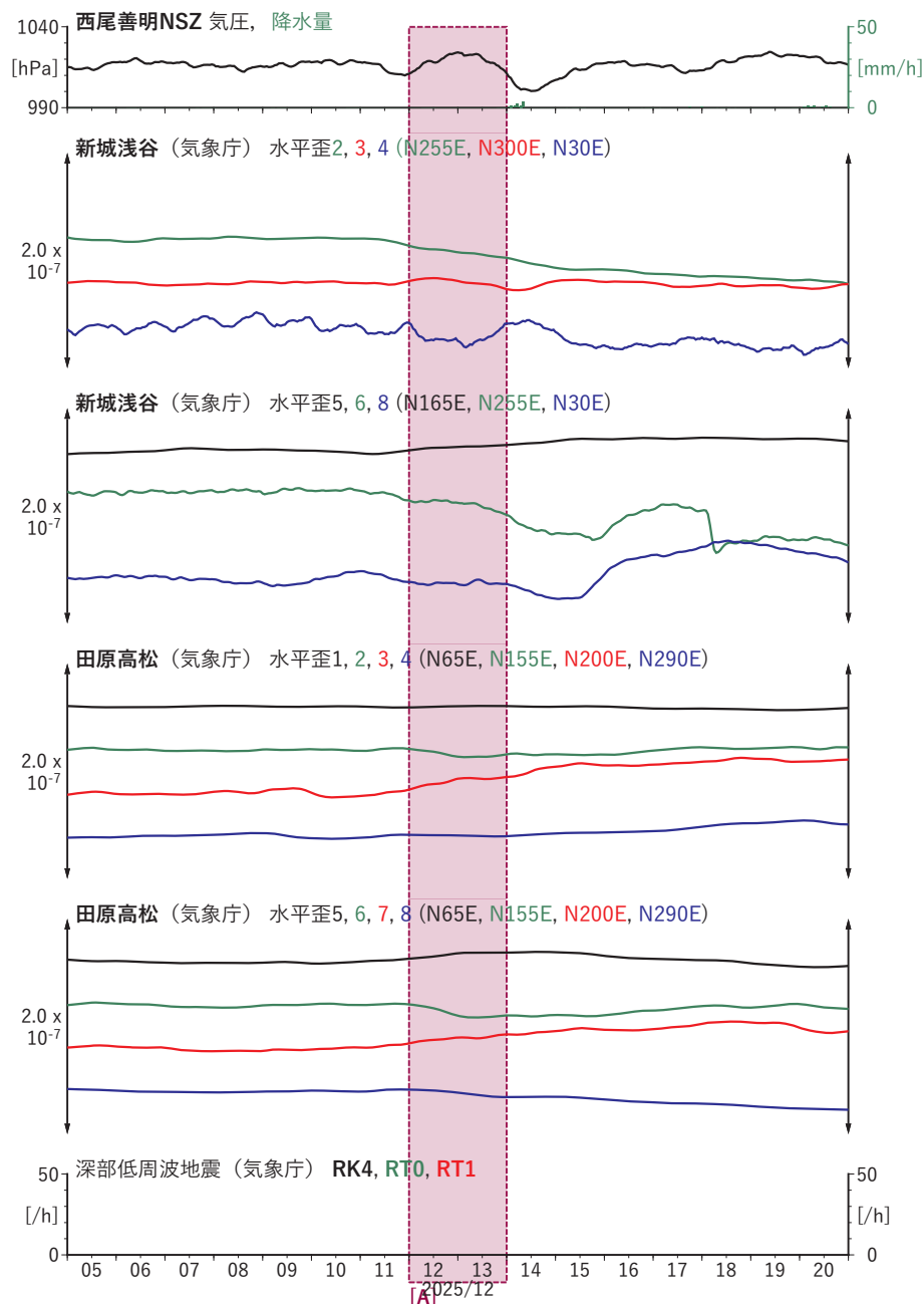
図6 歪の時間変化(2) (2025/12/05 00:00-2025/12/21 00:00 (JST))
