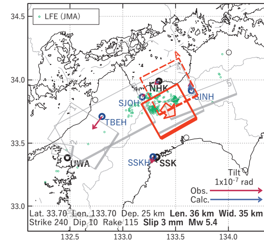
図10 2025/11/22-26の歪・傾斜変化 (図8[B]) を説明する断層モデル。
