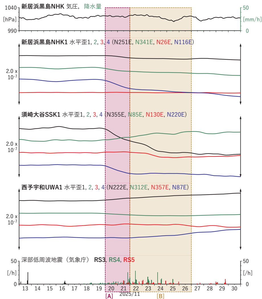
図8 歪・傾斜の時間変化(1) (2025/11/13 00:00-2025/12/01 00:00 (JST))
