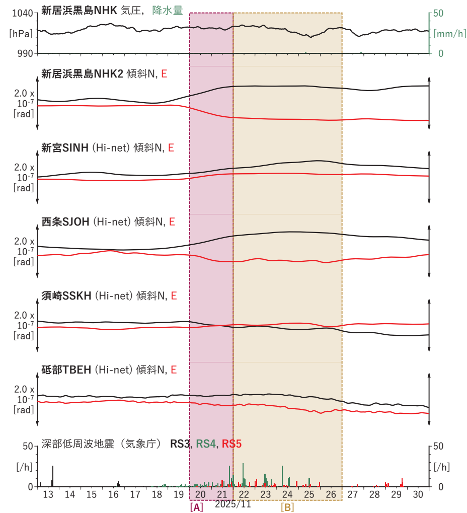
図8 歪・傾斜の時間変化(2) (2025/11/13 00:00-2025/12/01 00:00 (JST))
