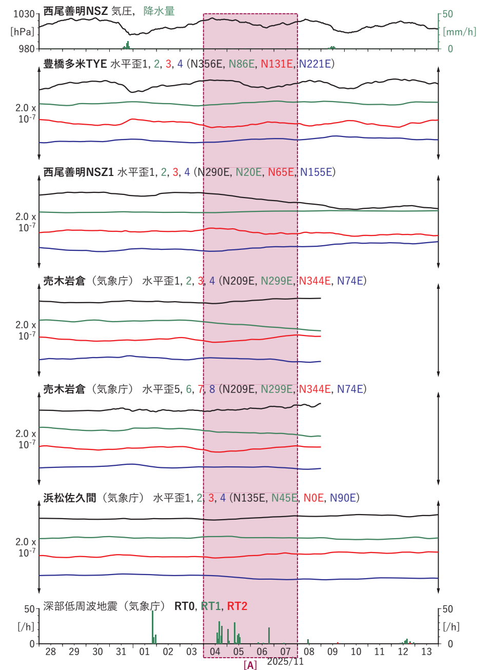
図2 歪・傾斜の時間変化(1) (2025/10/28 00:00–2025/11/14 00:00 (JST))
