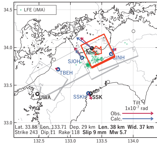
図9 2025/11/20-21の歪・傾斜変化 (図8[A]) を説明する断層モデル。
