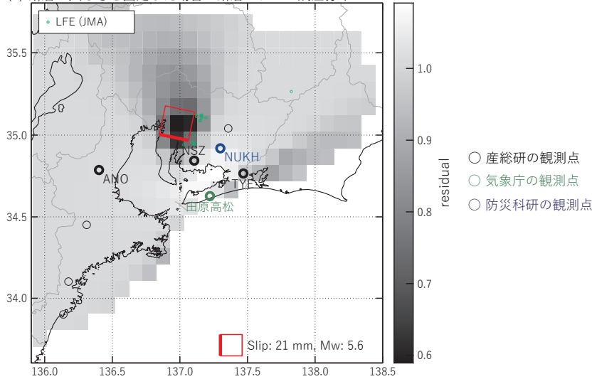
(b1) 推定した断層モデル
