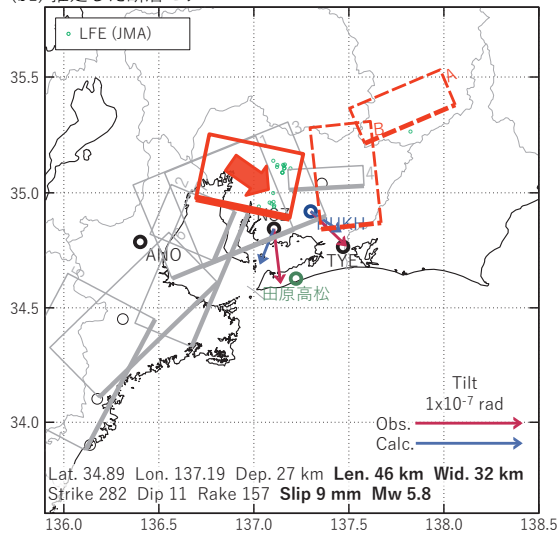
図5 2025/07/12PM-15AMの歪・傾斜変化 (図2[C]) を説明する断層モデル。
