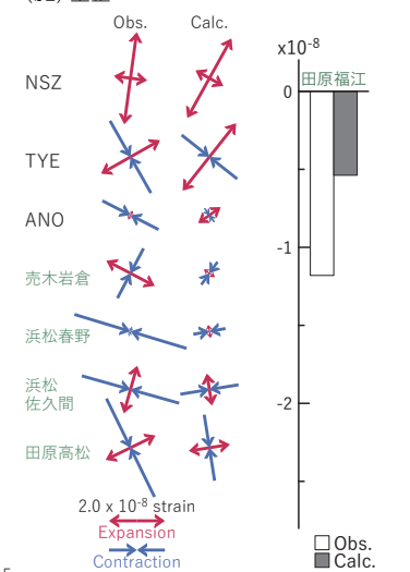
図6 2025/07/15PM-18の歪・傾斜変化 (図2[D]) を説明する断層モデル。
