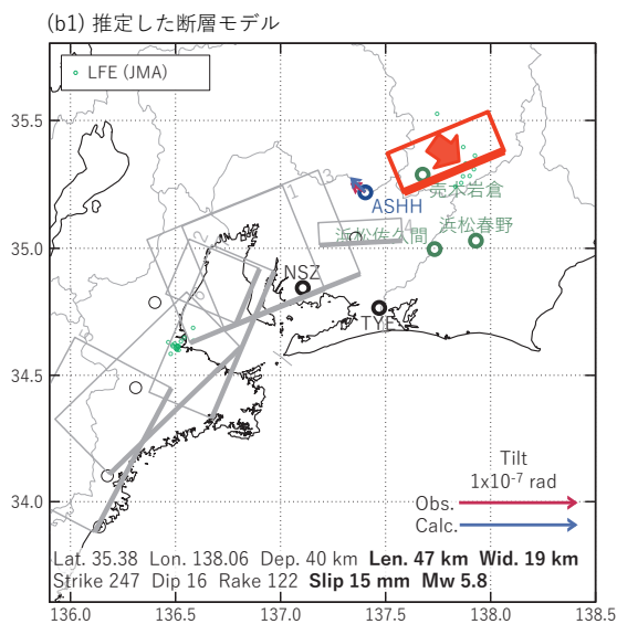
図3 2025/07/04PM-06の歪・傾斜変化（図2[A]）を説明する断層モデル。
