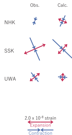
図11 2025/06/16-20の歪・傾斜変化 (図8[C]) を説明する断層モデル。
