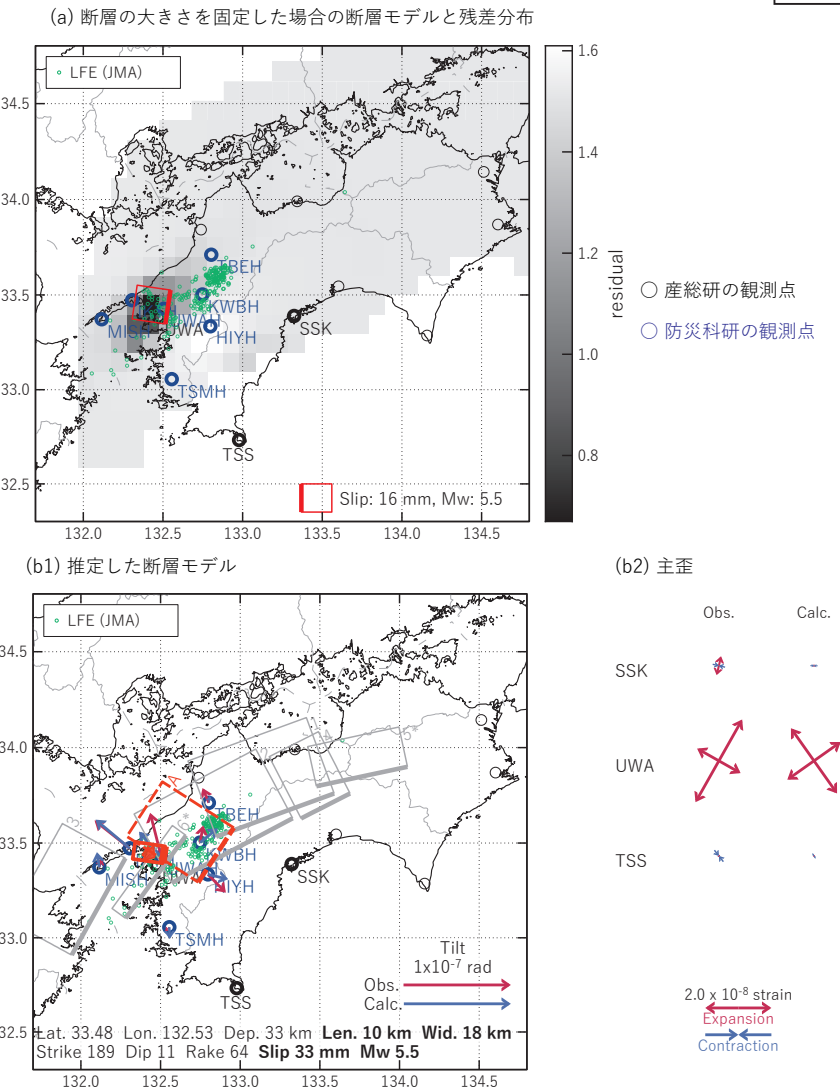
図10 2025/06/15の歪・傾斜変化（図8[B]）を説明する断層モデル。
