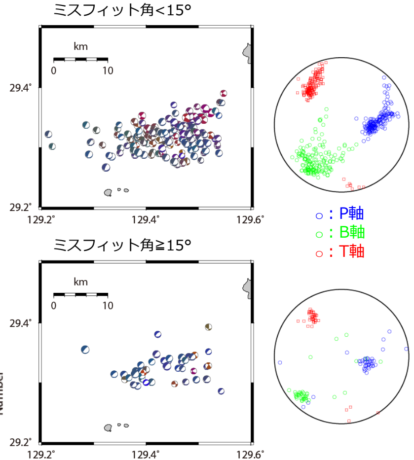
図5 ミスフィット角が15°未満と15°以上のメカニズム解の比較。ビーチボールの色は図2参照。ミスフィット角の大きい地震は類似した正断層型が多い。
