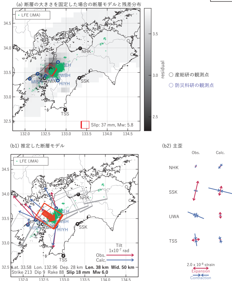
図9 2025/06/10-14の歪・傾斜変化（図8[A]）を説明する断層モデル。
