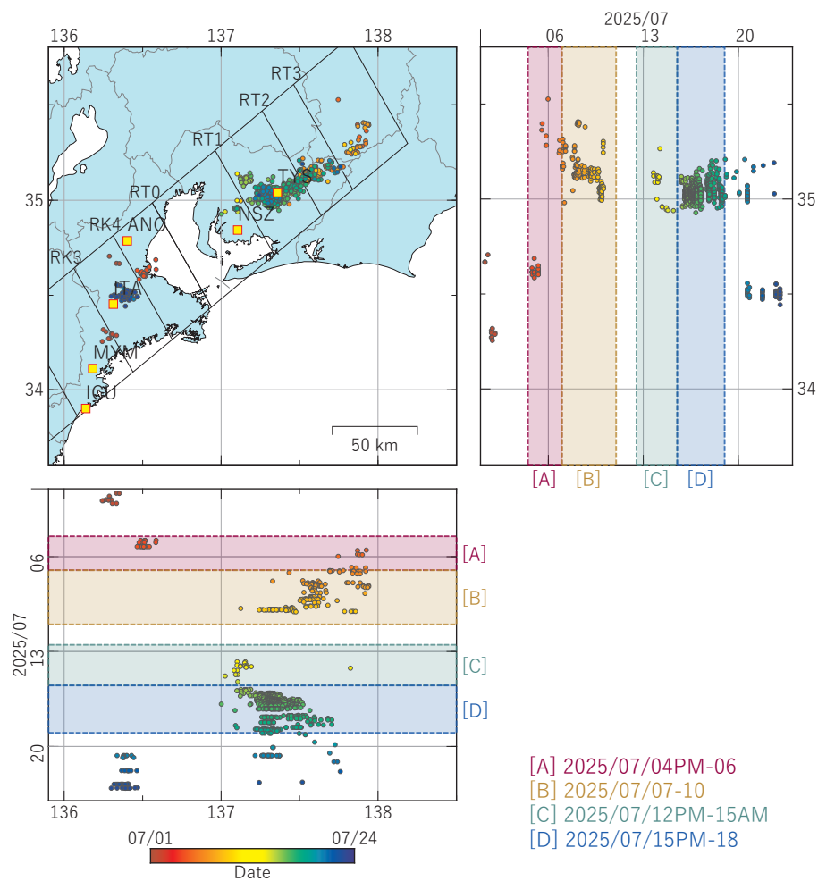
図1 東海・紀伊半島における低周波地震の時空間分布図 (2025/07/01 00:00 - 2025/07/24 00:00 (JST))。気象庁カタログによる。 (観測点名) TYS: 豊田神殿, NSZ: 西尾善明, ANO: 津安濃, ITA: 松阪飯高, MYM: 紀北海山, ICU: 熊野磯崎
