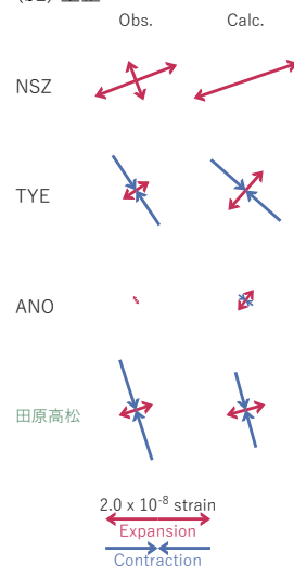
図5 2025/07/12PM-15AMの歪・傾斜変化 (図2[C]) を説明する断層モデル。
