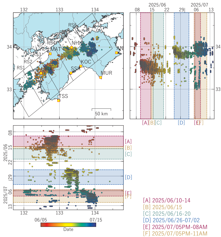
図7 四国地方における低周波地震の時空間分布図 (2025/06/05 00:00 - 2025/07/15 00:00 (JST))。気象庁カタログによる。 (観測点名) ANK: 阿南桑野, MUR: 室戸岬, NHK: 新居浜黒島, KOC: 高知五台山, SSK: 須崎大谷, MAT: 松山南江戸, UWA: 西予宇和, TSS: 土佐清水松尾
