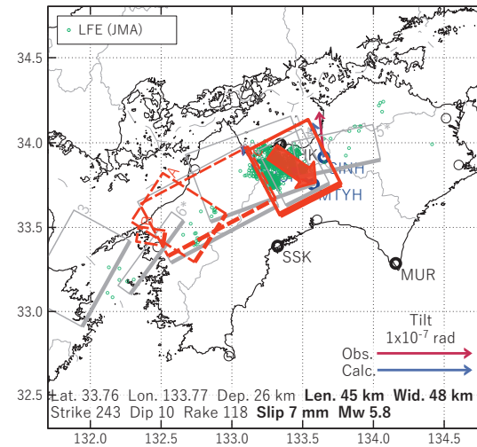
図12 2025/06/26-07/02の歪・傾斜変化 (図8[D]) を説明する断層モデル。
