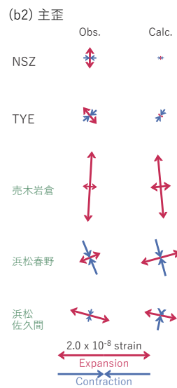
図3 2025/07/04PM-06の歪・傾斜変化（図2[A]）を説明する断層モデル。
