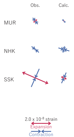
図12 2025/06/26-07/02の歪・傾斜変化 (図8[D]) を説明する断層モデル。
