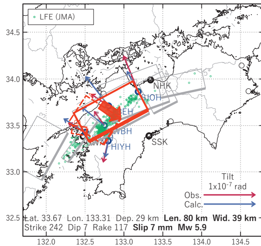
図11 2025/06/16-20の歪・傾斜変化 (図8[C]) を説明する断層モデル。
