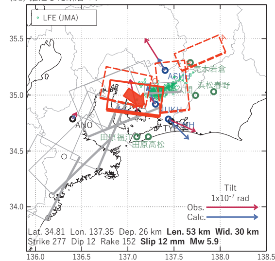
図6 2025/07/15PM-18の歪・傾斜変化 (図2[D]) を説明する断層モデル。
