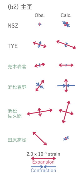
図4 2025/07/07-10の歪・傾斜変化（図2[B]）を説明する断層モデル。
