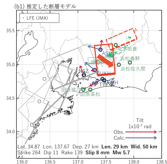
図4 2025/07/07-10の歪・傾斜変化（図2[B]）を説明する断層モデル。
