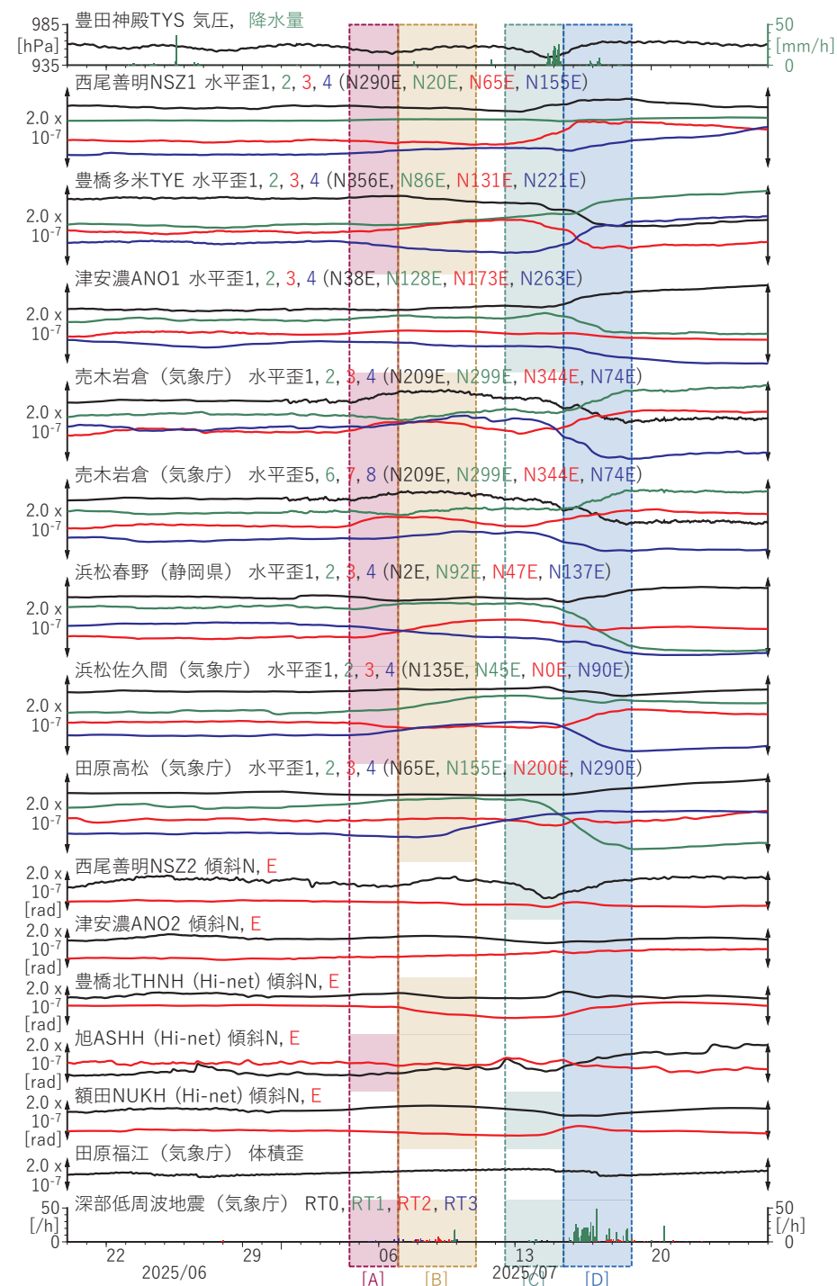
図2 東海・紀伊半島における歪・傾斜観測結果 (2025/06/20 00:00 - 2025/07/26 00:00 (JST))
