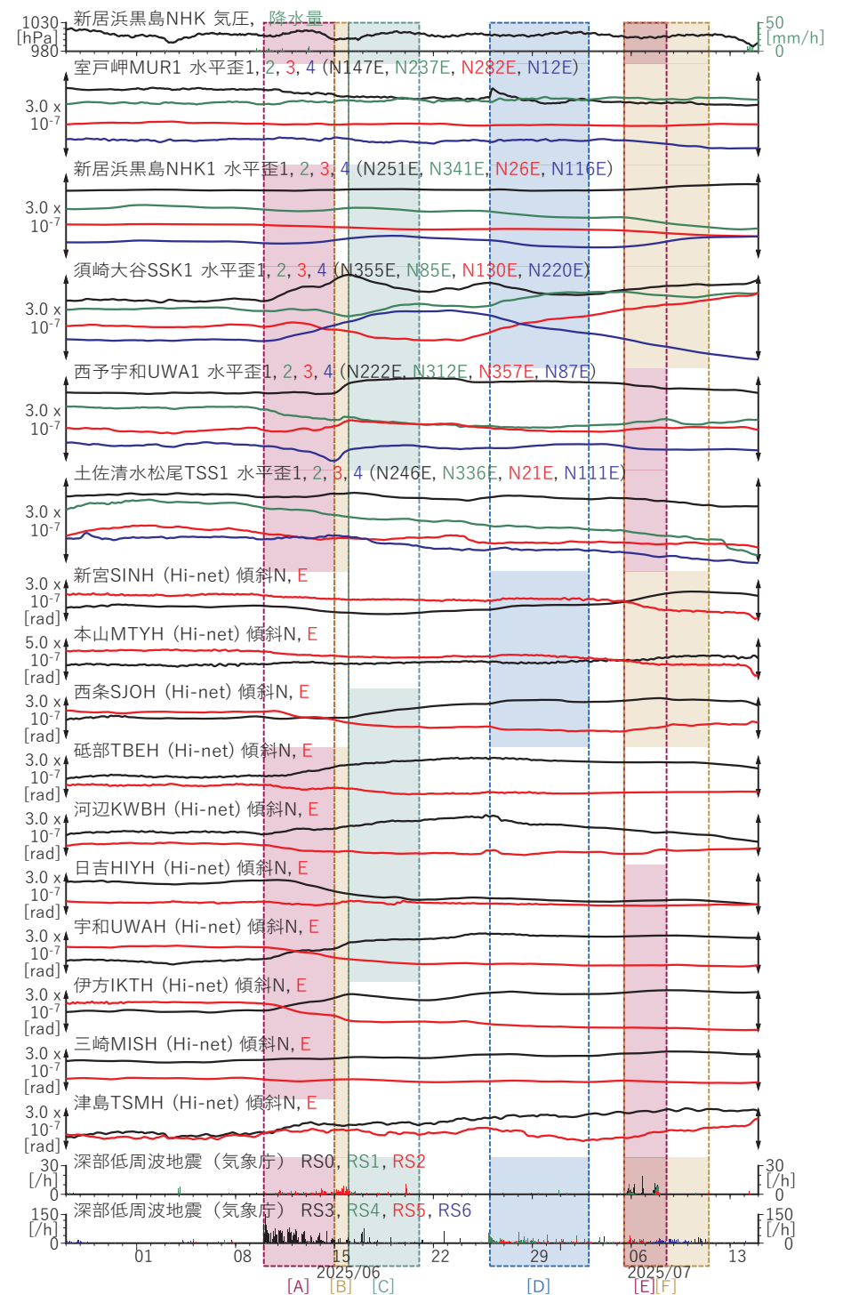
図8 四国地方における歪・傾斜観測結果 (2025/05/27 00:00 - 2025/07/15 00:00 (JST))
