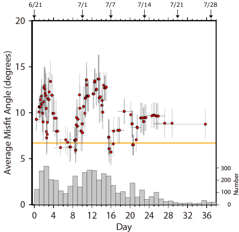
図4 ミスフィット角の平均値の時間変化（10イベントの移動平均）。横軸は6月21日からの経過日数。オレンジの線は、基準応力場の推定時に実施した応力テンソルインバージョンにおけるミスフィット角の平均値。灰色のバーは、気象庁一元化震源に基づく1日ごとの地震個数（M1以上）。
