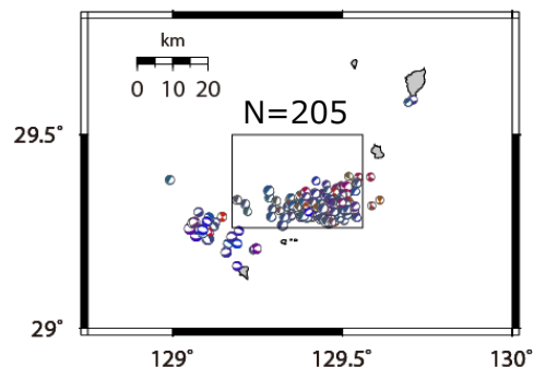
図3 ミスフィット角の計算に使った地震（2025/6/21～7/28、深さ20 km以浅のF-net解）
