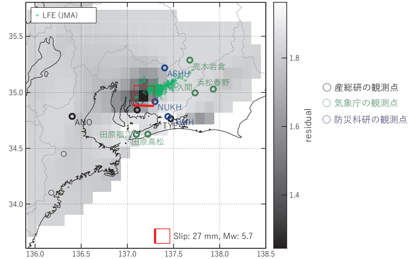
(b1) 推定した断層モデル
