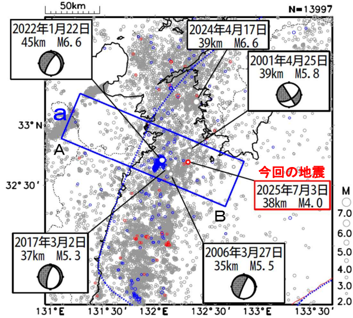
震央分布図 (1997年10月1日～2025年7月3日、深さ0～90km、 M \geq 2.0 ) 2024年1月22日から2022年6月30日までの地震を青色、 2025年6月以降の地震を赤色で表示 図中の発震機構はCMT解
