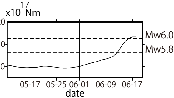
モーメント時系列図
