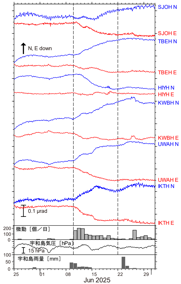
図1：2025年5月25日～7月1日の傾斜時系列。上方向への変化が北・東下がりの傾斜変動を表し、BAYTAP-Gにより潮汐・気圧応答成分を除去した。6月10日～21日の傾斜変化ベクトルを図2に示す。四国西部での微動活動度・気象庁宇和島観測点の気圧・雨量を合わせて示す。
