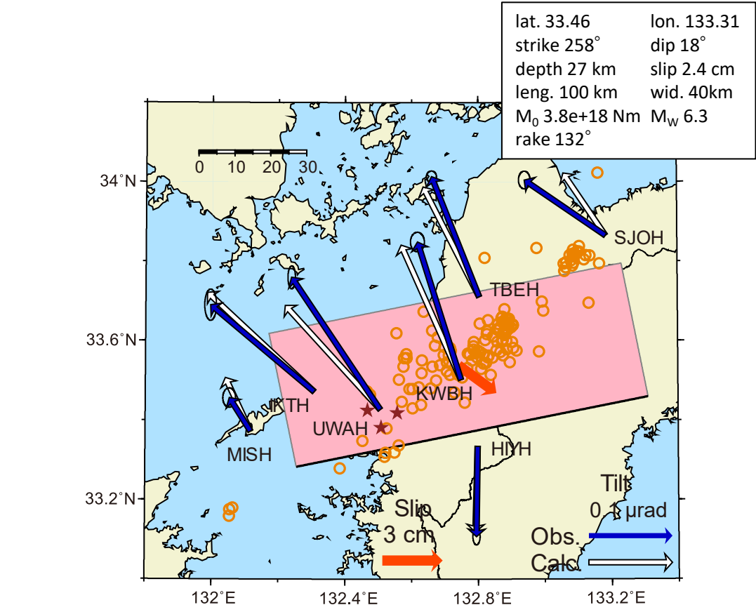
図2：6月10日～21日に観測された傾斜変化ベクトル（青矢印）、推定されたスロースリップイベントの断層モデル（赤矩形・矢印）、モデルから計算される傾斜変化ベクトル（白抜き矢印）を示す。1時間毎の微動エネルギーの重心位置（橙丸）、深部超低周波地震（茶星印）も合わせて示す。すべり角はプレート相対運動方向に固定している。
