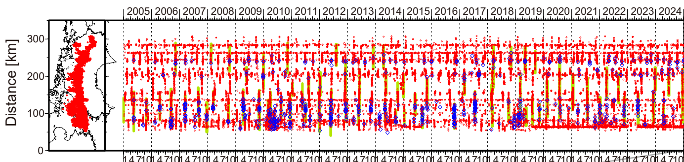
図 1. 四国における 2005 年 1 月 ~ 2025 年 1 月 7 日までの深部低周波微動の時空間分布 (上図). 赤丸はエンベロープ相関・振幅ハイブリッド法 (Maeda and Obara, 2009) およびクラスタ処理 (Obara et al., 2010) によって 1 時間毎に自動処理された微動分布の重心である. 青菱形は
