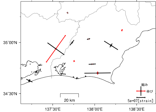
基準日: 2023/12/02 比較日: 2024/03/01
