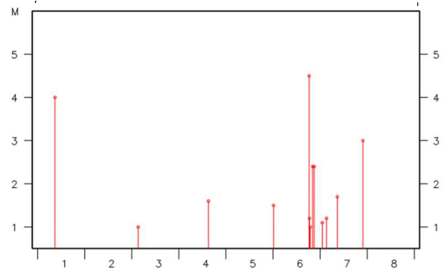
領域 b 内の M-T 図 (2025 年 1 月 1 日～8 日、 M \geq 1.0 )
