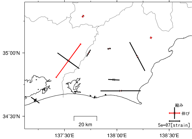
基準日: 2024/03/03 比較日: 2024/06/01
