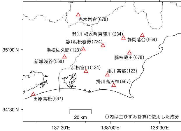
基準日: 2023/09/02 比較日: 2023/12/01
