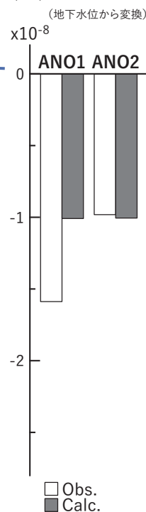
図3 2024/12/11-13AMの歪・傾斜・地下水位の変化(図2[A])を説明する断層モデル。
