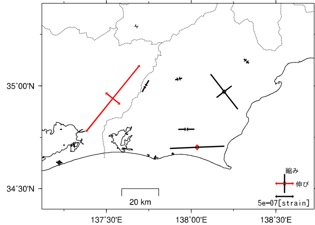
基準日: 2024/10/02 比較日: 2024/12/31
