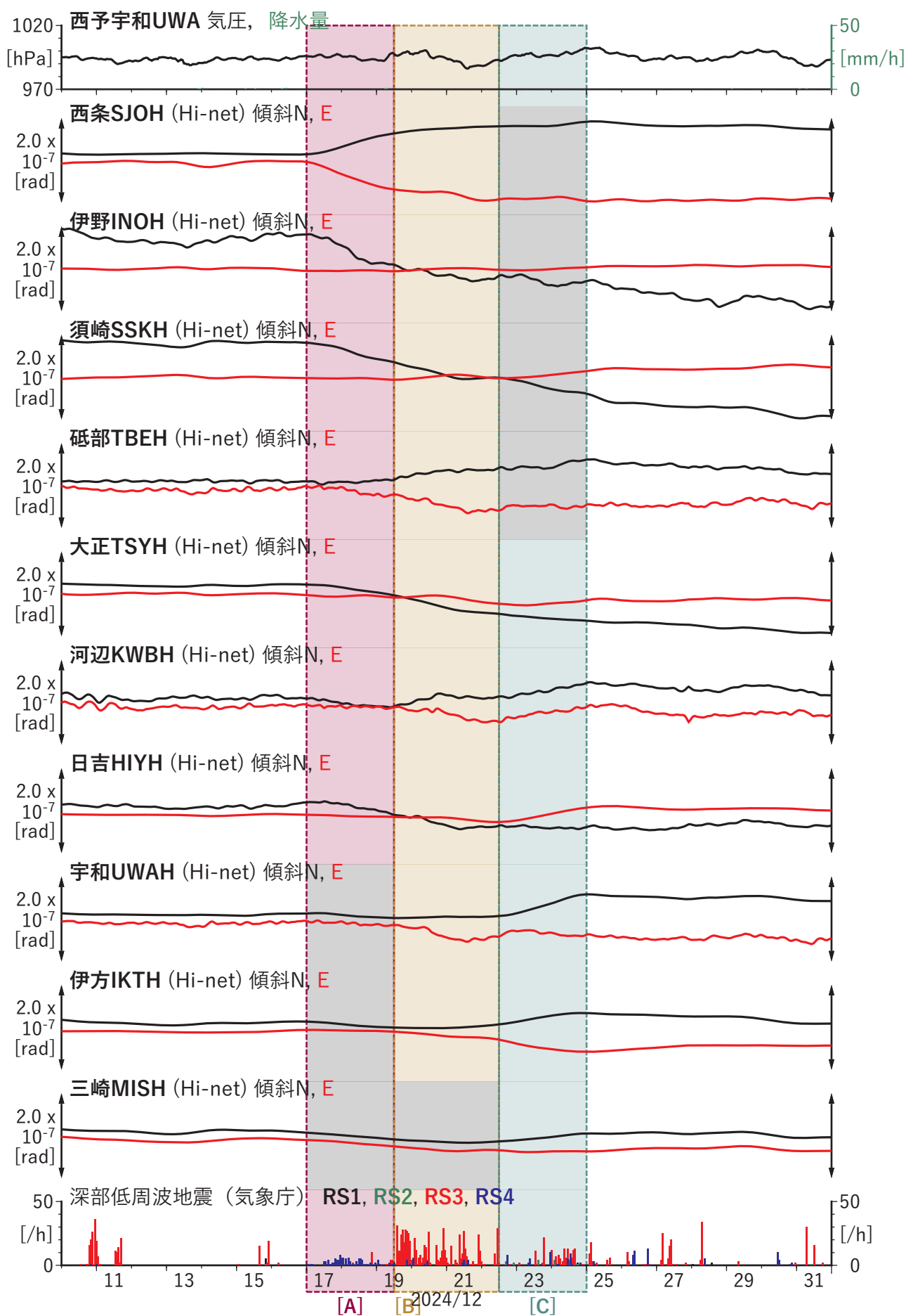
図6 歪・傾斜の時間変化(2) (2024/12/10 00:00-2025/01/01 00:00 (JST))
