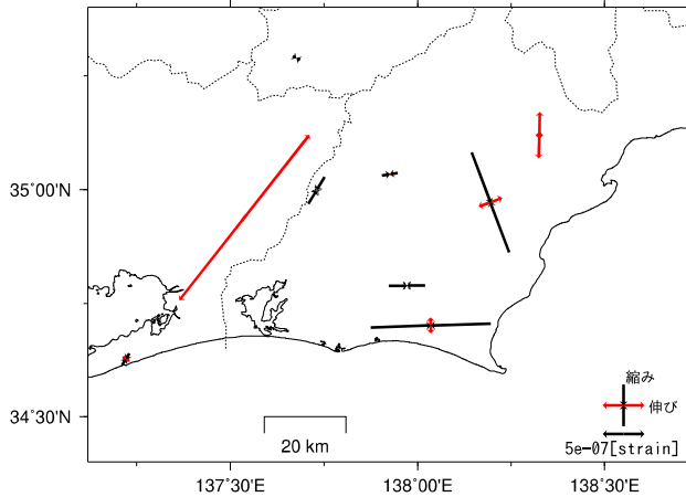
基準日: 2024/09/02 比較日: 2024/12/01
