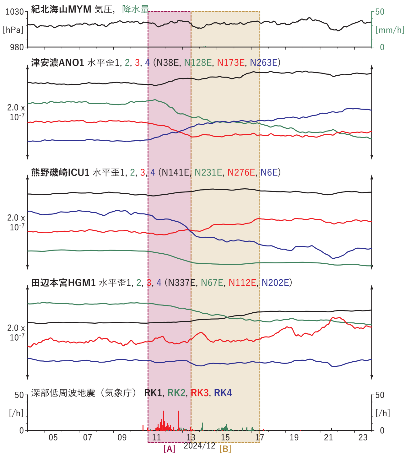
図2 歪・傾斜・地下水位の時間変化(1) (2024/12/04 00:00-2024/12/24 00:00 (JST))
