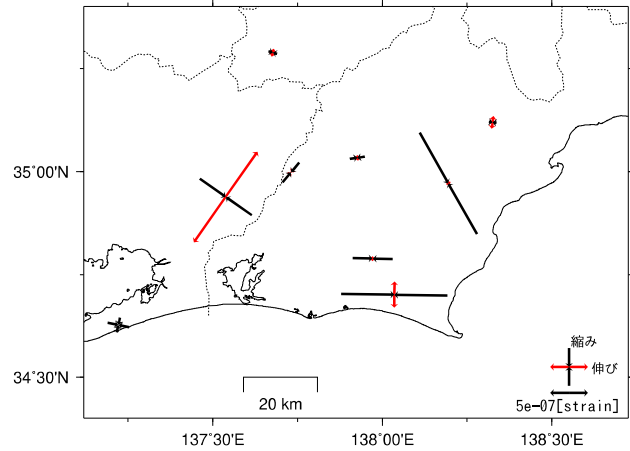
基準日: 2024/06/03 比較日: 2024/09/01
