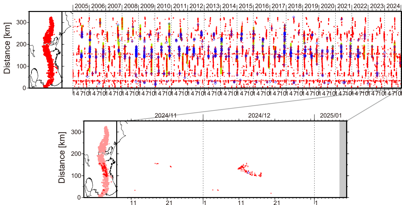
図 1. 紀伊半島・東海地域における 2005 年 1 月～2025 年 1 月 7 日までの深部低周波微動の時空間分布 (上図). 赤丸はエンベロープ相関・振幅ハイブリッド法 (Maeda and Obara, 2009) およびクラスタ処理 (Obara et al., 2010) によって 1 時間毎に自動処理された微動分布の重心である. 青菱形は周期 20 秒に卓越する超低周波地震 (Ito et al., 2007) である. 黄緑色の太線はこれまでに検出された短期的スロースリップイベント (SSE) を示す. 下図は 2024 年 12 月を中心とした期間の拡大図である. 12 月 10 ～ 17 日頃には三重県中部から三重・奈良県境付近において、活発な微動活動がみられた. この活動は三重・奈良県境付近から開始し、13 日頃まで北東・南西両方向への活動域の拡大がみられた. その後、南西方向への活動域の移動が 17 日頃までみられた.
