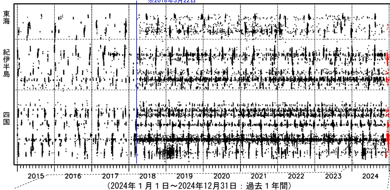
上図領域a内の時空間分布図（A-B投影）
