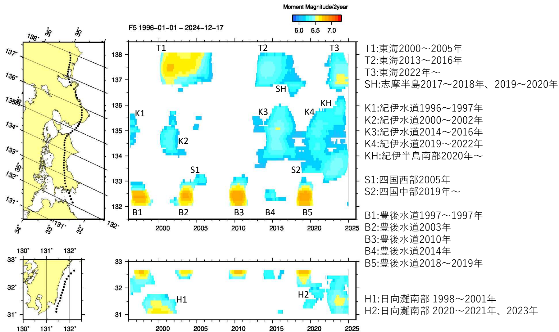
第2図 長期的スロースリップの規模分布（1996年～2024年12月） 2年間あたりの変化量から推定したモーメントマグニチュード。
