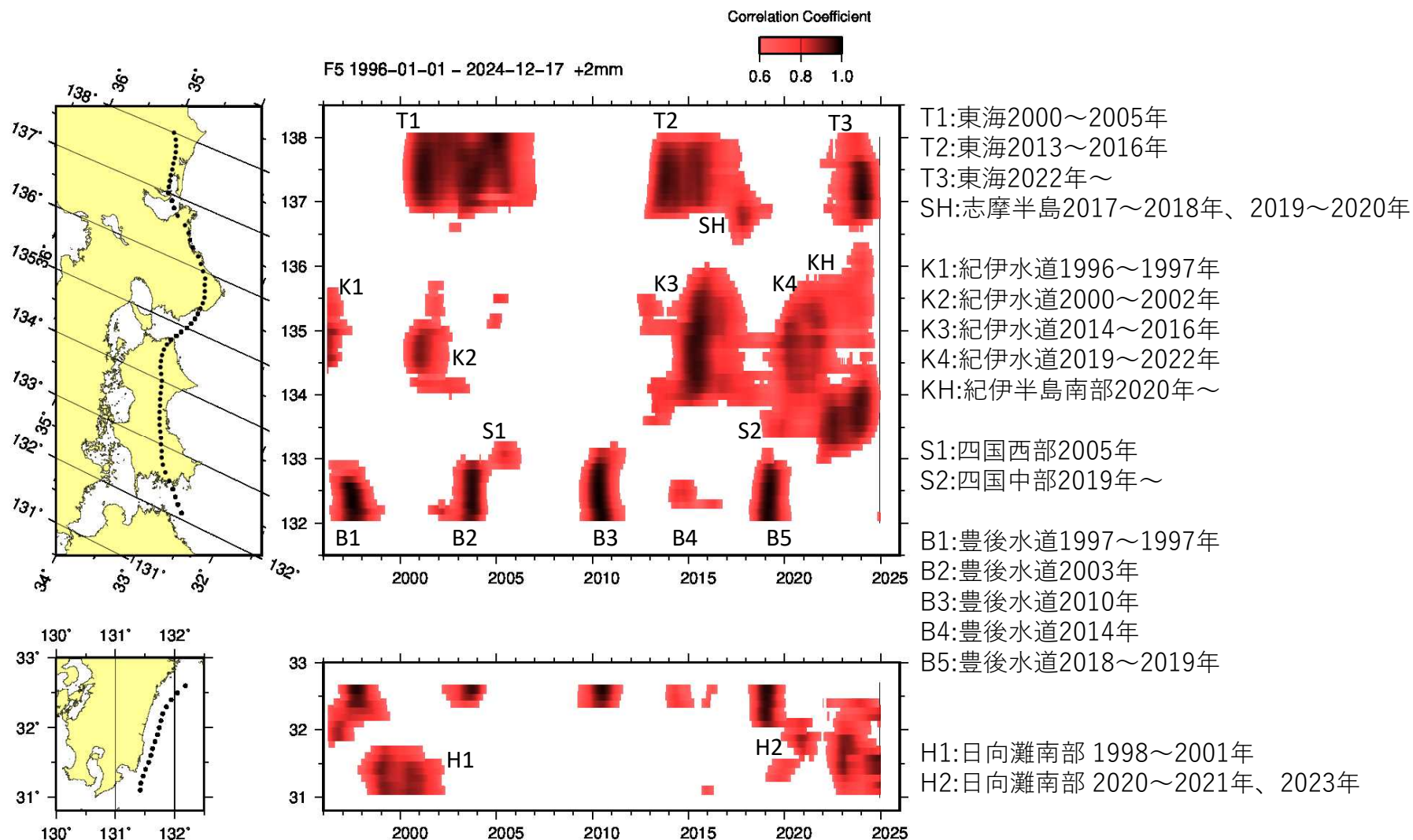
第1図 長期的スロースリップ客観検知図（1996年～2024年12月）
