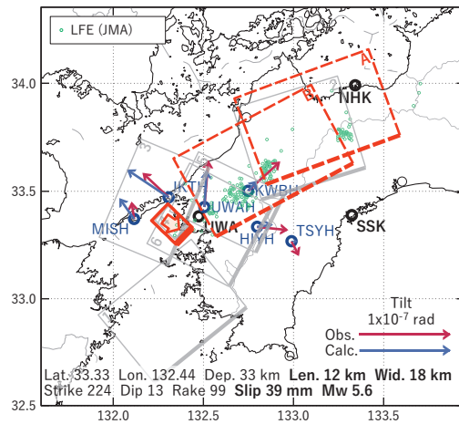
図9 2024/12/22PM-24の歪・傾斜変化（図6[C]）を説明する断層モデル。
