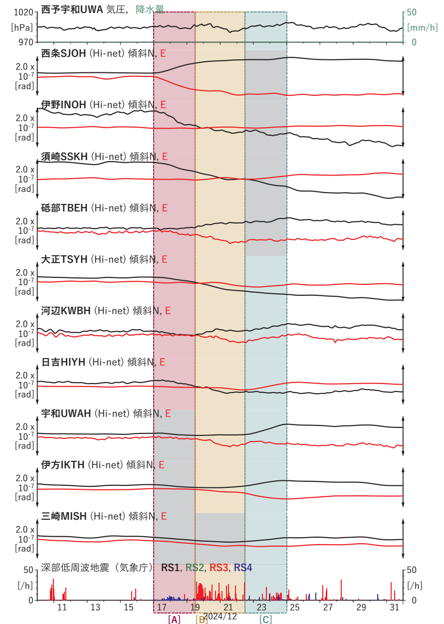
図6 歪・傾斜の時間変化(2) (2024/12/10 00:00-2025/01/01 00:00 (JST))
