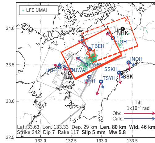
図8 2024/12/19PM-22AMの歪・傾斜変化（図6[B]）を説明する断層モデル。
