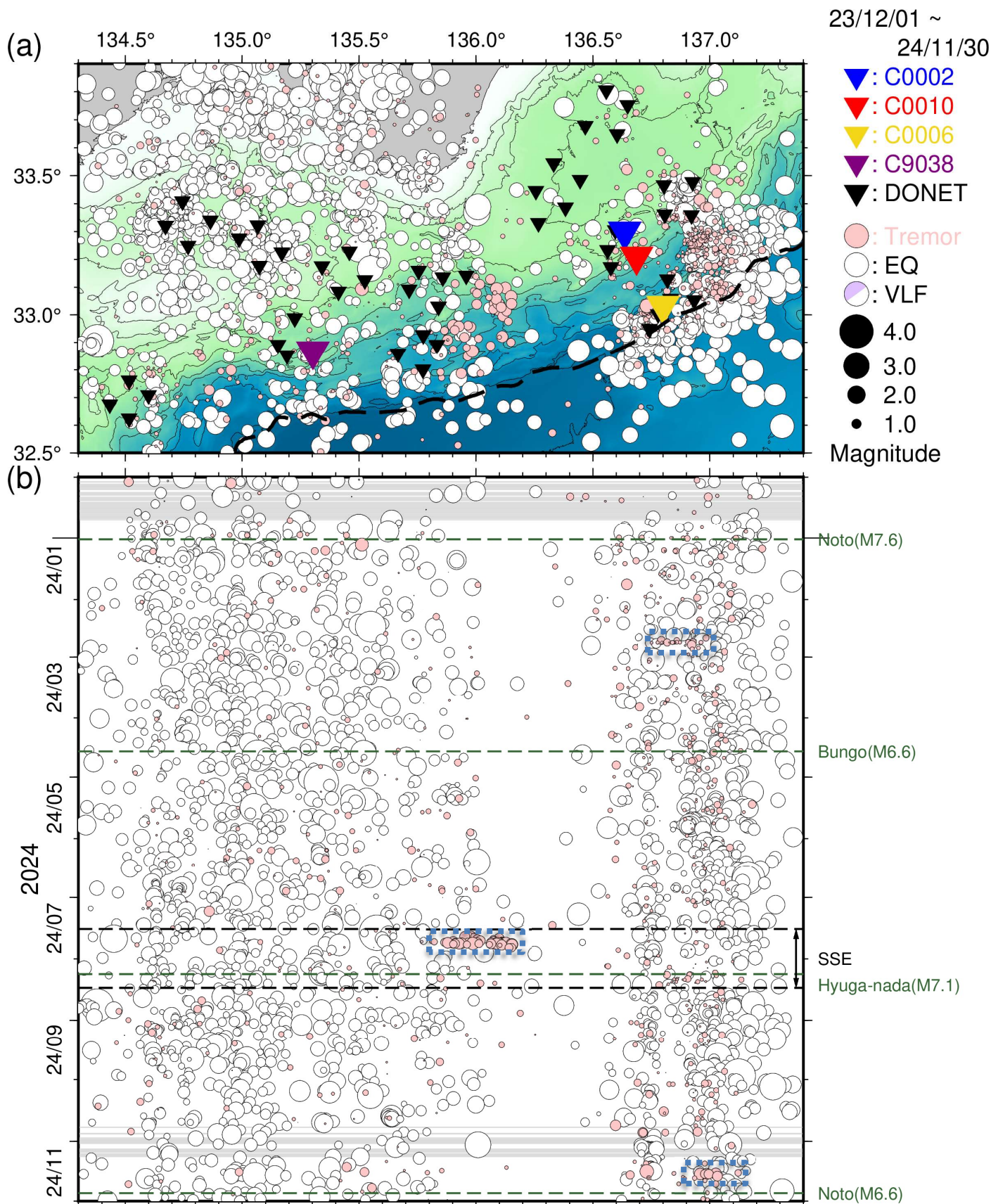
図 6 直近 1 年間に於いて熊野灘から室戸沖にて発生した低周波微動・通常地震・超低周波地震 (2023 年 12 月 1 日~2024 年 11 月 30 日)。図 4 と同様のシンボルにて表示。(a) 震央分布図。(b) a に示した震央を経度方向へ投影した時空間分布図。青点線の長方形領域は、これまでの評価文において言及した微動活動を示す。なお、過去資料の図 3 及び図 5 に緑点線で記した地震のうち、a の領域外かつ M6.5 未満のものは掲載していない。
