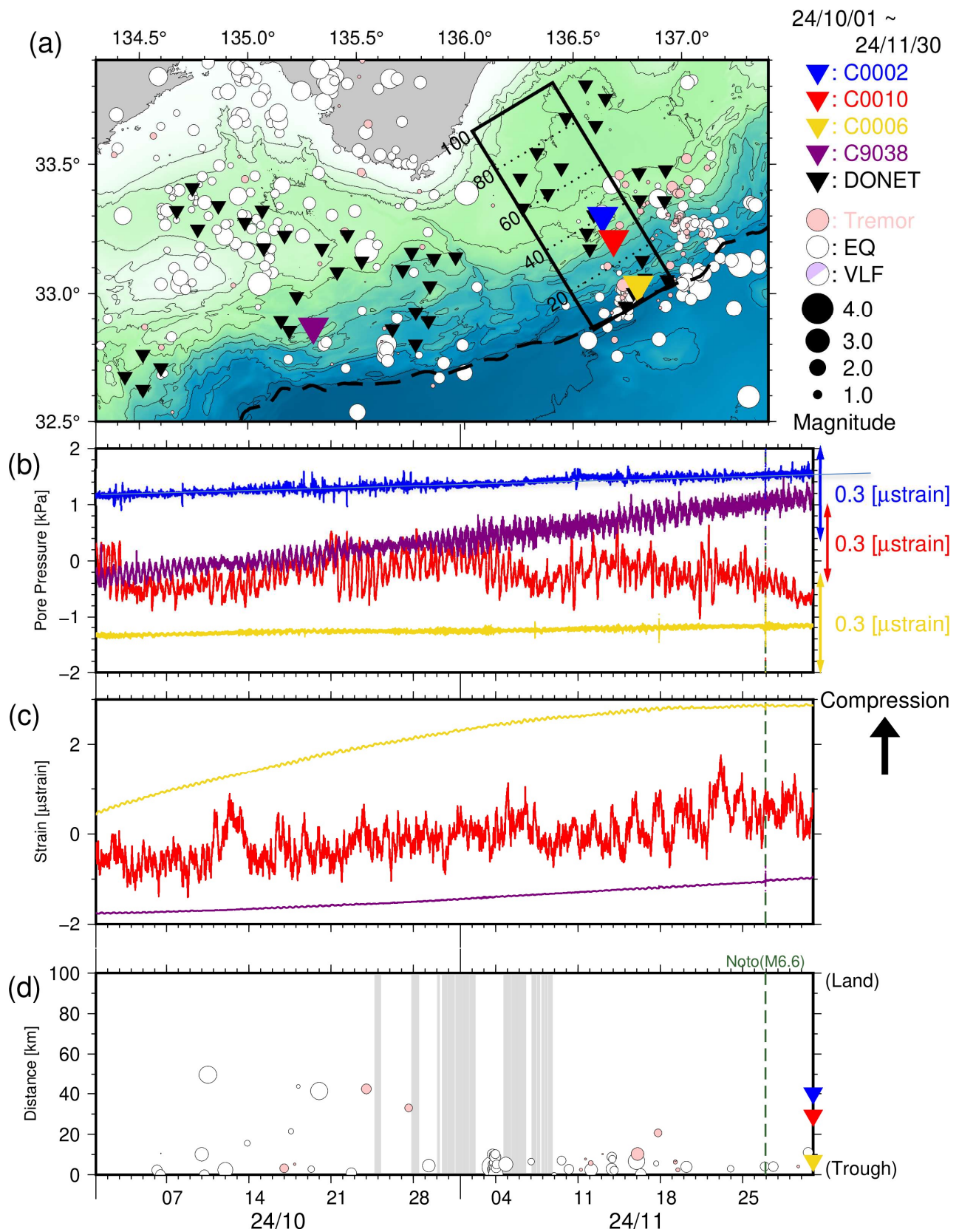
図3 直近2ヶ月間のSSE・低周波微動モニタリング(2024年10月1日~2024年11月30日)。 (a) 震央分布図(●:低周波微動(深さ0~15km)、○:通常地震(深さ0~60km)、●:超低周波地震のメカニズム解)。▼▼▼▼▼は、それぞれC0002・C0010・C0006・C9038・DONET観測点。破線はトラフ軸。(b) 長期孔内観測点における間隙水圧変化(—:C0002、—:C0010、—:C0006、—:C9038)。(c) 長期孔内観測点における体積歪計(—:C0010、—:C0006)および光ファイバ歪計(—:C9038)の変化。(d) 図3a中に実線で示した矩形領域内における、低周波微動・通常地震・超低周波地震の時空間分布。縦軸は、トラフ軸からの距離(km)。
