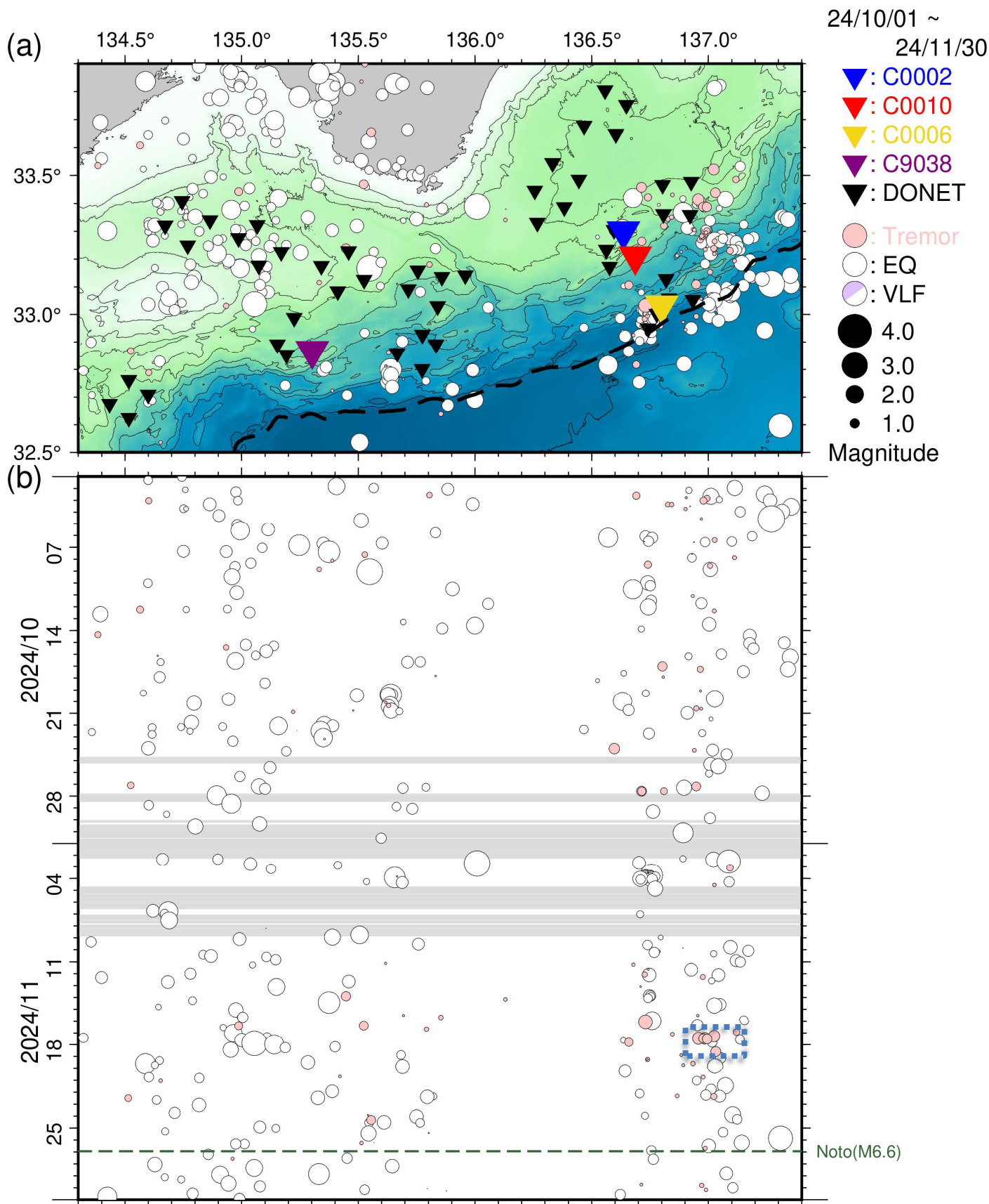
図5 直近2ヵ月間において熊野灘から室戸沖にて発生した低周波微動・通常地震・超低周波地震（2024年10月1日～2024年11月30日）。図3と同様のシンボルにて表示。(a) 震央分布図。(b) aに示した震央を経度方向へ投影した時空間分布図。青点線の長方形領域は、DONET1のBノードにおける低周波微動の群発的な活動を示す。
