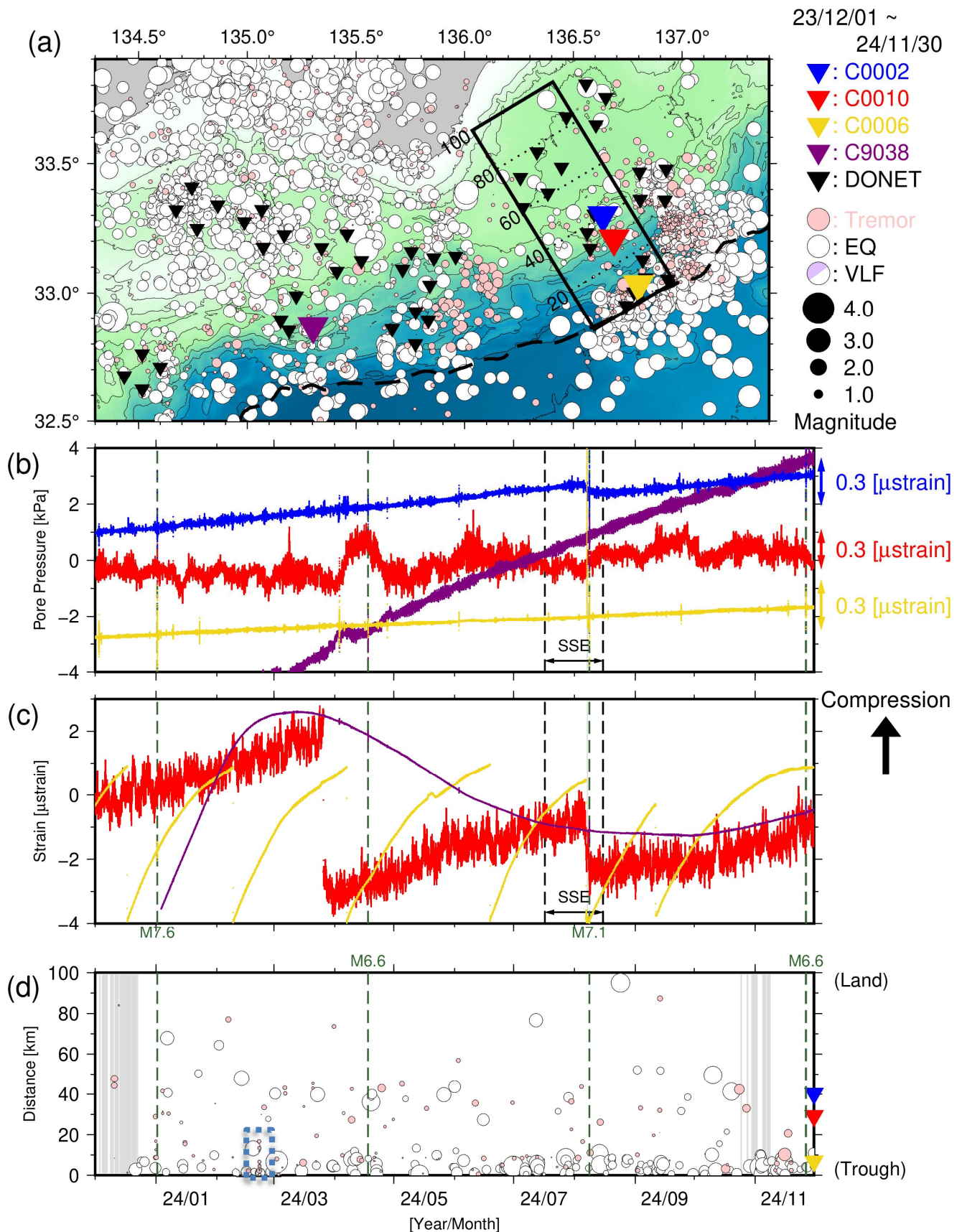
図4 直近1年間のSSE・低周波微動モニタリング(2023年12月1日~2024年11月30日)。(a) 低周波微動・通常地震・超低周波地震の震央分布。(b) 間隙水圧変化。(c) 体積歪変化。(d) 時空間分布。灰色はエアガン発振期間。緑点線は、能登地方の地震(1月1日M7.6、11月26日M6.6)、豊後水道の地震(4月17日M6.6)および日向灘の地震(8月8日M7.1)。青点線の長方形領域は、DONET1のCノード付近における低周波微動の群発的な活動を示す。なお、過去資料の図3に緑点線で記した地震のうち、aの領域外かつM6.5未満のものは掲載していない。
