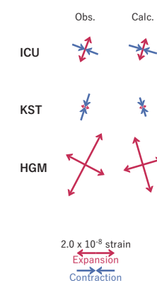
図4 2024/09/21-24 の歪・傾斜変化 (図2 [B]) を説明する断層モデル。
