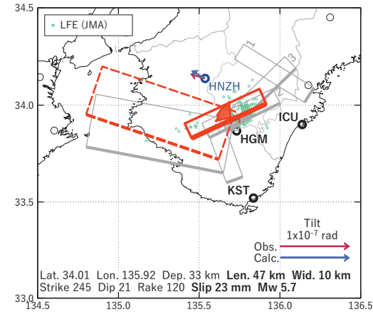
図4 2024/09/21-24 の歪・傾斜変化 (図2 [B]) を説明する断層モデル。
