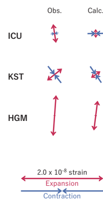
図3 2024/09/07 - 09AM の歪・傾斜変化 (図2 [A]) を説明する断層モデル。
