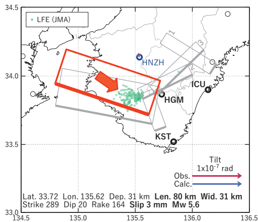
図3 2024/09/07 - 09AM の歪・傾斜変化 (図2 [A]) を説明する断層モデル。
