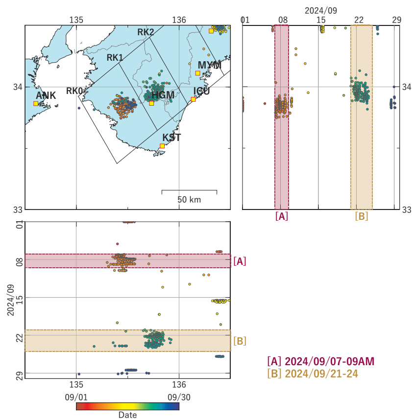
図1 紀伊半島における深部低周波地震の時空間分布図。 (2024/09/01 00:00 - 2024/09/30 00:00 (JST)) 気象庁カタログによる。
