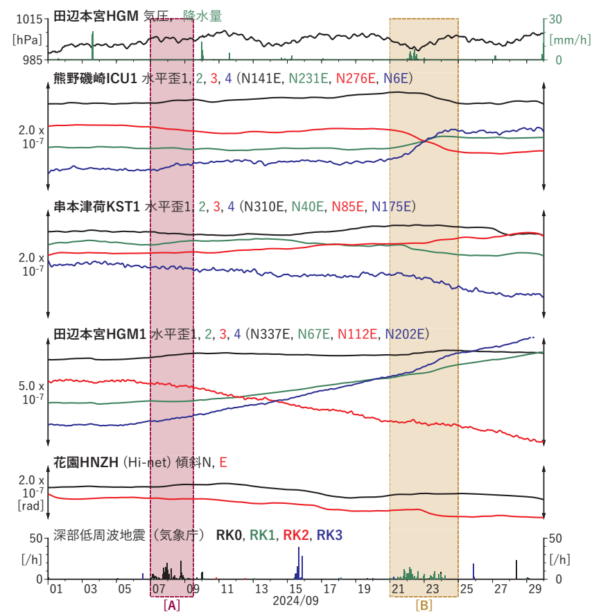
図2 紀伊半島における歪・傾斜の時間変化 (2024/09/01 00:00 - 2024/09/30 00:00 (JST))
