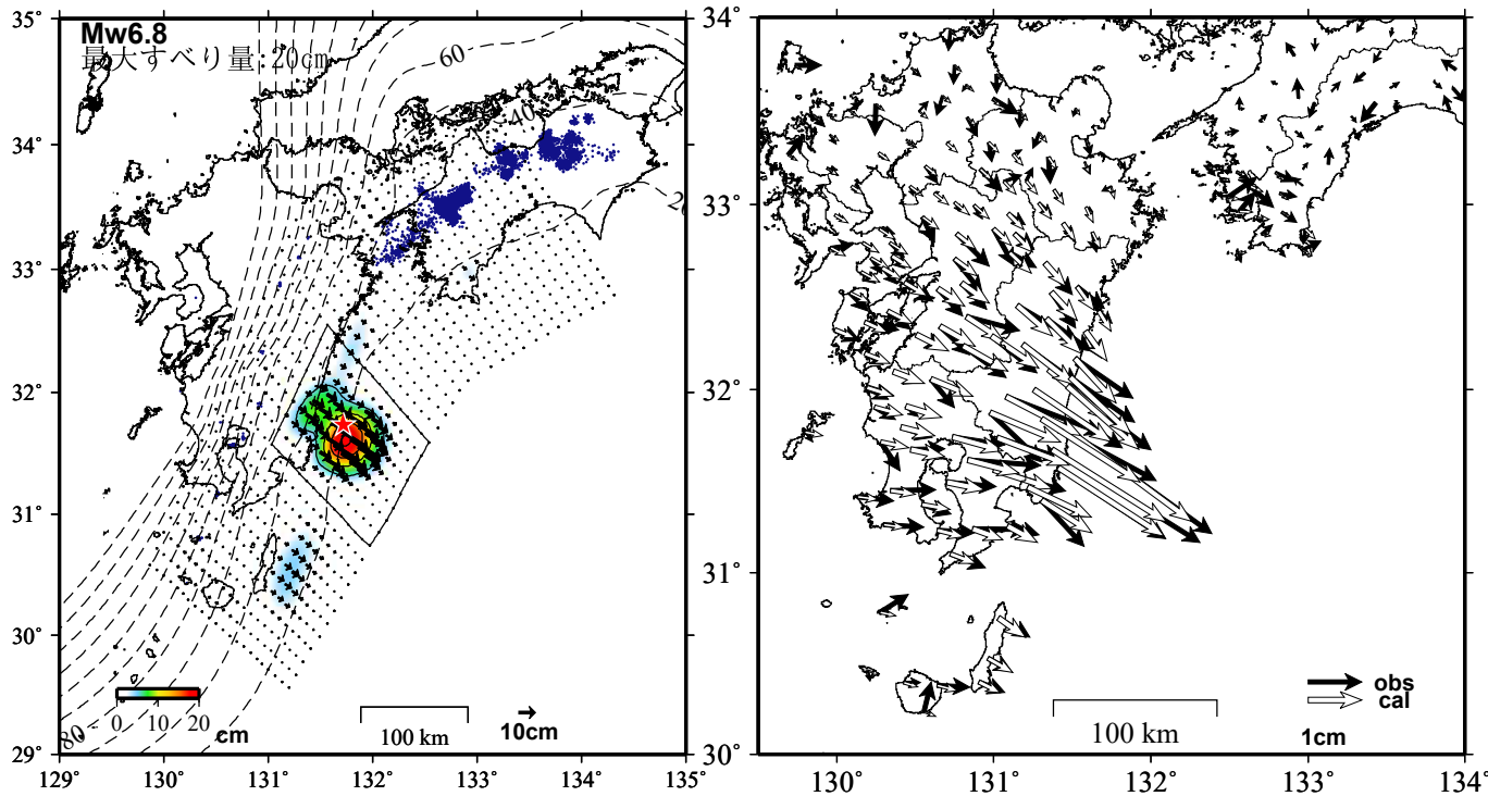
推定すべり分布 (2024-08-06/2024-09-28)
