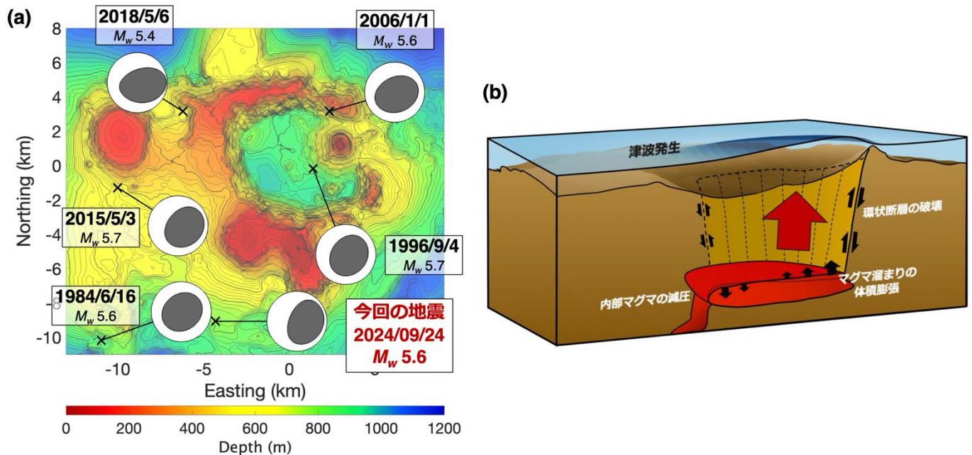
図1. (a) スミスカルデラ周辺で繰り返す地震活動. 1984 年・1996 年・2006 年・2015 年・2018 年については Global CMT catalog の情報に基づく. 2024 年の地震については, CMT 解については防災科学技術研究所の解析結果, モーメントマグニチュードについては米国地質調査所の W-phase の解析解に基づく. なお震源位置には数 km~10km 程度の誤差が含まれることに留意. (b) 2015 年のスミスカルデラ地震に対して提案された「トラップドア断層破壊による海底カルデラ隆起」仮説の模式図 (Sandarbata et al. (2022, JGR: Solid Earth) の図を修正).
