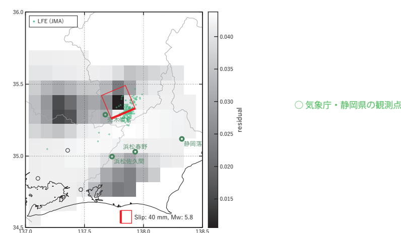
(b1) 推定した断層モデル
