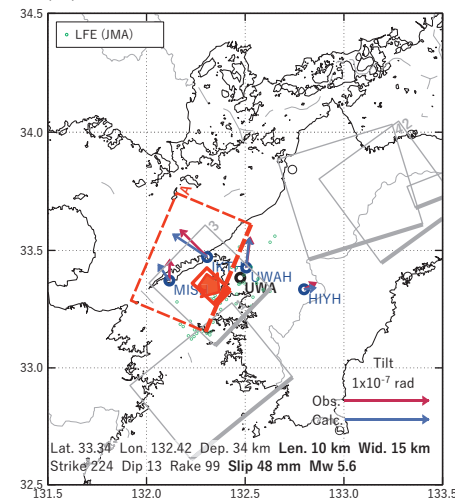
図16 2024/08/22-23の歪・傾斜変化 (図14 [B]) を説明する断層モデル。
