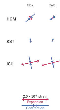
図8 2024/08/07-08 の歪・傾斜変化 (図2~7 [A]) を説明する断層モデル。
