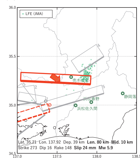
図12 2024/08/13-16の歪・傾斜変化（図2~7 [E]）を説明する断層モデル。
