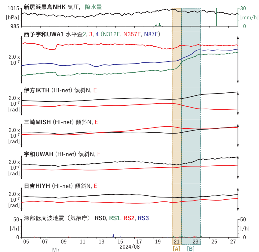
図14 四国地方西部における歪・傾斜の時間変化 (2024/08/05 00:00 - 2024/08/28 00:00 (JST))
