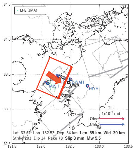
図15 2024/08/21の歪・傾斜変化 (図14 [A]) を説明する断層モデル。
