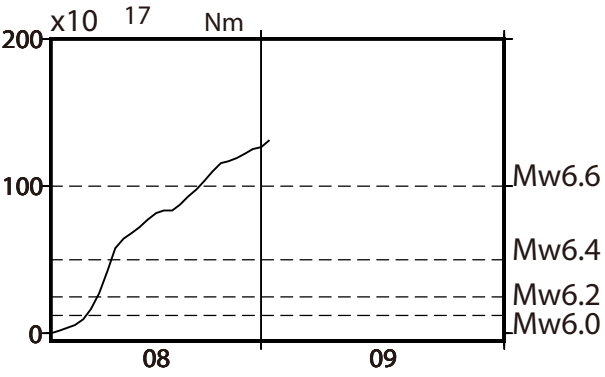
モーメント * 時系列（試算）
