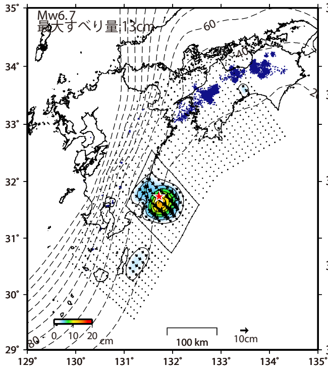
推定すべり分布 (2024-08-06/2024-09-02)
