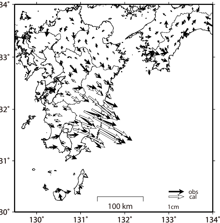
観測値（黒）と計算値（白）の比較 (2024-08-06/2024-09-02)
