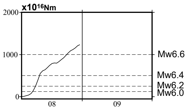
2024年8月8日の地震後の余効すべりの モーメント時系列
