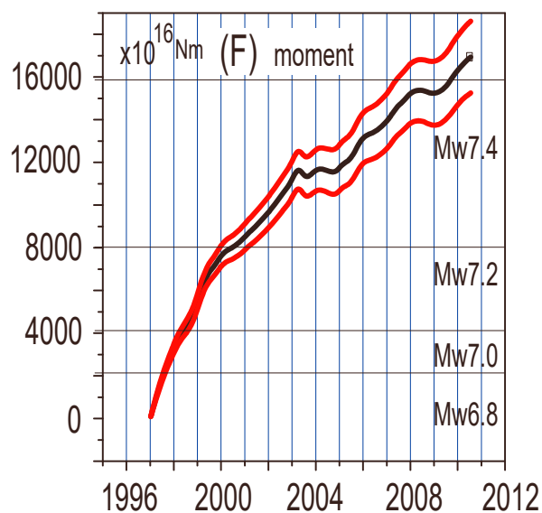
日向灘南部の長期的ゆっくりすべり域の モーメント時系列 (1997年1月～2010年10月)
