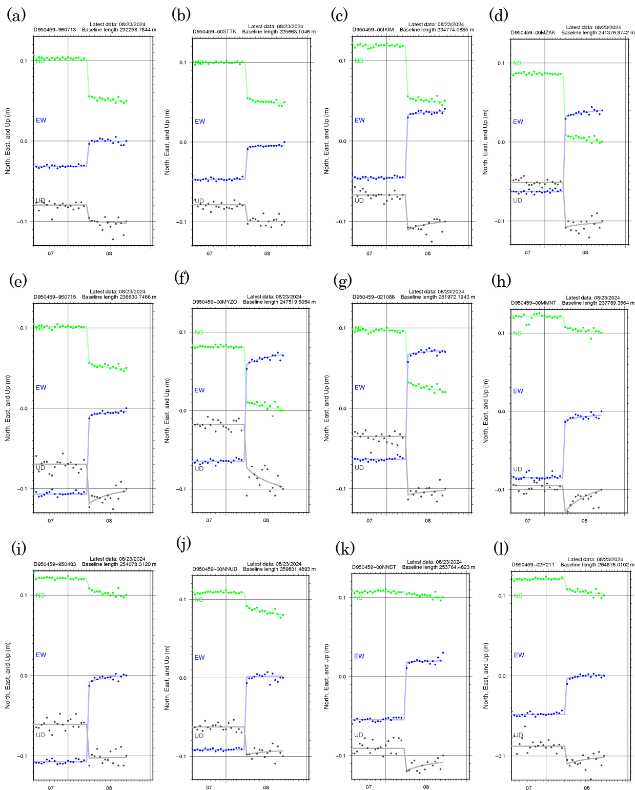
図3 2024 年 8 月 8 日日向灘の地震 (M7.1) 前後の地殻変動 (日座標値、精密暦使用、参照点 GEONET950459 平戸)。地震発生日のデータは取り除いている。横軸の数値は月を表す。薄い実線は地震時ステップと余効変動を対数関数でフィッティングしたもの。最新データは 2024 年 8 月 23 日。 (a) 960713。(b) STTK。(c) IKIM。(d) MZAK。(e) 960715。(f) MYZO。(g) 021088。(h) MMNT。(i) 950483。(j) NNUD。(k) NNST。(l) 02P211。
