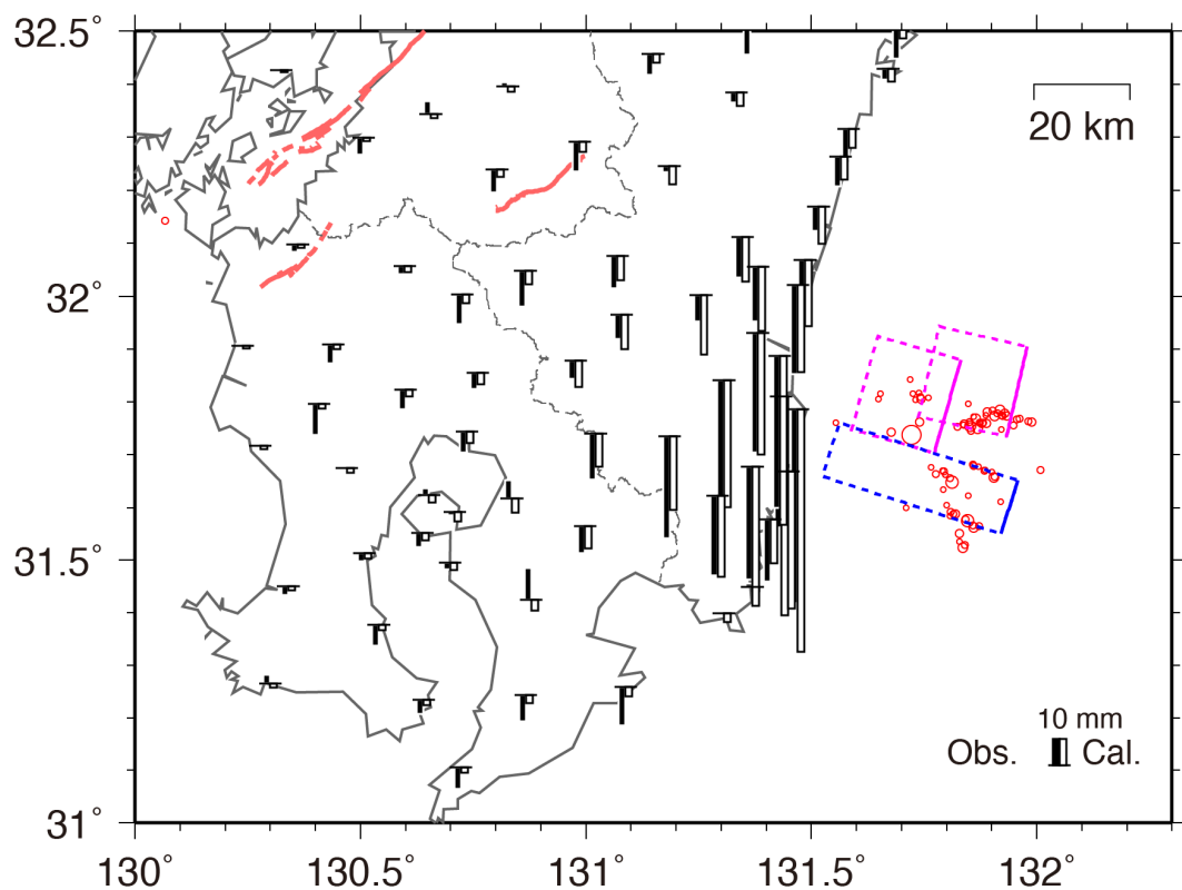
図2 2024年8月8日日向灘の地震(M7.1)の震源断層モデル(青色矩形領域)。矩形断層一様すべりを仮定し、プレート境界に深さ、走向、傾斜を固定して矩形断層の断層パラメータを Matsu'ura and Hasegawa(1988)の手法で推定した。推定された断層パラメータは、N31.655°, E131.741°, 深さ 19.8km、長さ 11.8 km、幅 41.8 km、走向 198°, 傾斜 19°, すべり角 70°, すべり量 2.07m、 M_w 7.08
