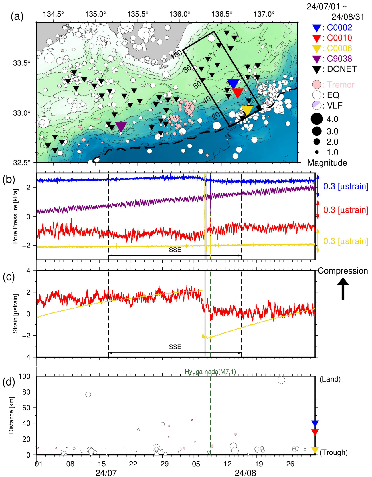
図3 直近2ヶ月間のSSE・低周波微動モニタリング(2024年7月1日~2024年8月31日)。(a) 震央分布図(●:低周波微動(深さ0~15 km)、○:通常地震(深さ0~60 km)、●:超低周波地震のメカニズム解)。●●●●●は、それぞれC0002・C0010・C0006・C9038・DONET観測点。破線はトラフ軸。(b) 長期孔内観測点における間隙水圧変化(—:C0002、—:C0010、—:C0006、—:C9038)。(c) 長期孔内観測点における体積歪変化(—:C0010、—:C0006)。(d) 図3a中に実線で示した矩形領域内における、低周波微動・通常地震・超低周波地震の時空間分布。縦軸は、トラフ軸からの距離(km)。緑点線は、日向灘の地震(8月8日M7.1)。
