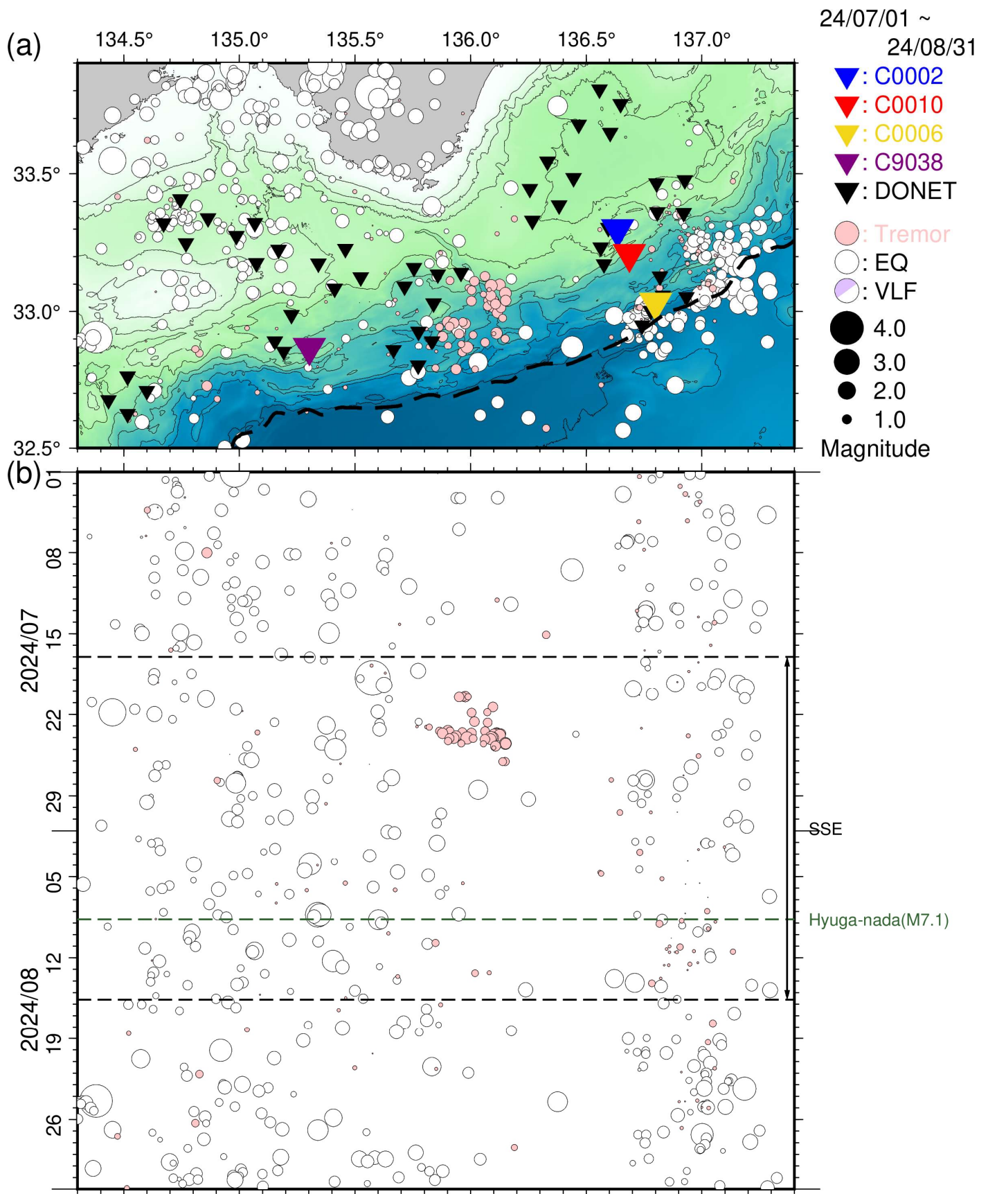
図5 直近2ヵ月間において熊野灘から室戸沖にて発生した低周波微動・通常地震・超低周波地震 (2024年7月1日~2024年8月31日)。図3と同様のシンボルにて表示。(a) 震央分布図。(b) aに示した震央を経度方向へ投影した時空間分布図。
