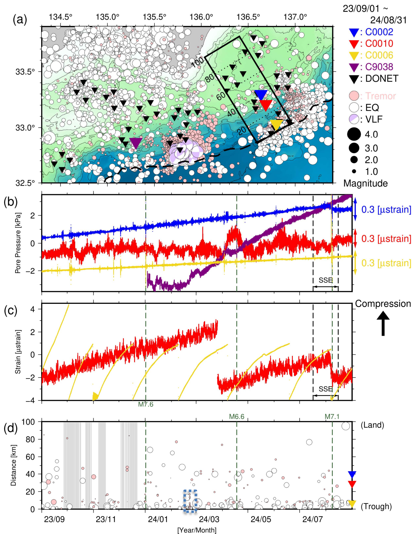
図4 直近1年間のSSE・低周波微動モニタリング(2023年9月1日~2024年8月31日)。(a)低周波微動・通常地震・超低周波地震の震央分布。(b)間隙水圧変化。(c)体積歪変化。(d)時空間分布。灰色はエアガン発振期間。緑点線は、能登地方の地震(1月1日M7.6)、豊後水道の地震(4月17日M6.6)および日向灘の地震(8月8日M7.1)。青点線の長方形領域は、DONET1のCノード付近における低周波微動の群発的な活動を示す。なお、過去資料の図3に緑点線で記した地震のうち、aの領域外かつM6.5未満のものは掲載していない。
