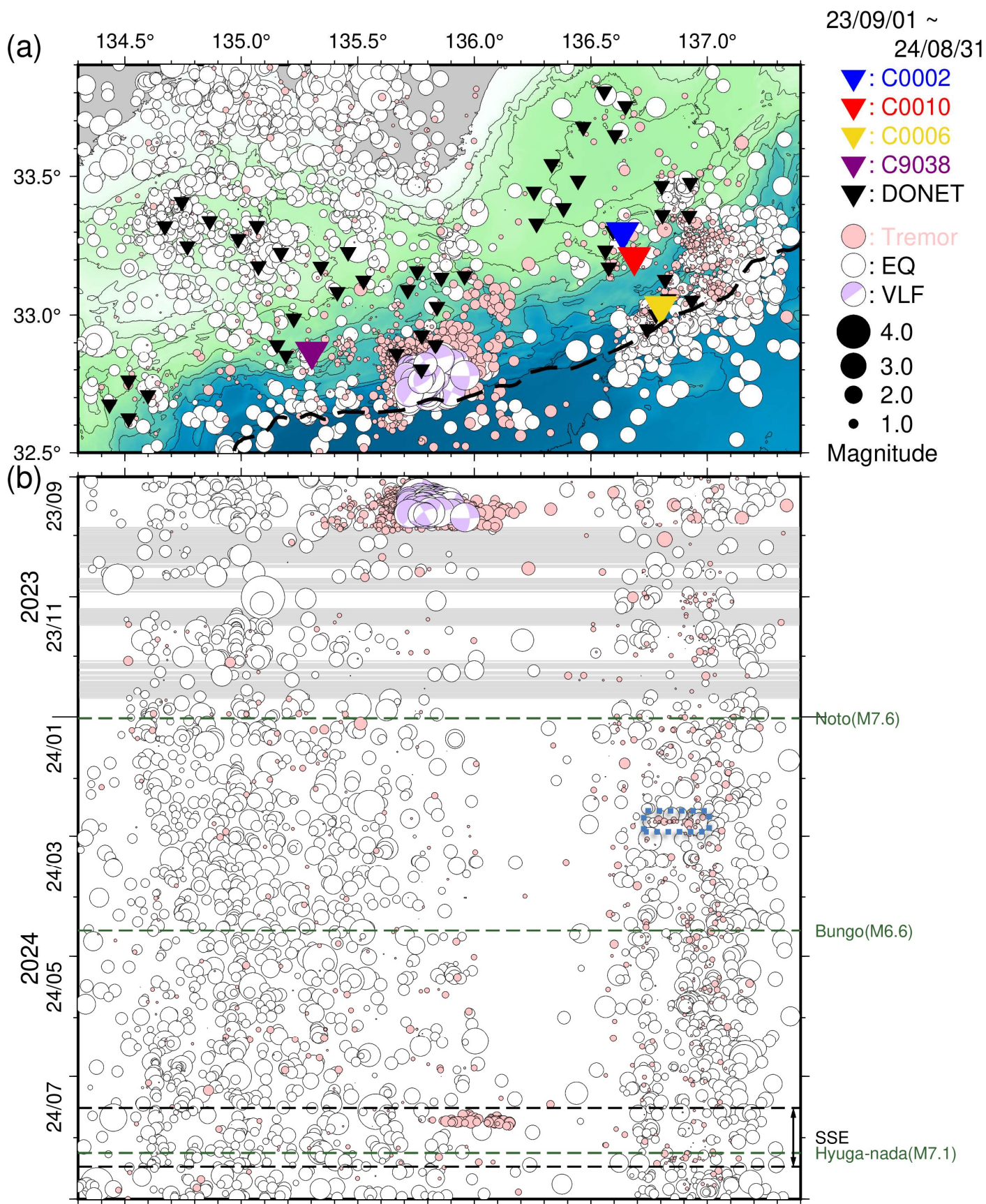
図 6 直近 1 年間に於いて熊野灘から室戸沖にて発生した低周波微動・通常地震・超低周波地震 (2023 年 9 月 1 日~2024 年 8 月 31 日)。図 4 と同様のシンボルにて表示。(a) 震央分布図。(b) a に示した震央を経度方向へ投影した時空間分布図。青点線の長方形領域は、DONET1 の B ノード及び C ノード付近における低周波微動の群発的な活動を示す。なお、過去資料の図 3 及び図 5 に緑点線で記した地震のうち、a の領域外かつ M6.5 未満のものは掲載していない。
