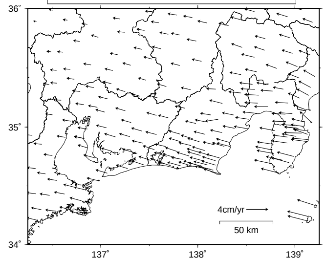
スロースリップ終息後の水平地殻変動速度 (2008年1月～2011年1月)
