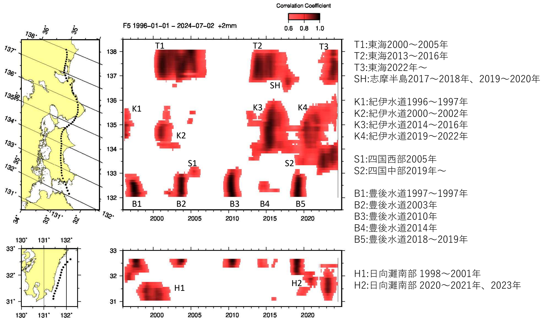
第1図 長期的スロースリップ客観検知図（1996年～2024年7月）
