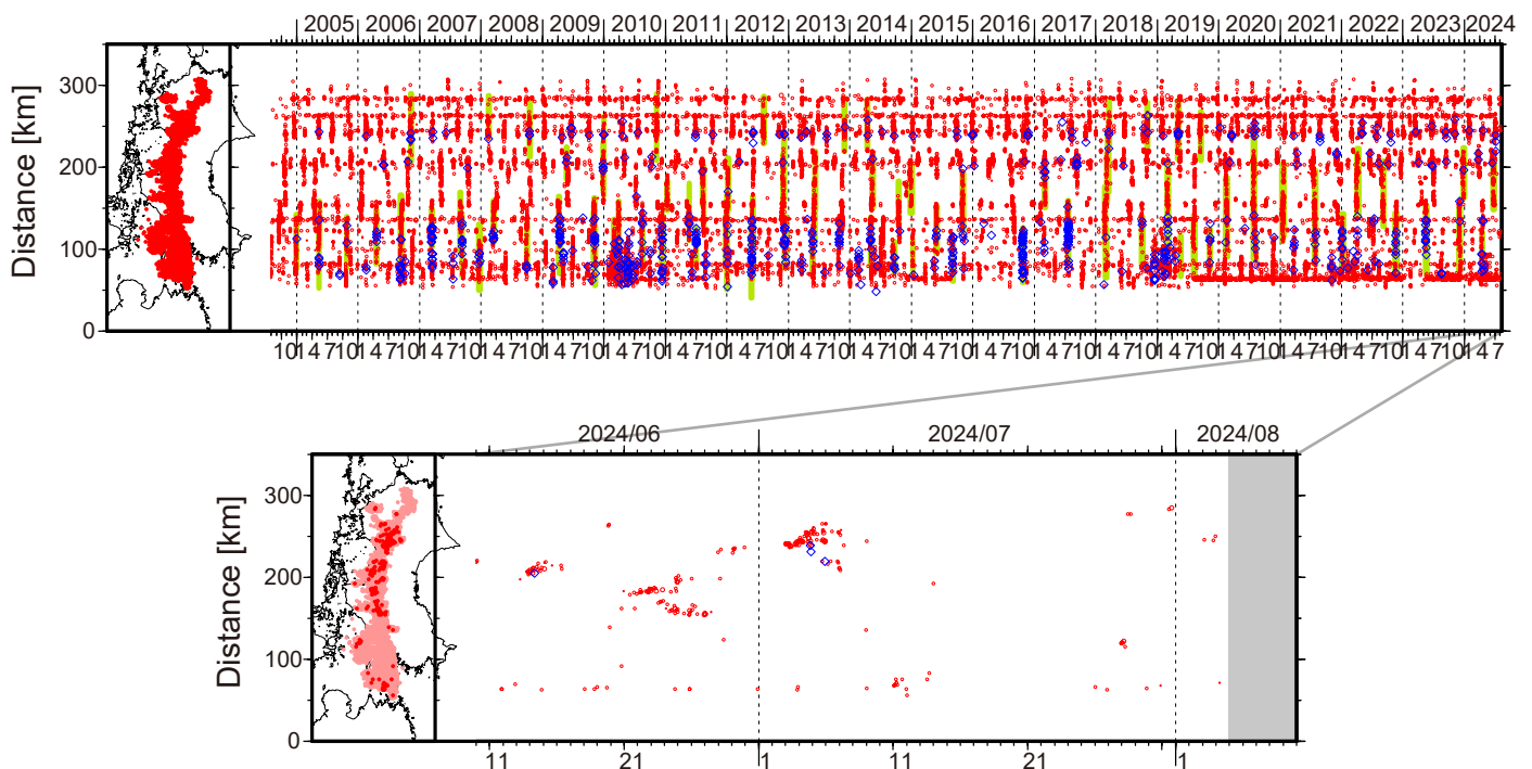
図 1. 四国における 2004 年 8 月～ 2024 年 8 月 4 日までの深部低周波微動の時空間分布（上図）．赤丸はエンベロープ相関・振幅ハイブリッド法 (Maeda and Obara, 2009) およびクラスタ処理 (Obara et al., 2010) によって 1 時間毎に自動処理された微動分布の重心である．青菱形は周期 20 秒に卓越する超低周波地震 (Ito et al., 2007) である．黄緑色太線は、これまでに検出された短期的スロースリップイベント (SSE) を示す．下図は 2024 年 7 月を中心とした期間の拡大図である．7 月 2 ～ 9 日頃には徳島県西部から愛媛県東部で活発な微動活動がみられた．この活動は愛媛・香川・徳島県境付近で開始し、東方向への活動域の拡大がみられた後、5 日頃からは愛媛県東部でも活動がみられた．7 月 11 ～ 12 日頃には豊後水道において、7 月 27 ～ 28 日頃に愛媛県西部において、8 月 3 日頃には愛媛・香川・徳島県境付近において、それぞれごく小規模な活動がみられた．
