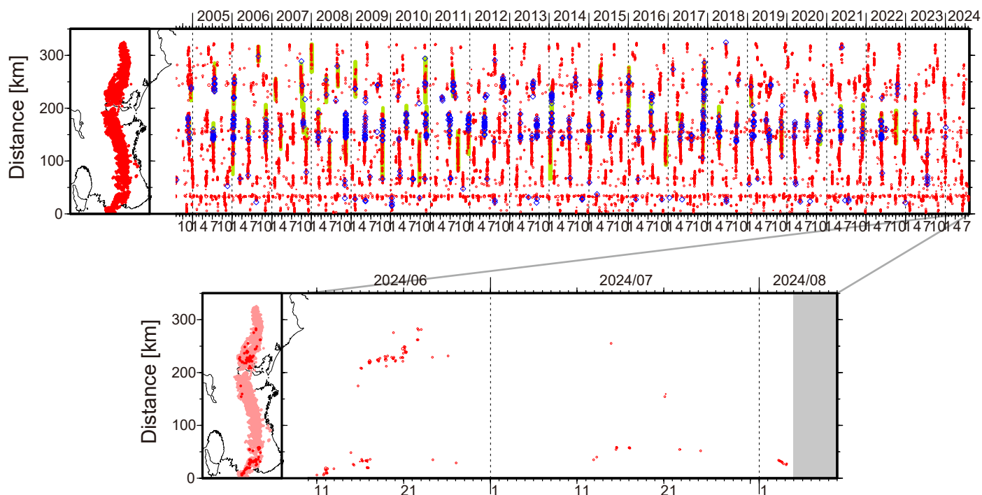
図 1. 紀伊半島・東海地域における 2004 年 8 月～2024 年 8 月 4 日までの深部低周波微動の時空間分布 (上図). 赤丸はエンベロープ相関・振幅ハイブリッド法 (Maeda and Obara, 2009) およびクラスタ処理 (Obara et al., 2010) によって 1 時間毎に自動処理された微動分布の重心である. 青菱形は周期 20 秒に卓越する超低周波地震 (Ito et al., 2007) である. 黄緑色の太線はこれまでに検出された短期的スロースリップイベント (SSE) を示す. 下図は 2024 年 7 月を中心とした期間の拡大図である. 7 月以降の期間に顕著な活動はとくにみられなかったものの, 7 月 15 日および 17 日頃には奈良・和歌山県境付近において, 8 月 3～4 日頃には和歌山県中部において, それぞれごく小規模な活動がみられた.
