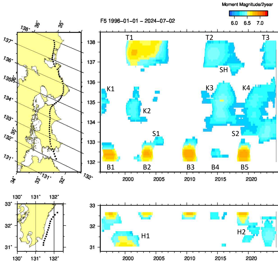
第2図 長期的スロースリップの規模分布（1996年～2024年7月） 2年間あたりの変化量から推定したモーメントマグニチュード。
