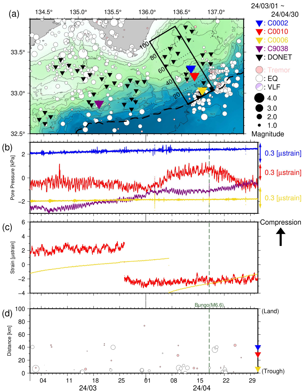
図3 直近2ヶ月間のSSE・低周波微動モニタリング(2024年3月1日~2024年4月30日)。(a)震央分布図(●:低周波微動(深さ0~15km)、○:通常地震(深さ0~60km)、●:超低周波地震のメカニズム解)。▼、▼、▼、▼、▼は、それぞれC0002・C0010・C0006・C9038・DONET観測点。破線はトラフ軸。(b)長期孔内観測点における間隙水圧変化(—:C0002、—:C0010、—:C0006、—:C9038)。(c)長期孔内観測点における体積歪変化(—:C0010、—:C0006)。(d)図3a中に実線で示した矩形領域内における、低周波微動・通常地震・超低周波地震の時空間分布。緑点線は、豊後水道の地震(4月17日M6.6)。縦軸は、トラフ軸からの距離(km)。
