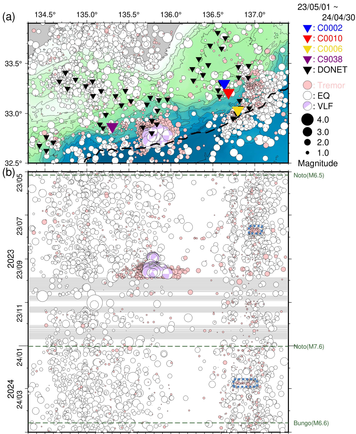
図 6 直近 1 年間に於いて熊野灘から室戸沖にて発生した低周波微動・通常地震・超低周波地震 (2023 年 5 月 1 日~2024 年 4 月 30 日)。図 4 と同様のシンボルにて表示。(a) 震央分布図。(b) a に示した震央を経度方向へ投影した時空間分布図。青点線の長方形領域は、DONET1 の B ノード及び C ノード付近における低周波微動の群発的な活動を示す。なお、過去資料の図 3 及び図 5 に緑点線で記した地震のうち、a の領域外かつ M6.5 未満のものは掲載していない。
