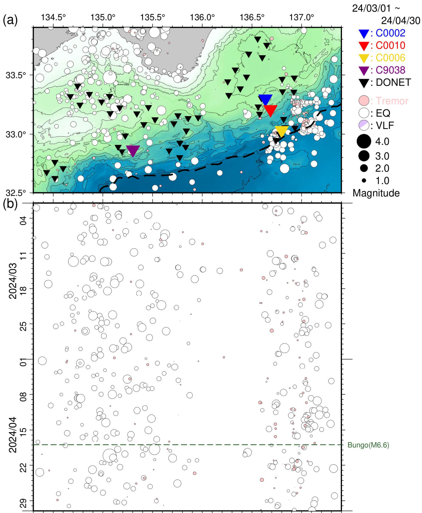
図5 直近2ヵ月間において熊野灘から室戸沖にて発生した低周波微動・通常地震・超低周波地震 (2024年3月1日~2024年4月30日)。図3と同様のシンボルにて表示。(a) 震央分布図。(b) aに示した震央を経度方向へ投影した時空間分布図。
