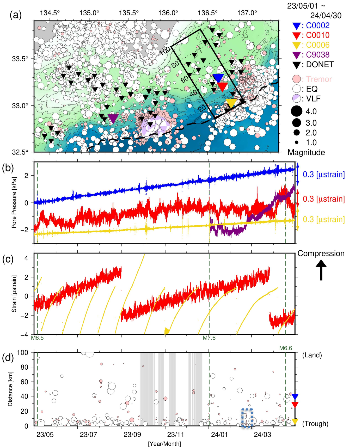
図4 直近1年間のSSE・低周波微動モニタリング（2023年5月1日～2024年4月30日）。(a) 低周波微動・通常地震・超低周波地震の震央分布。(b) 間隙水圧変化。(c) 体積歪変化。(d) 時空間分布。灰色はエアガン発振期間。緑点線は、能登地方の地震（2023年5月5日M6.5と2024年1月1日M7.6）および豊後水道の地震（4月17日M6.6）。青点線の長方形領域は、DONET1のCノード付近における低周波微動の群発的な活動を示す。なお、過去資料の図3に緑点線で記した地震のうち、aの領域外かつM6.5未満のものは掲載していない。
