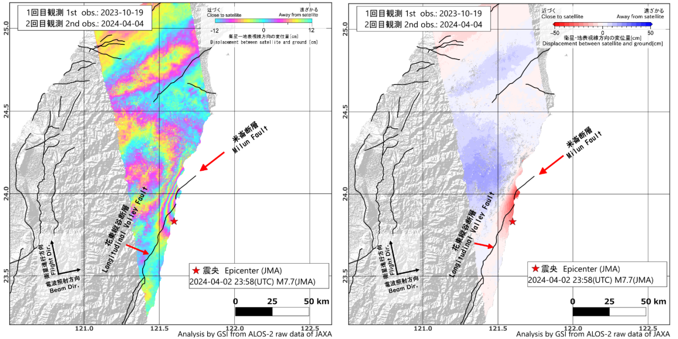
図1. SAR干渉解析結果(右はアンラップ済み)。震央はJMAによる。断層線はStyron et al. (2020)より。
