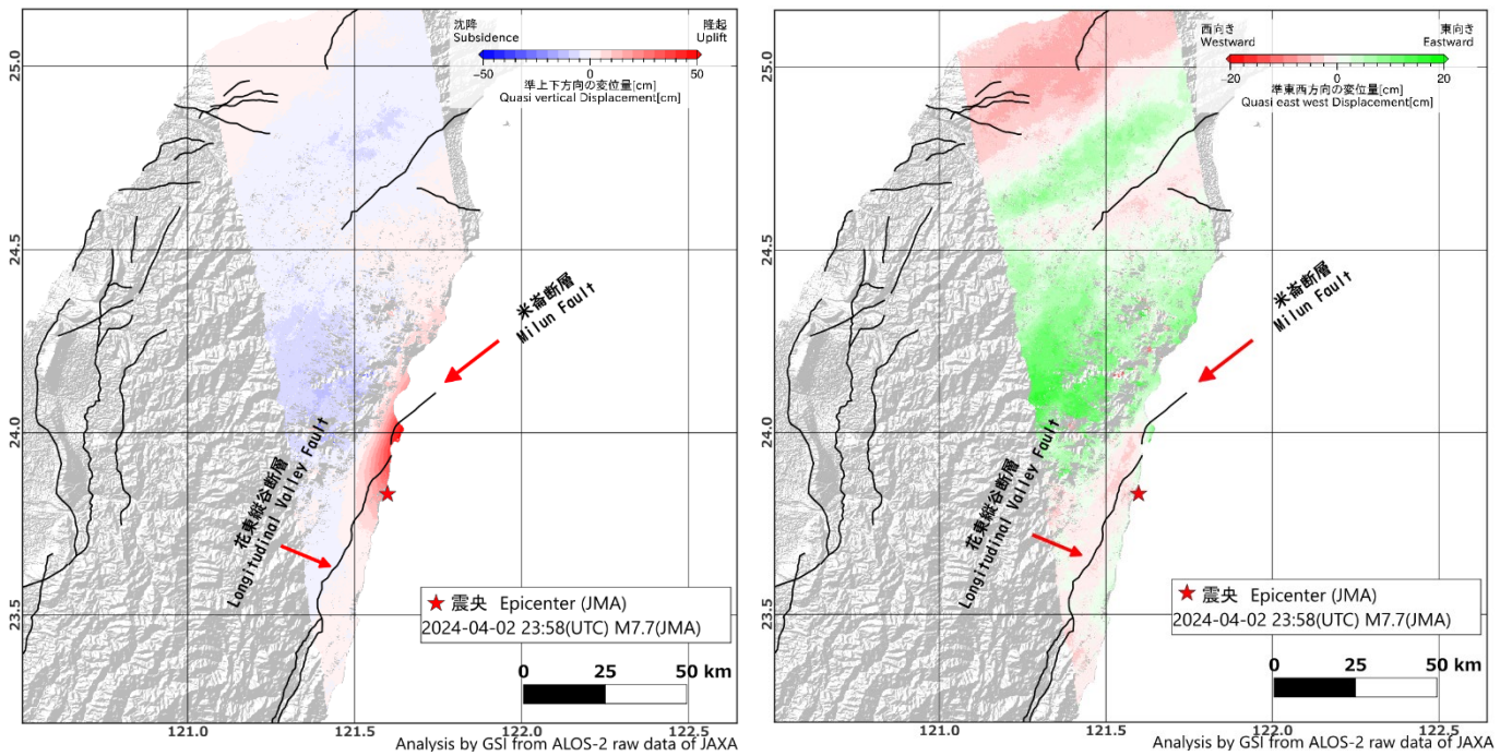
図3. 図1と図2での2.5次元解析結果。震央はJMAによる。断層線はStyron et al. (2020)より。
