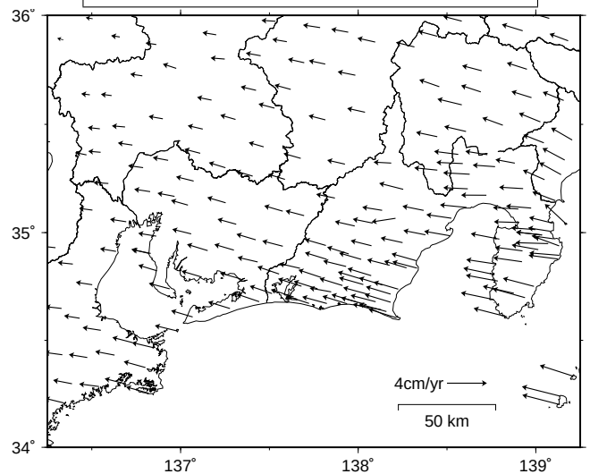
スロースリップ終息後の水平地殻変動速度 (2008年1月～2011年1月)
