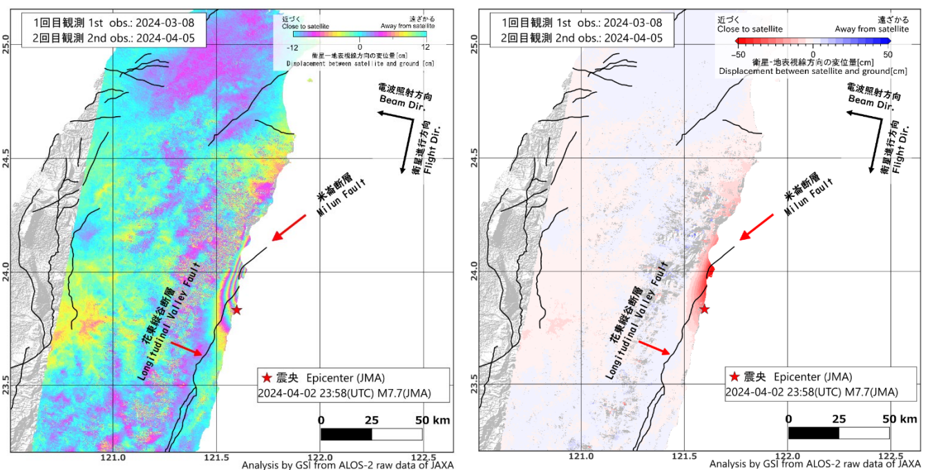
図2. SAR干渉解析結果(右はアンラップ済み)。震央はJMAによる。断層線はStyron et al. (2020)より。
