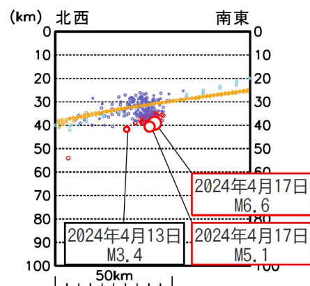
今回の地震の震央周辺※の断面図
