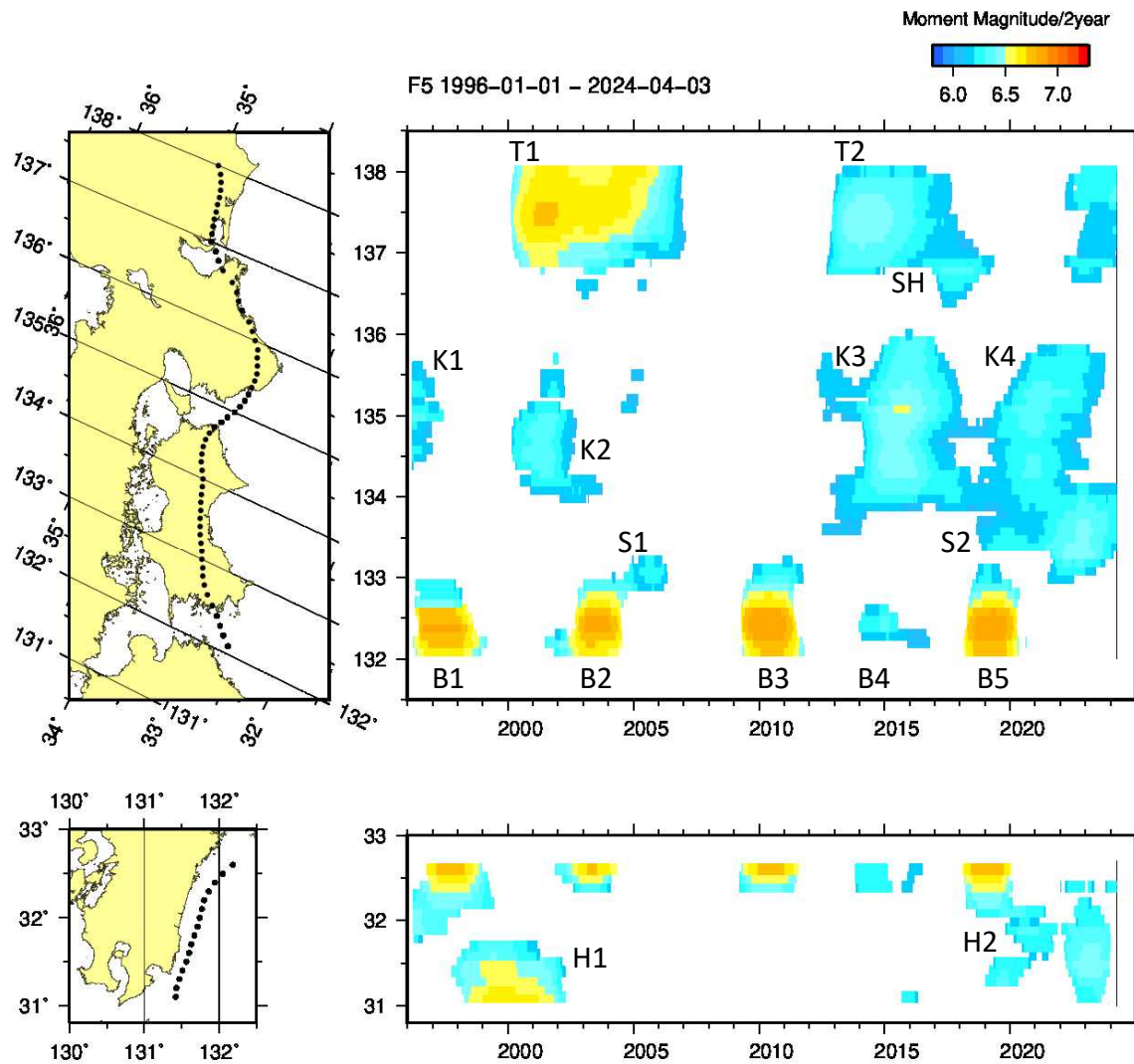
第2図 長期的スロースリップの規模分布（1996年～2024年4月） 2年間あたりの変化量から推定したモーメントマグニチュード。
