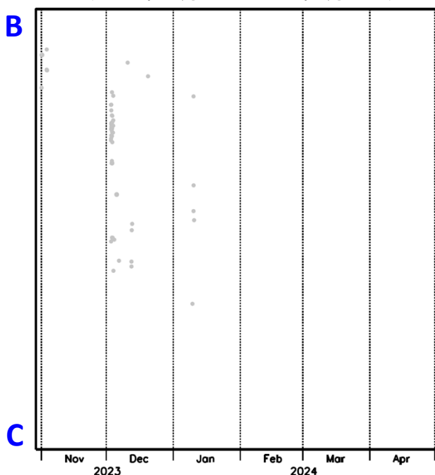
領域a内の時空間分布図(B-C投影) (2023年11月1日～2024年4月30日)
