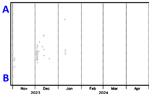
領域a内の時空間分布図(A-B投影) (2023年11月1日～2024年4月30日)
