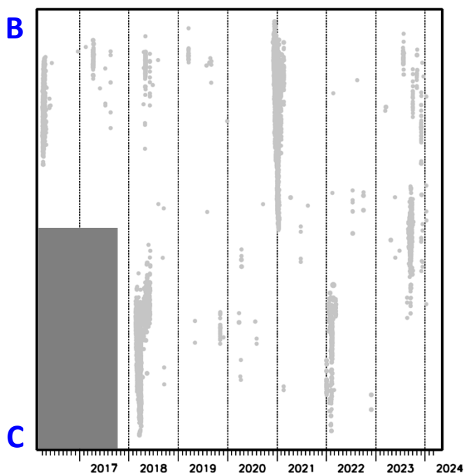
領域a内の時空間分布図(B-C投影) (2016年4月1日～2024年4月30日)
