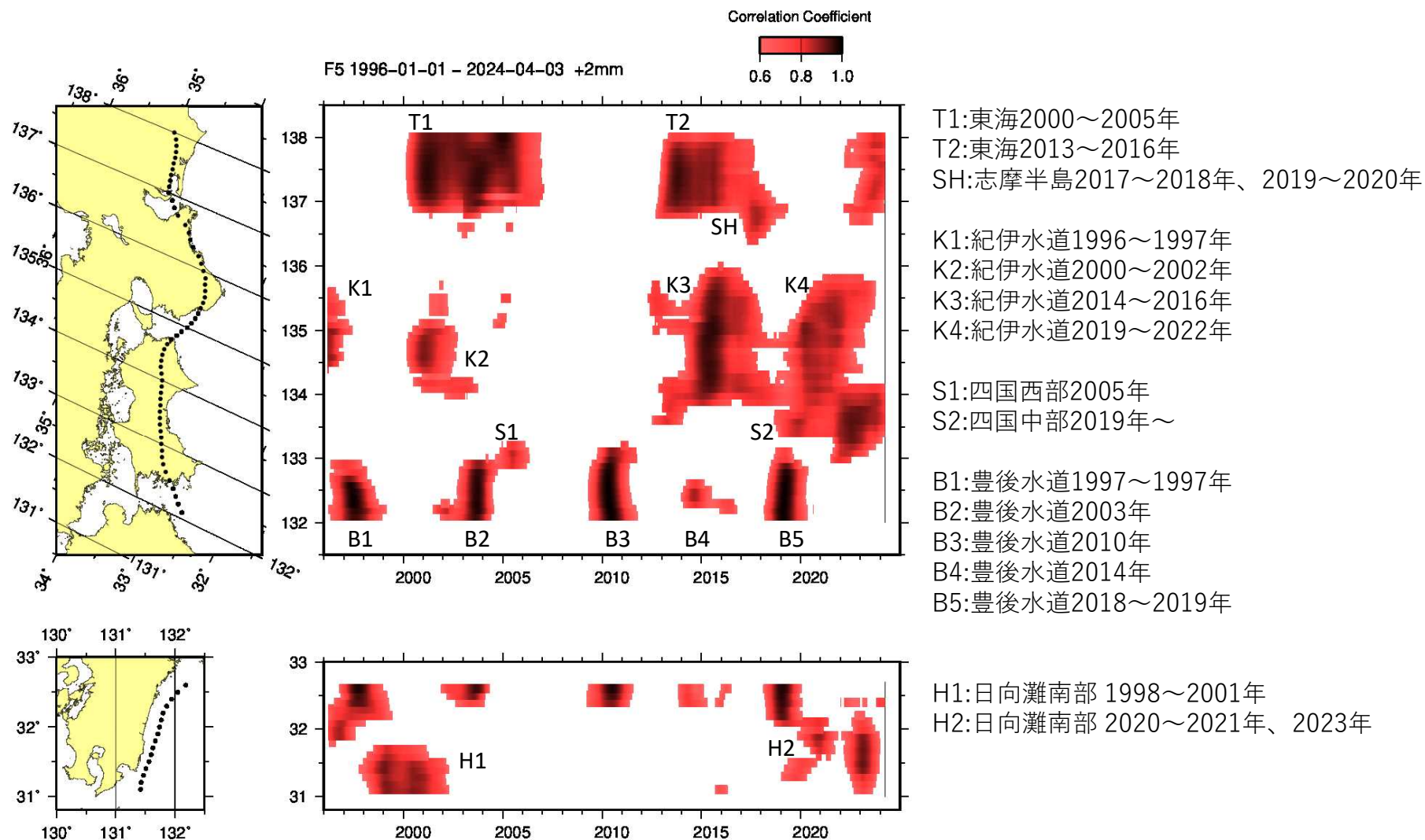
第1図 長期的スロースリップ客観検知図（1996年～2024年4月）
