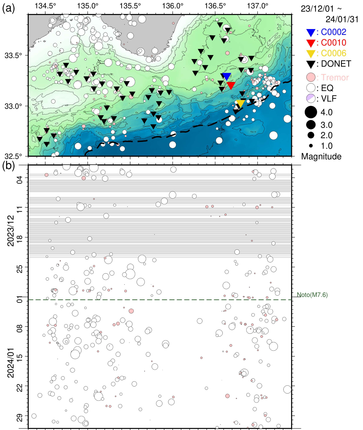
図5 直近2ヵ月間において熊野灘から室戸沖にて発生した低周波微動・通常地震・超低周波地震（2023年12月1日～2024年1月31日）。図3と同様のシンボルにて表示。(a) 震央分布図。(b) aに示した震央を経度方向へ投影した時空間分布図。
