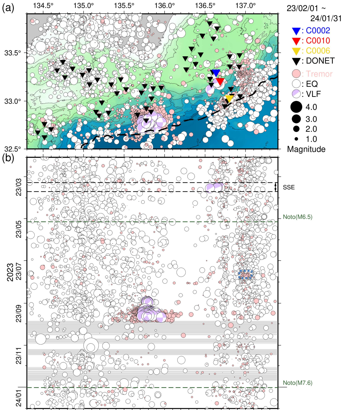
図 6 直近 1 年間に於いて熊野灘から室戸沖にて発生した低周波微動・通常地震・超低周波地震 (2023 年 2 月 1 日~2024 年 1 月 31 日)。図 4 と同様のシンボルにて表示。(a) 震央分布図。(b) a に示した震央を經度方向へ投影した時空間分布図。青点線の長方形領域は、DONET1 の B ノード付近における低周波微動の群発的な活動を示す。なお、過去資料の図 3 及び図 5 に緑点線で記した地震のうち、a の領域外かつ M6.5 未満のものは掲載していない。
