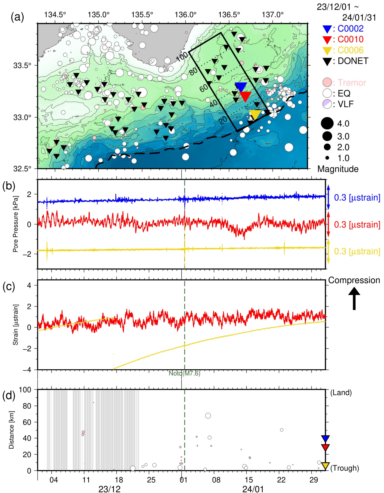
図 3 直近 2 ヶ月間の SSE・低周波微動モニタリング (2023 年 12 月 1 日~2024 年 1 月 31 日)。 (a) 震央分布図 (●: 低周波微動 (深さ 0~15 km)、○: 通常地震 (深さ 0~60 km)、●: 超低周波地震のメカニズム解)。▼: C0002・C0010・C0006・DONET 観測点。破線はトラフ軸。(b) 長期孔内観測点における間隙水圧変化 (—: C0002、—: C0010、—: C0006)。(c) 長期孔内観測点における体積歪変化 (—: C0010、—: C0006)。(d) 図 3a 中に実線で示した矩形領域内における、低周波微動・通常地震・超低周波地震の時空間分布。緑点線は、能登地方の地震 (2024 年 1 月 1 日 M7.6)。縦軸は、トラフ軸からの距離 (km)。灰色はエアガン発振期間。
