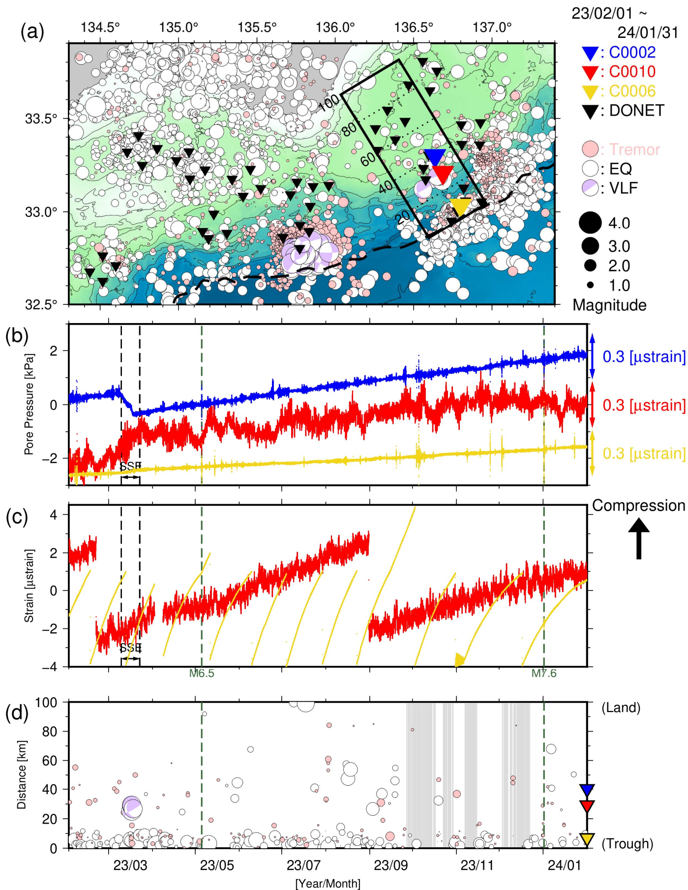
図4 直近1年間のSSE・低周波微動モニタリング(2023年2月1日~2024年1月31日)。(a)低周波微動・通常地震・超低周波地震の震央分布。(b)間隙水圧変化。(c)体積歪変化。(d)時空間分布。緑点線は、能登地方の地震(2023年5月5日M6.5と2024年1月1日M7.6)。なお、過去資料の図3に緑点線で記した地震のうち、aの領域外かつM6.5未満のものは掲載していない。
