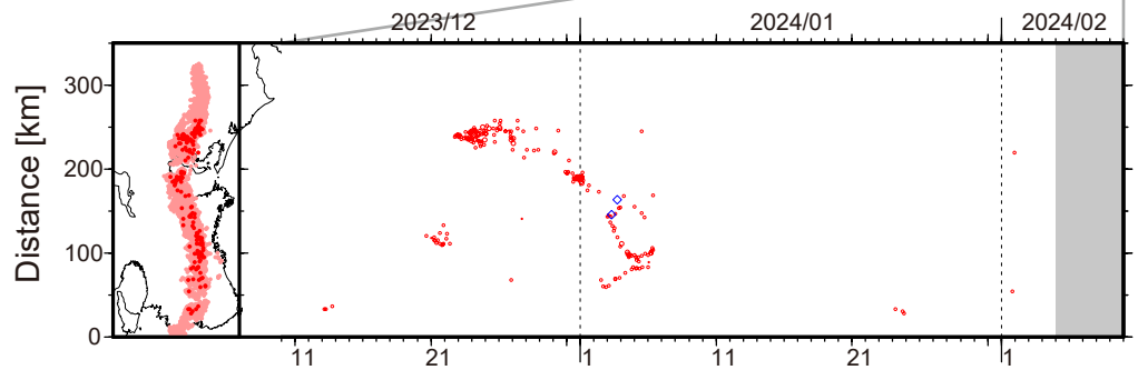
図1. 紀伊半島・東海地域における2004年2月～2024年2月4日までの深部低周波微動の時空間分布(上図). 赤丸はエンベロップ相関・振幅ハイブリッド法 (Maeda and Obara, 2009) およびクラスタ処理 (Obara et al., 2010) によって1時間毎に自動処理された微動分布の重心である. 青菱形は周期20秒に卓越する超低周波地震 (Ito et al., 2007) である. 黄緑色の太線はこれまでに検出された短期的スロースリップイベント (SSE) を示す. 下図は2024年1月を中心とした期間の拡大図である. 12月22日～1月6日頃には、愛知県中部から奈良県南部において活発な活動がみられた. この活動は愛知県中部での開始後、東西方向への活動域の拡大がややみられたのち、27日頃からいったん低調となった. その後12月30日頃から伊勢湾付近で活動が開始し南西方向への活動域の移動がみられた. またこの活動に対し、1月2日頃から奈良県南部で開始した活動が北東方向に移動し、1月4日頃に合流した. 1月24日頃には和歌山県中部において、ごく小規模な活動がみられた.
