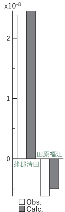
(b3) 体積歪
