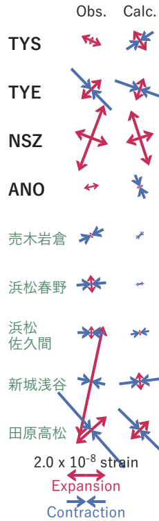
(b2) 主歪
