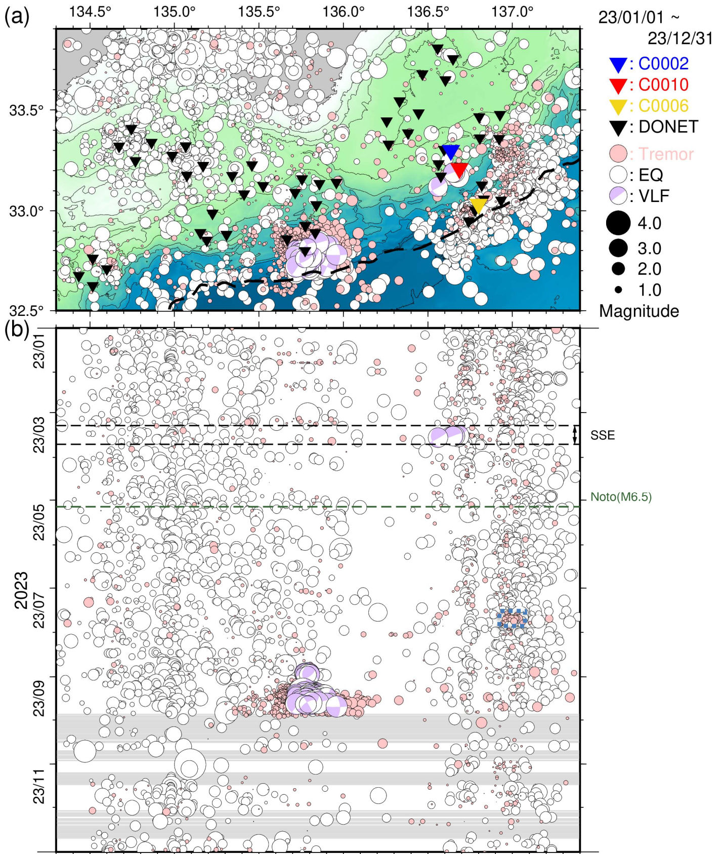
図 6 直近 1 年間に於いて熊野灘から室戸沖にて発生した低周波微動・通常地震・超低周波地震 (2023 年 1 月 1 日~2023 年 12 月 31 日)。図 4 と同様のシンボルにて表示。(a) 震央分布図。(b) a に示した震央を経度方向へ投影した時空間分布図。青点線の長方形領域は、DONET1 の B ノード付近における低周波微動の群発的な活動を示す。なお、図 3 および図 5 において過去資料に緑点線で記した地震のうち、a の領域外かつ M6.5 未満のものは掲載していない。
