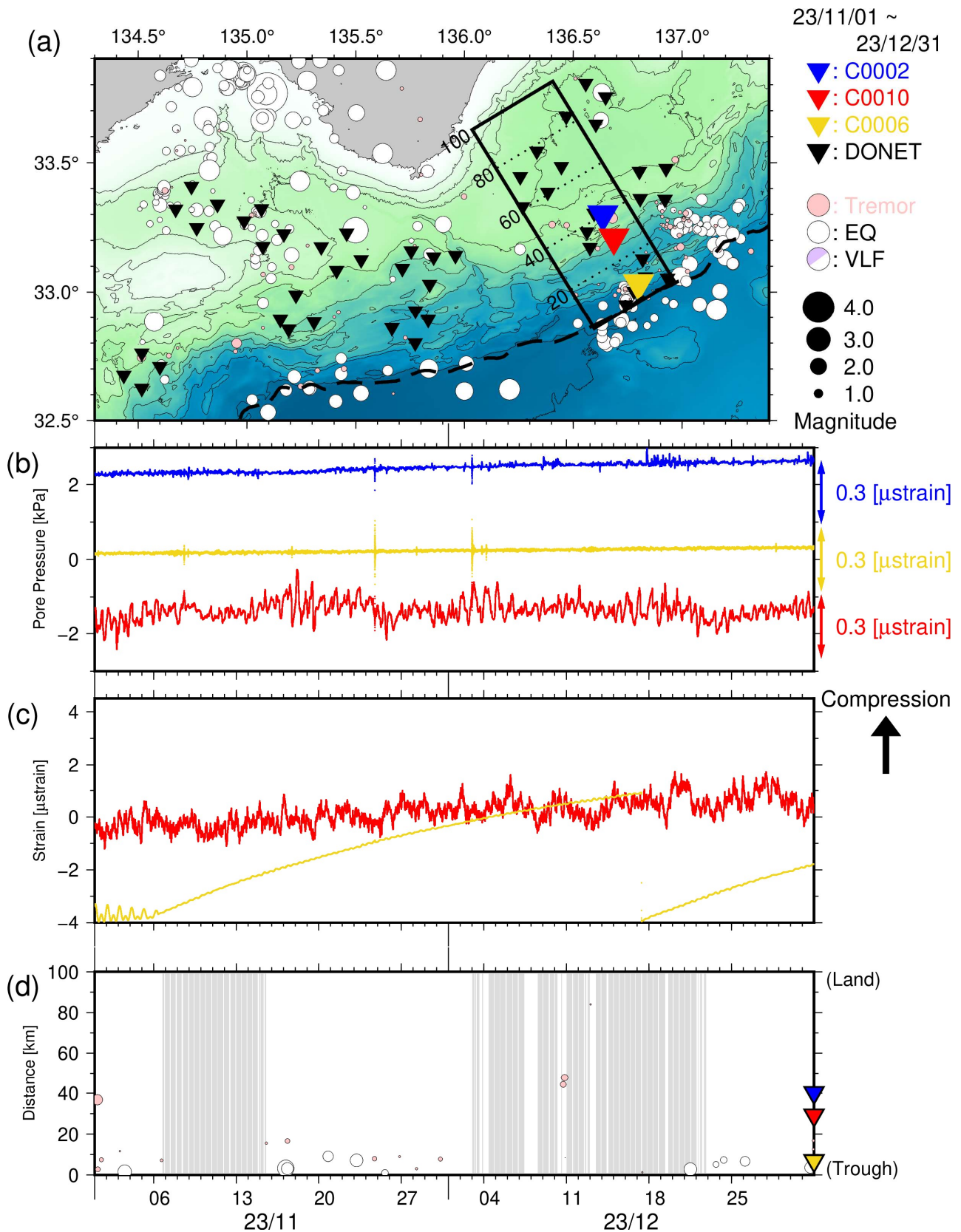
図3 直近2ヶ月間のSSE・低周波微動モニタリング(2023年11月1日~2023年12月31日)。 (a) 震央分布図(●:低周波微動(深さ0~15km)、○:通常地震(深さ0~60km)、●:超低周波地震のメカニズム解)。▼▼▼▼は、それぞれC0002・C0010・C0006・DONET観測点。破線はトラフ軸。(b) 長期孔内観測点における間隙水圧変化(—:C0002、—:C0010、—:C0006)。(c) 長期孔内観測点における体積歪変化(—:C0010、—:C0006)。(d) 図3a中に実線で示した矩形領域内における、低周波微動・通常地震・超低周波地震の時空間分布。縦軸は、トラフ軸からの距離(km)。灰色はエアガン発振期間を示す。
