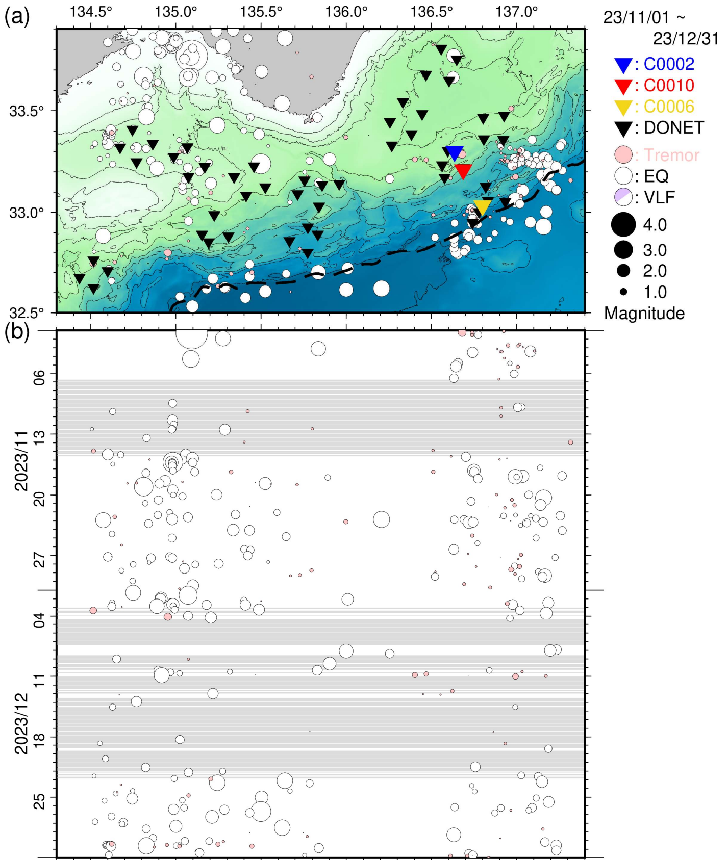
図5 直近2ヵ月間において熊野灘から室戸沖にて発生した低周波微動・通常地震・超低周波地震 (2023年11月1日~2023年12月31日)。図3と同様のシンボルにて表示。(a) 震央分布図。(b) aに示した震央を経度方向へ投影した時空間分布図。
