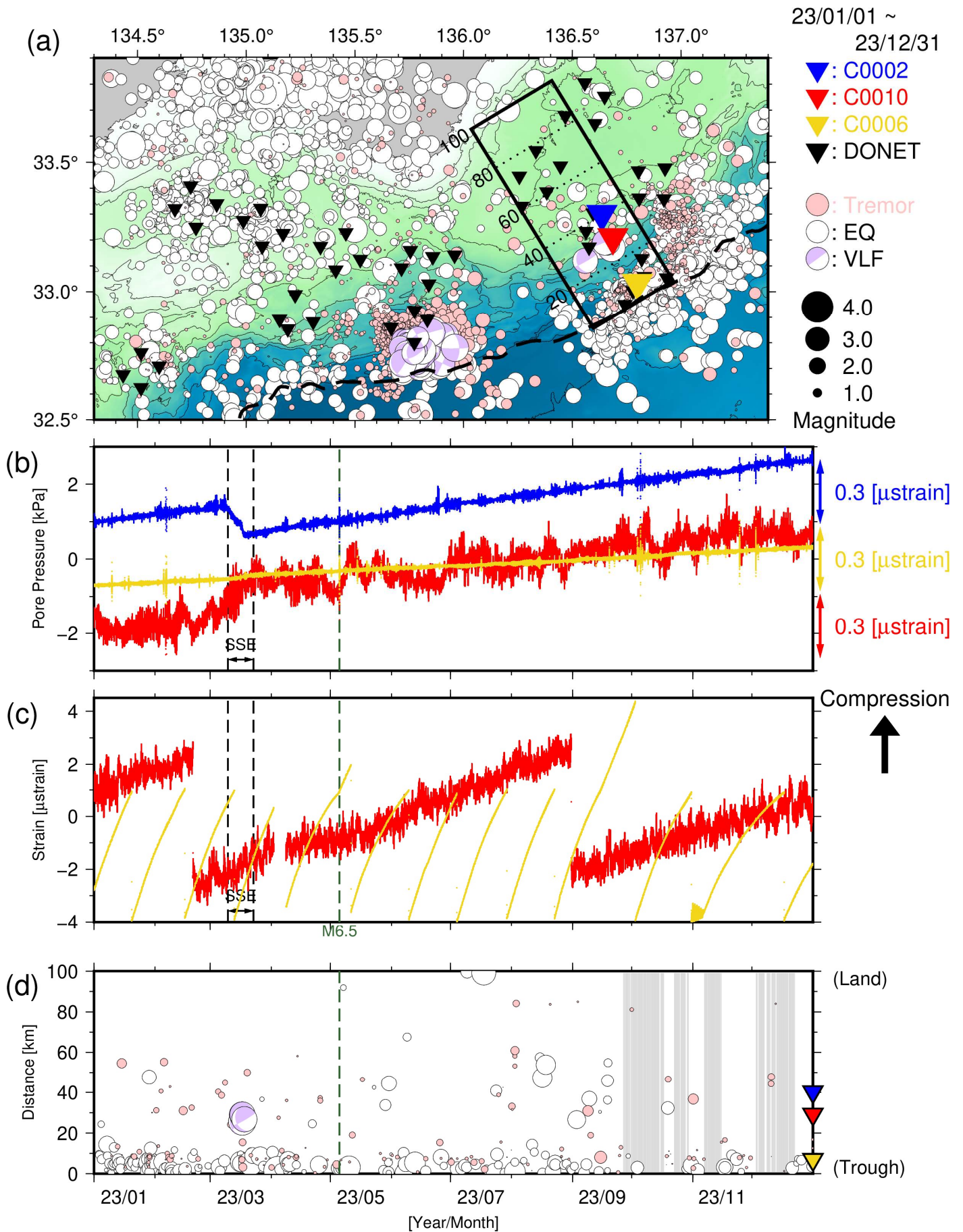
図4 直近1年間のSSE・低周波微動モニタリング(2023年1月1日~2023年12月31日)。(a)低周波微動・通常地震・超低周波地震の震央分布。(b)間隙水圧変化。(c)体積歪変化。(d)時空間分布。緑点線は、5月5日の能登地方地震を示す。なお、図3において過去資料に緑点線で記した地震のうち、aの領域外かつM6.5未満のものは掲載していない。
