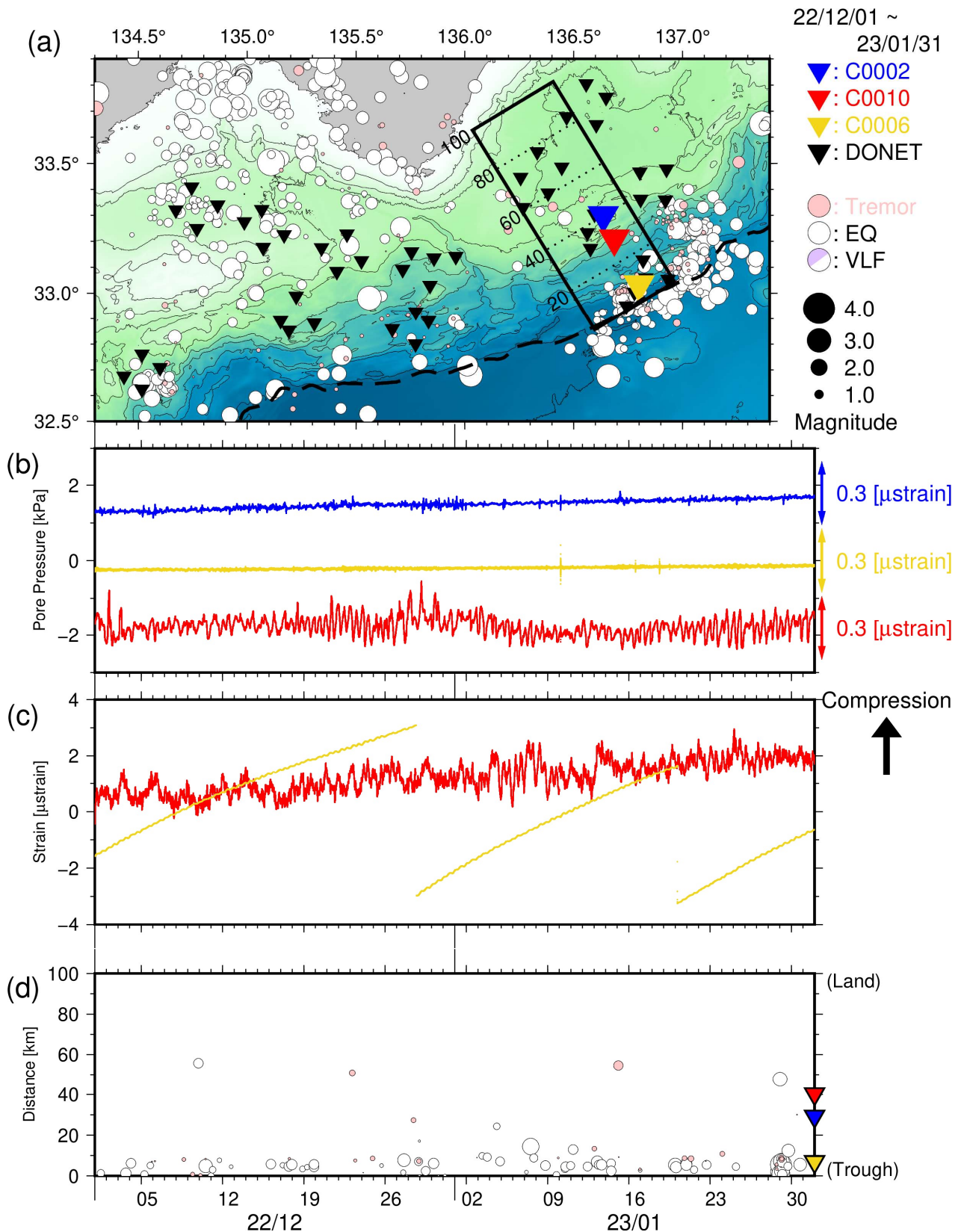
図3 直近2ヶ月間のSSE・低周波微動モニタリング(2022年12月1日~2023年1月31日)。 (a) 震央分布図(●:低周波微動(深さ0~15km)、○:通常地震(深さ0~60km)、●:超低周波地震のメカニズム解)。▼▼▼▼は、それぞれC0002・C0010・C0006・DONET観測点。破線はトラフ軸。(b) 長期孔内観測点における間隙水圧変化(—:C0002、—:C0010、—:C0006)。(c) 長期孔内観測点における体積歪変化(—:C0010、—:C0006)。(d) 図3a中に実線で示した矩形領域内における、低周波微動・通常地震・超低周波地震の時空間分布。灰色はエアガン発振期間。縦軸は、トラフ軸からの距離(km)。
