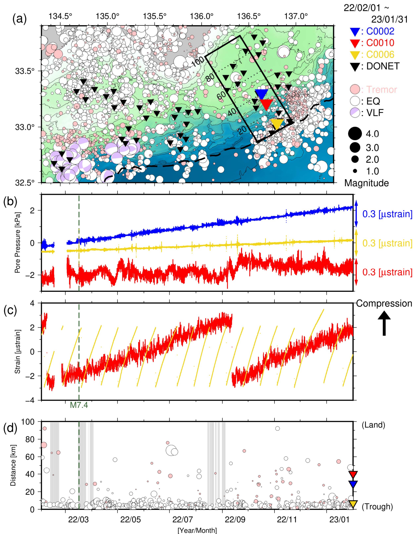
図4 直近1年間のSSE・低周波微動モニタリング(2022年2月1日~2023年1月31日)。(a)低周波微動・通常地震・超低周波地震の震央分布。(b)間隙水圧変化。(c)体積歪変化。(d)時空間分布。灰色はエアガン発振期間を示す。(b-d)の緑点線は3月16日福島県沖地震。なお、図3において過去資料に緑点線で記した地震のうち、aの領域外かつM6.5未満のものは掲載していない。
