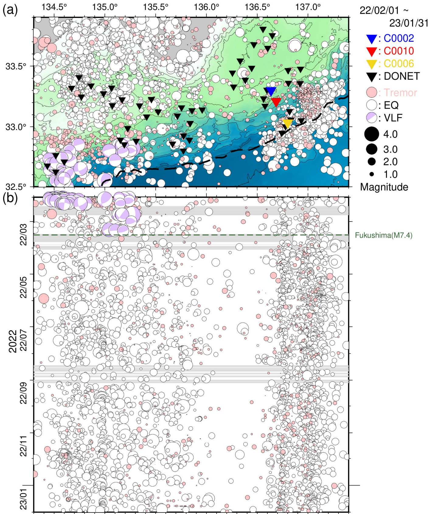
図 6 直近 1 年間に於いて熊野灘から室戸沖にて発生した低周波微動・通常地震・超低周波地震 (2022 年 2 月 1 日~2023 年 1 月 31 日)。図 4 と同様のシンボルにて表示。(a) 震央分布図。(b) a に示した震央を経度方向へ投影した時空間分布図。なお、図 3 および図 5 において過去資料に緑点線で記した地震のうち、a の領域外かつ M6.5 未満のものは掲載していない。
