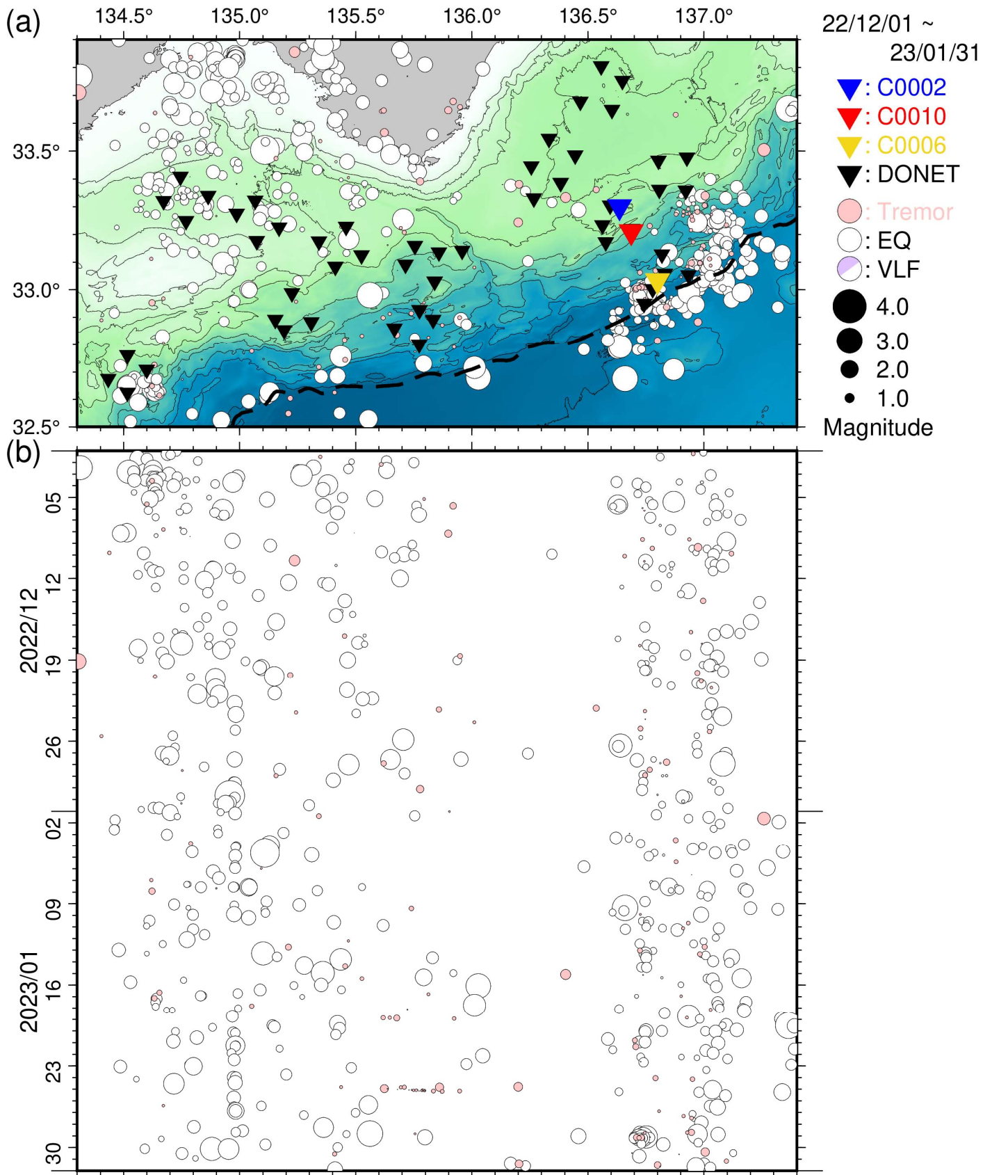
図5 直近2ヵ月間において熊野灘から室戸沖にて発生した低周波微動・通常地震・超低周波地震 (2022年12月1日~2023年1月31日)。図3と同様のシンボルにて表示。(a) 震央分布図。(b) aに示した震央を経度方向へ投影した時空間分布図。
