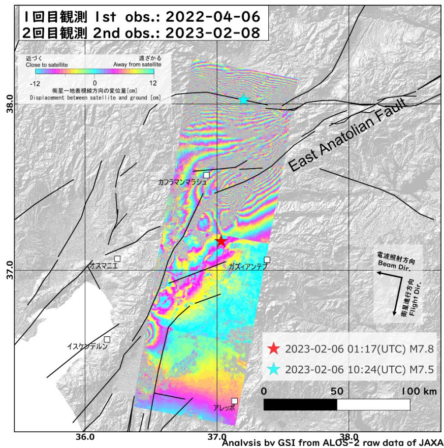
図1. SAR干渉解析結果。震央はUSGS、断層線はStyron et al. (2020)より。
