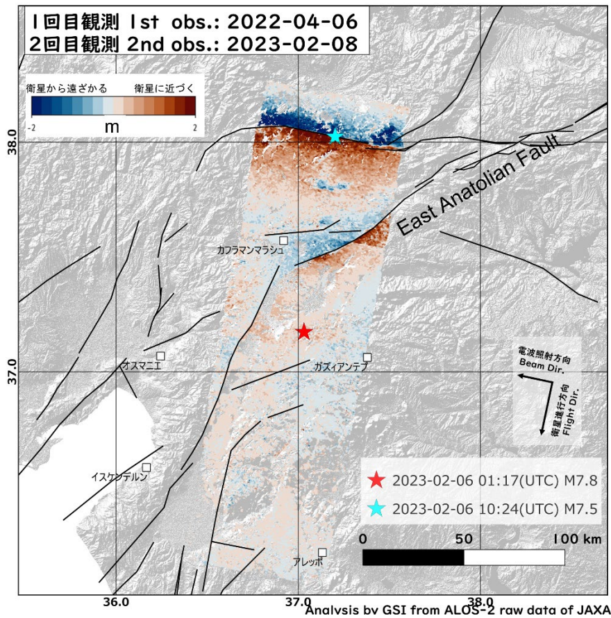
図2. ピクセルオフセット法による結果。震央はUSGS、断層線はStyron et al. (2020)より。
