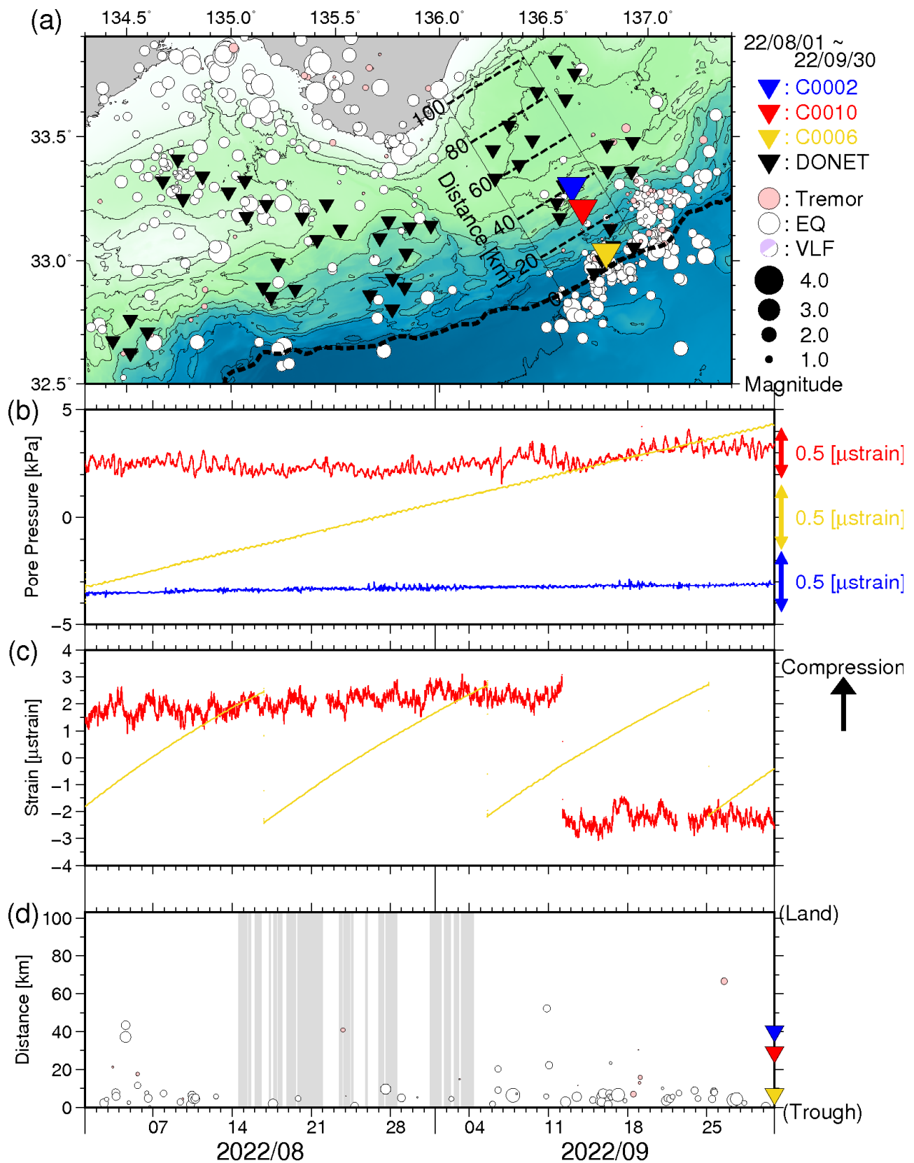
図3 直近2ヶ月間のSSE・低周波微動モニタリング(2022年8月1日~2022年9月30日)。(a) 震央分布図(●:低周波微動(深さ0~15km)、○:通常地震(深さ0~60km)、●:超低周波地震のメカニズム解)。▼▼▼▼は、それぞれC0002・C0010・C0006・DONET観測点。破線はトラフ軸。(b)長期孔内観測点における間隙水圧変化(—:C0002、—:C0010、—:C0006)。(c)長期孔内観測点における体積歪変化(—:C0010、—:C0006)。(d)図3a中に実線で示した矩形領域内における、低周波微動・通常地震・超低周波地震の時空間分布。灰色はエアガン発振期間。縦軸は、トラフ軸からの距離(km)。
