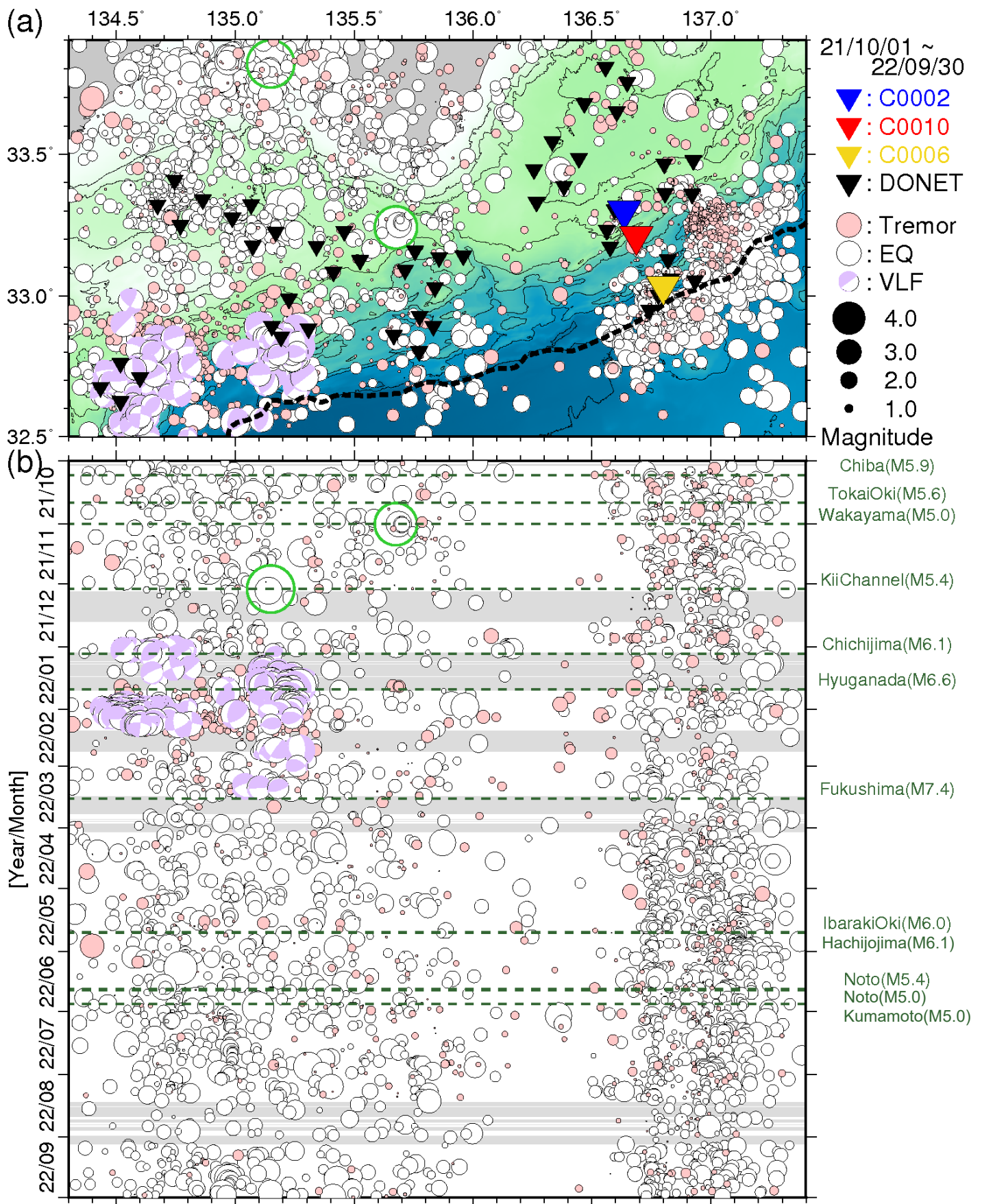
図 6 直近 1 年間に於いて熊野灘から室戸沖にて発生した低周波微動・通常地震・超低周波地震 (2021 年 10 月 1 日~2022 年 9 月 30 日)。図 4 と同様のシンボルにて表示。(a) 震央分布図。(b) a に示した震央を経度方向へ投影した時空間分布図。
