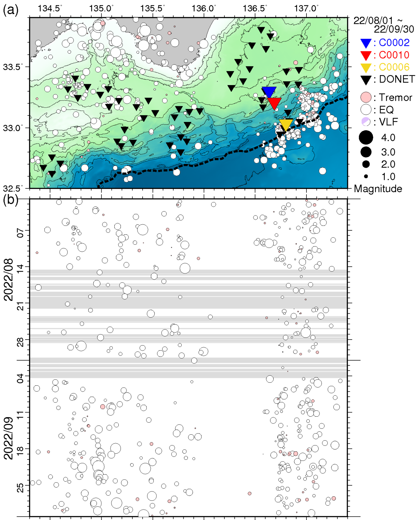
図5 直近2ヵ月間において熊野灘から室戸沖にて発生した低周波微動・通常地震・超低周波地震 (2022年8月1日～2022年9月30日)。図3と同様のシンボルにて表示。(a) 震央分布図。(b) aに示した震央を経度方向へ投影した時空間分布図。
