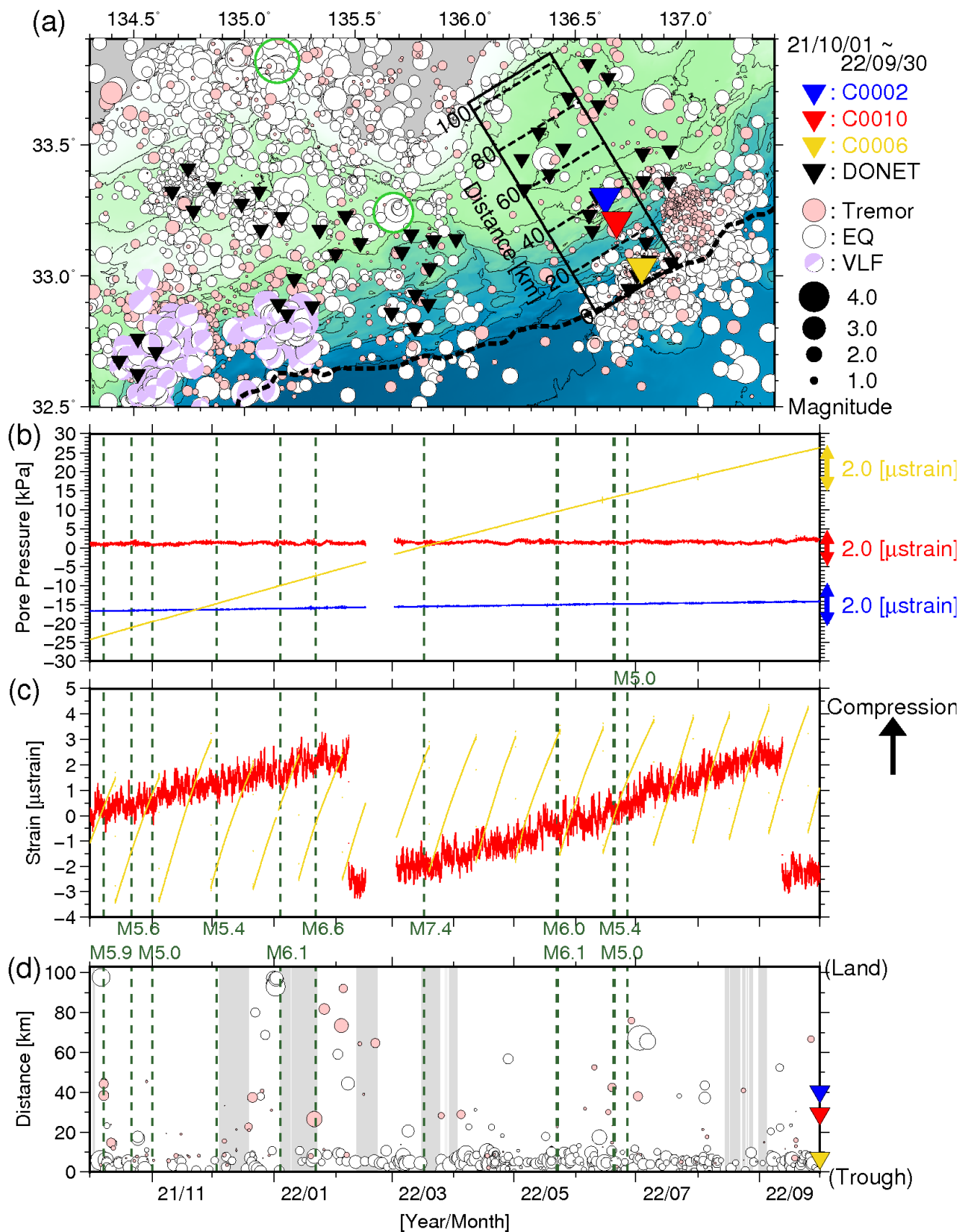
図4 直近1年間のSSE・低周波微動モニタリング(2021年10月1日~2022年9月30日)。(a)低周波微動・通常地震・超低周波地震の震央分布。(b)間隙水圧変化。(c)体積歪変化。(d)時空間分布。灰色はエアガン発振期間を示す。(b-d)の緑点線は、10月7日千葉県北西部地震、10月21日東海道南方沖地震、11月1日和歌山県南方沖地震、12月3日紀伊水道地震、1月4日父島近海地震、1月22日日向灘地震、3月16日福島県沖地震、5月22日茨城県沖地震、5月23日八丈島東方沖地震、6月19日・20日能登地方地震、及び6月26日熊本地方地震。
