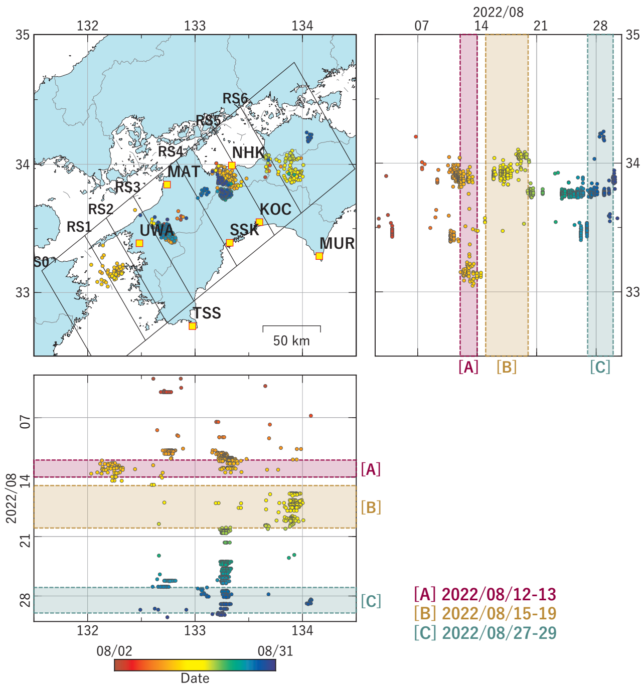
図1 四国地方における深部低周波地震の時空間分布図。 (2022/08/02 00:00 - 2022/08/31 00:00 (JST)) 気象庁カタログによる。
