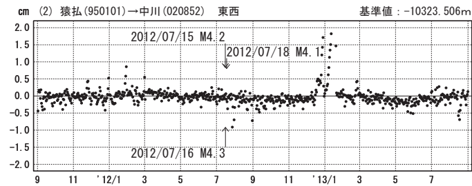
2012年7月の地震活動
