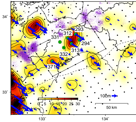
すべり量（カラー）及びすべりベクトルは水平面に投影したものを示す。 推定したすべり量が標準偏差（ \sigma ）の3倍以上のグリッドを青色表示している。
