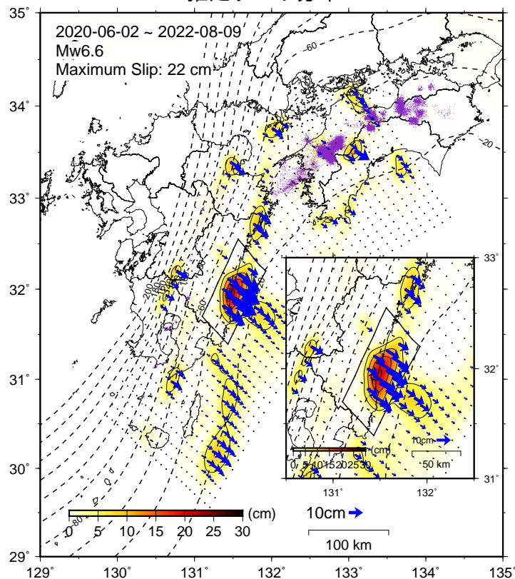
推定すべり分布
