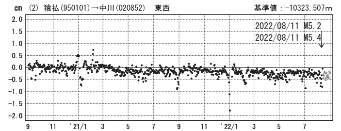
2022年8月の地震活動
