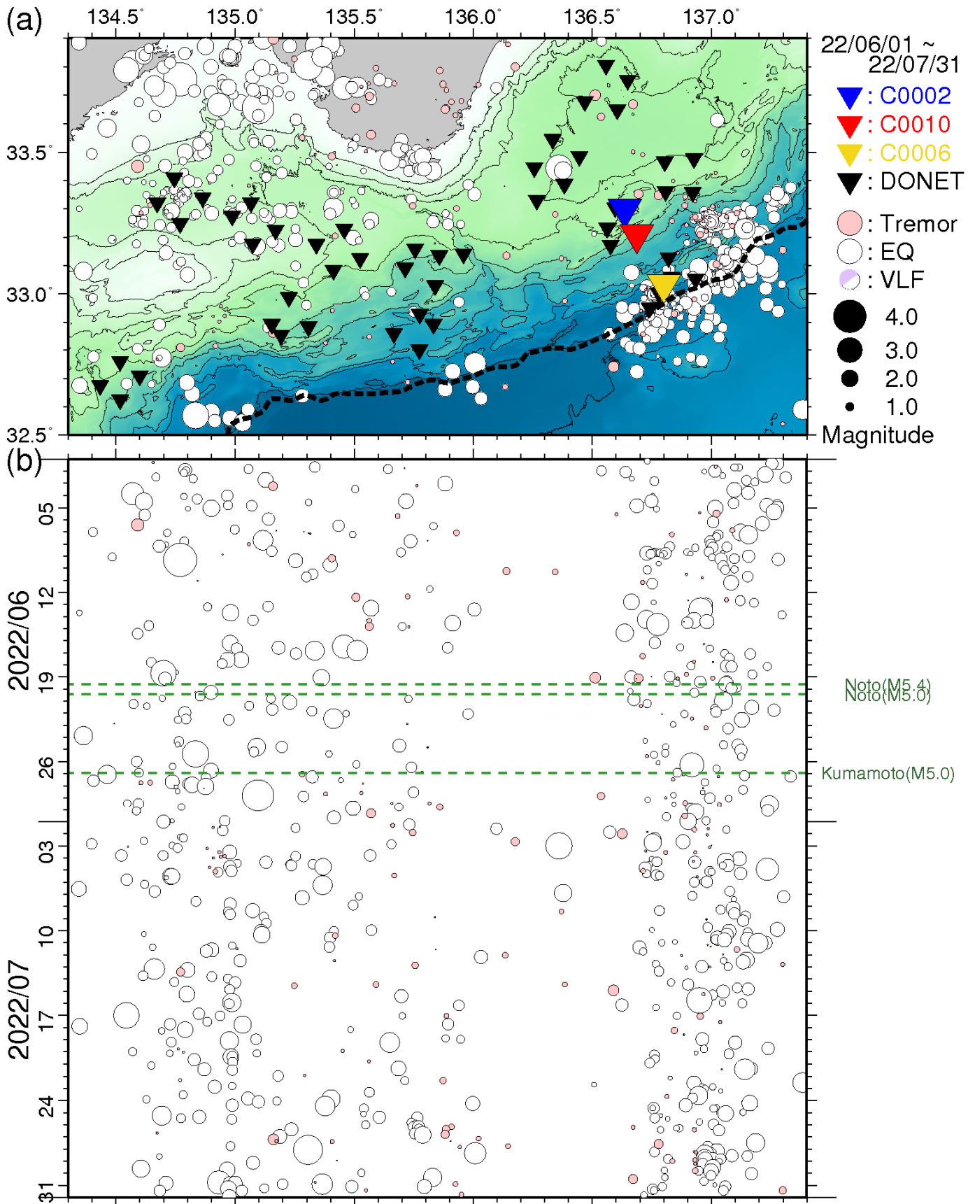
図5 直近2ヵ月間において熊野灘から室戸沖にて発生した低周波微動・通常地震・超低周波地震(2022年6月1日~2022年7月31日)。図3と同様のシンボルにて表示。(a)震央分布図。(b)aに示した震央を経度方向へ投影した時空間分布図。
