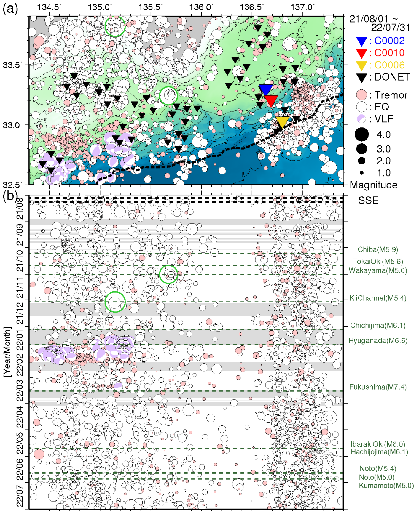
図 6 直近 1 年間に於いて熊野灘から室戸沖にて発生した低周波微動・通常地震・超低周波地震 (2021 年 8 月 1 日~2022 年 7 月 31 日)。図 4 と同様のシンボルにて表示。(a) 震央分布図。(b) a に示した震央を経度方向へ投影した時空間分布図。
