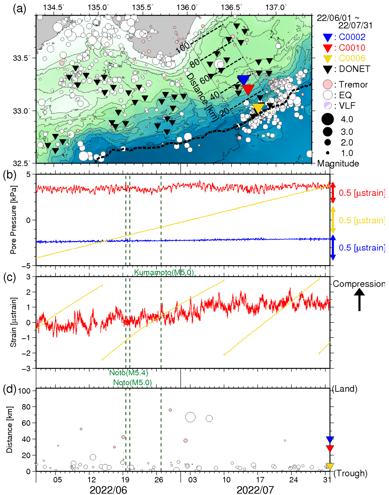
図3 直近2ヶ月間のSSE・低周波微動モニタリング(2022年6月1日~2022年7月31日)。(a) 震央分布図(●:低周波微動(深さ0~15km)、○:通常地震(深さ0~60km)、●:超低周波地震のメカニズム解)。 \blacktriangledown \blacktriangledown \blacktriangledown \blacktriangledown は、それぞれC0002・C0010・C0006・DONET観測点。破線はトラフ軸。(b)長期孔内観測点における間隙水圧変化(—:C0002、—:C0010、—:C0006)。(c)長期孔内観測点における体積歪変化(—:C0010、—:C0006)。(d)図3a中に実線で示した矩形領域内における、低周波微動・通常地震・超低周波地震の時空間分布。灰色はエアガン発振期間。縦軸は、トラフ軸からの距離(km)。(b-d)の緑点線は、6月19日・20日能登地方地震、及び6月26日熊本地方地震。
