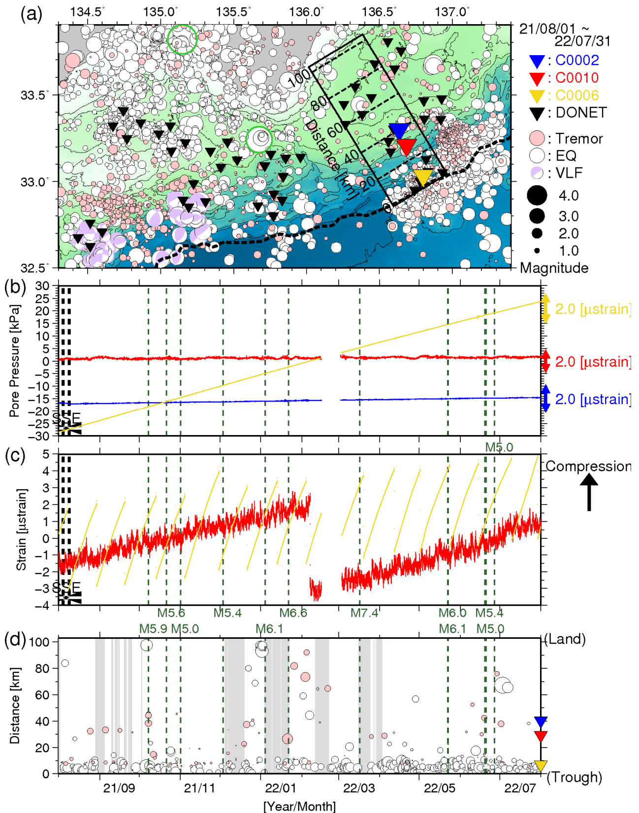
図4 直近1年間のSSE・低周波微動モニタリング(2021年8月1日~2022年7月31日)。(a)低周波微動・通常地震・超低周波地震の震央分布。(b)間隙水圧変化。(c)体積歪変化。(d)時空間分布。灰色はエアガン発振期間を示す。(b-d)の緑点線は、10月7日千葉県北西部地震、10月21日東海道南方沖地震、11月1日和歌山県南方沖地震、12月3日紀伊水道地震、1月4日父島近海地震、1月22日日向灘地震、3月16日福島県沖地震、5月22日茨城県沖地震、5月23日八丈島東方沖地震、6月19日・20日能登地方地震、及び6月26日熊本地方地震。
