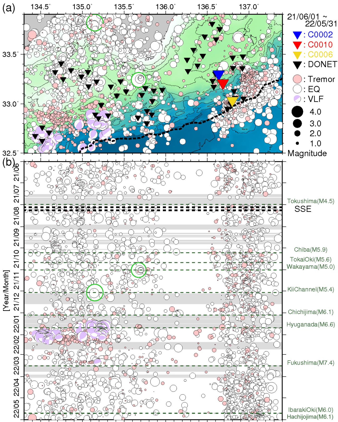
図 6 直近 1 年間に於いて熊野灘から室戸沖にて発生した低周波微動・通常地震・超低周波地震 (2021 年 6 月 1 日~2022 年 5 月 31 日)。図 4 と同様のシンボルにて表示。(a) 震央分布図。(b) a に示した震央を経度方向へ投影した時空間分布図。
