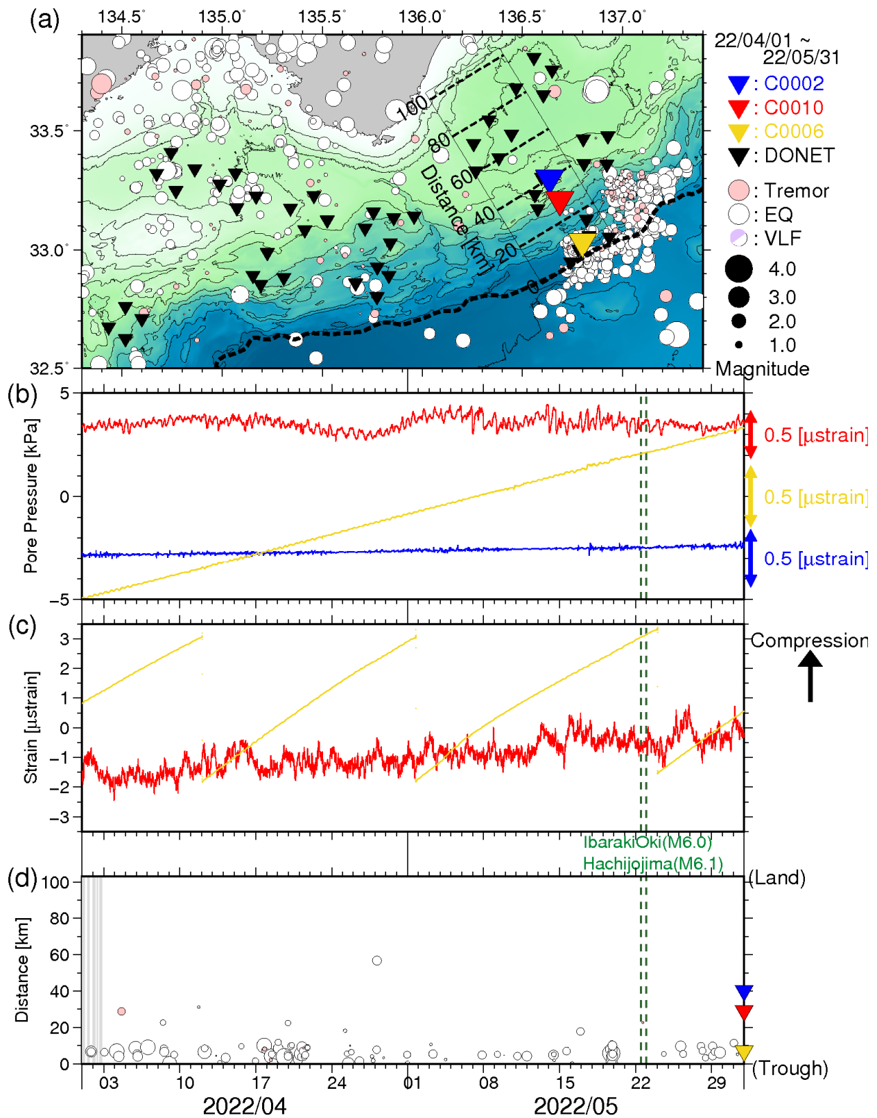
図3 直近2ヶ月間のSSE・低周波微動モニタリング(2022年4月1日~2022年5月31日)。(a) 震央分布図(●:低周波微動(深さ0~15km)、○:通常地震(深さ0~60km)、●:超低周波地震のメカニズム解)。▼▼▼▼は、それぞれC0002・C0010・C0006・DONET観測点。破線はトラフ軸。(b) 長期孔内観測点における間隙水圧変化(—:C0002、—:C0010、—:C0006)。(c) 長期孔内観測点における体積歪変化(—:C0010、—:C0006)。(d) 図3a中に実線で示した矩形領域内における、低周波微動・通常地震・超低周波地震の時空間分布。灰色はエアガン発振期間。縦軸は、トラフ軸からの距離(km)。(b-d)の緑点線は、5月22日茨城県沖地震、及び5月23日八丈島東方沖地震。
