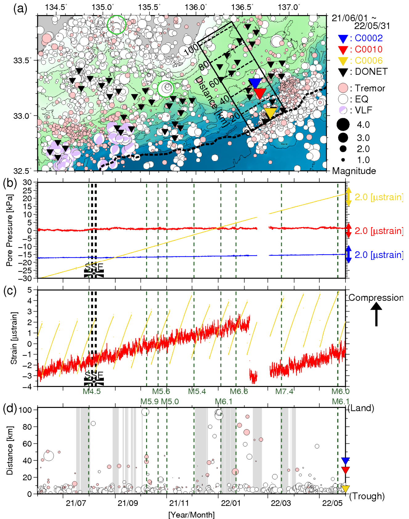
図4 直近1年間のSSE・低周波微動モニタリング(2021年6月1日~2022年5月31日)。(a) 低周波微動・通常地震・超低周波地震の震央分布。(b) 間隙水圧変化。(c) 体積歪変化。(d) 時空間分布。灰色はエアガン発振期間を示す。(b-d)の緑点線は、7月31日徳島県南部地震、10月7日千葉県北西部地震、10月21日東海道南方沖地震、11月1日和歌山県南方沖地震、12月3日紀伊水道地震、1月4日父島近海地震、1月22日日向灘地震、3月16日福島県沖地震、5月22日茨城県沖地震、及び5月23日八丈島東方沖地震。
