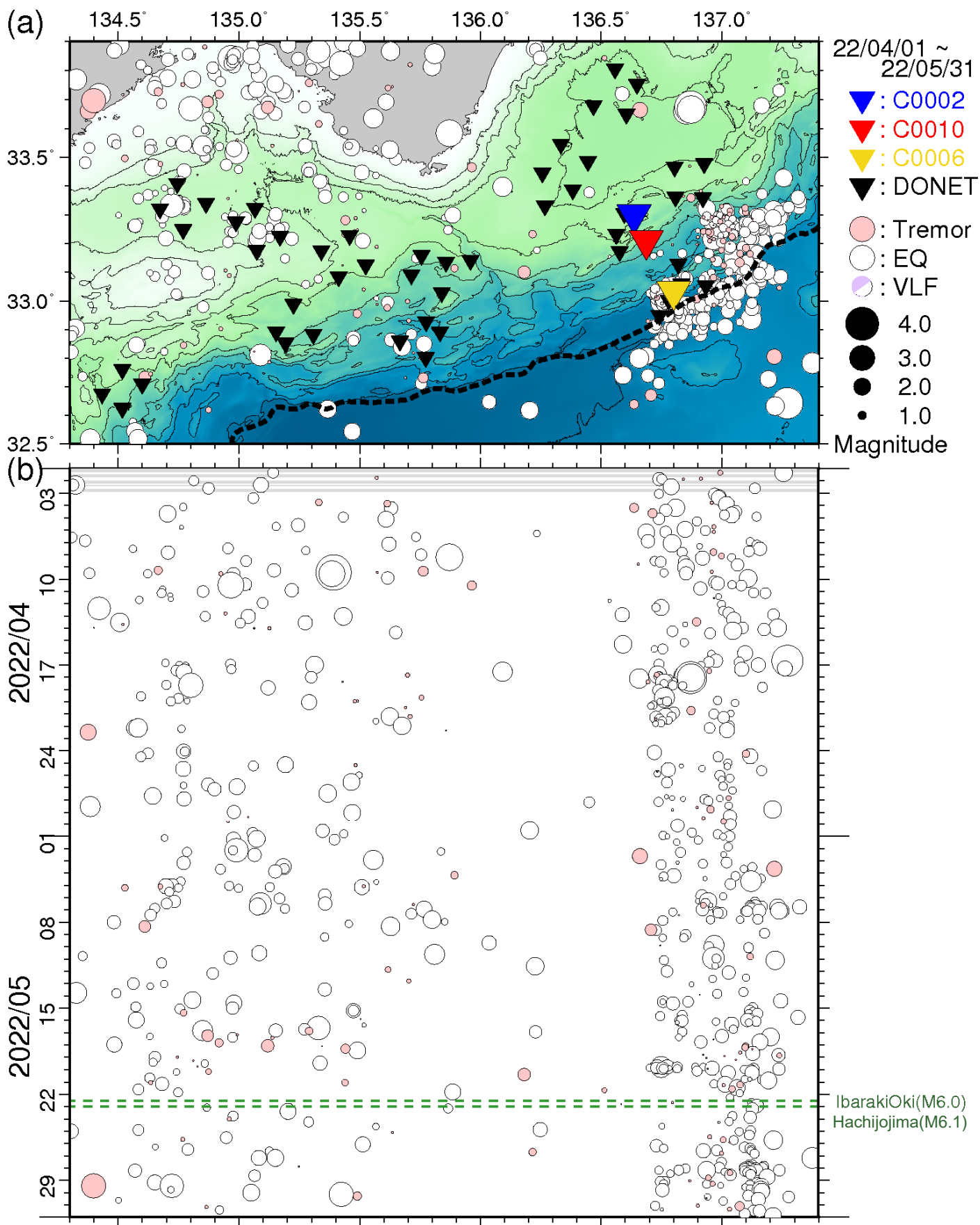
図5 直近2ヵ月間において熊野灘から室戸沖にて発生した低周波微動・通常地震・超低周波地震 (2022年4月1日~2022年5月31日)。図3と同様のシンボルにて表示。(a) 震央分布図。(b) aに示した震央を経度方向へ投影した時空間分布図。
