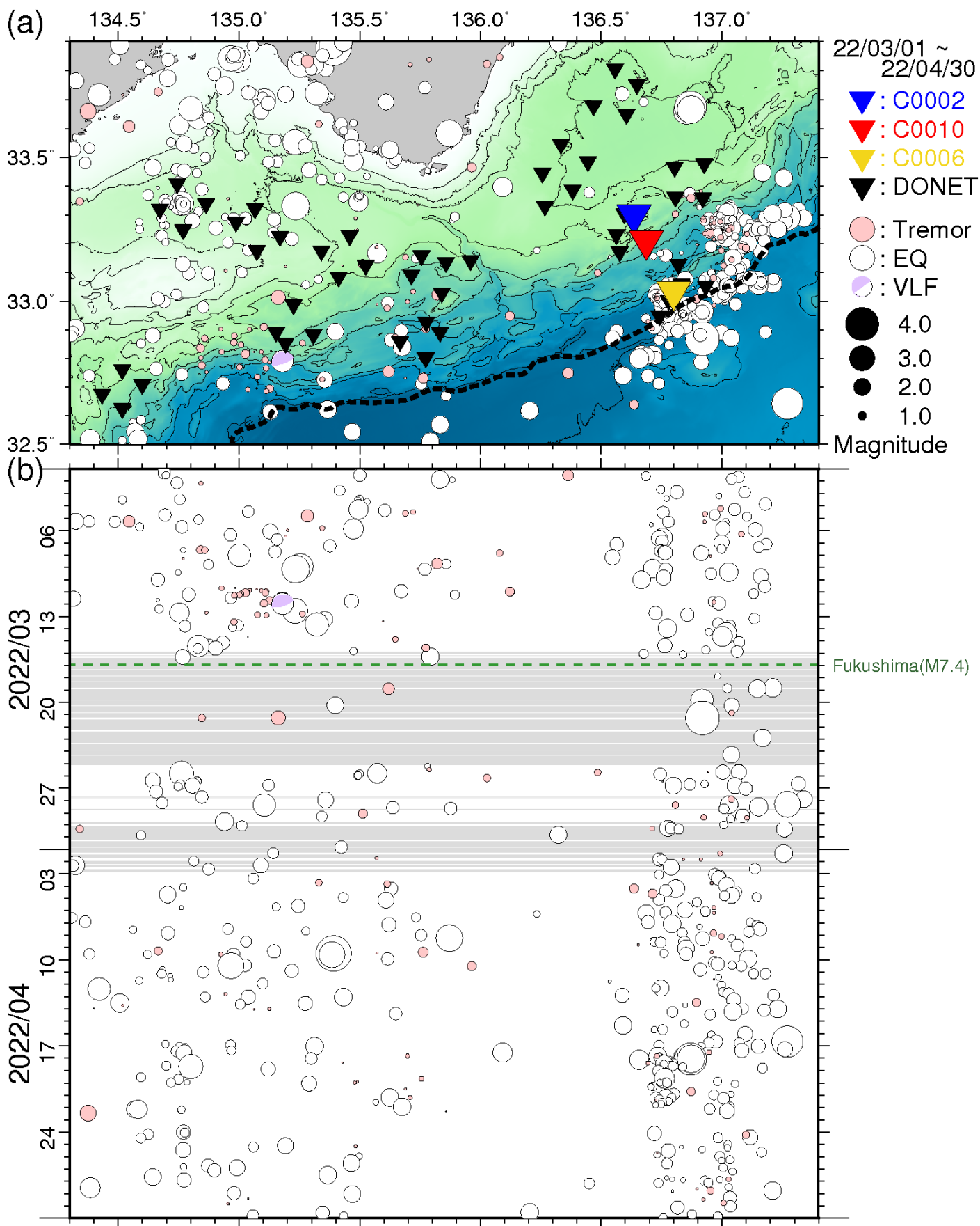
図5 直近2ヵ月間において熊野灘から室戸沖にて発生した低周波微動・通常地震・超低周波地震 (2022年3月1日～2022年4月30日)。図3と同様のシンボルにて表示。(a) 震央分布図。(b) aに示した震央を経度方向へ投影した時空間分布図。
