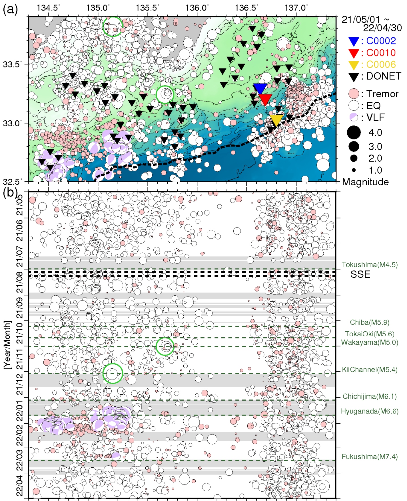
図 6 直近 1 年間に於いて熊野灘から室戸沖にて発生した低周波微動・通常地震・超低周波地震 (2021 年 5 月 1 日~2022 年 4 月 30 日)。図 4 と同様のシンボルにて表示。(a) 震央分布図。(b) a に示した震央を経度方向へ投影した時空間分布図。
