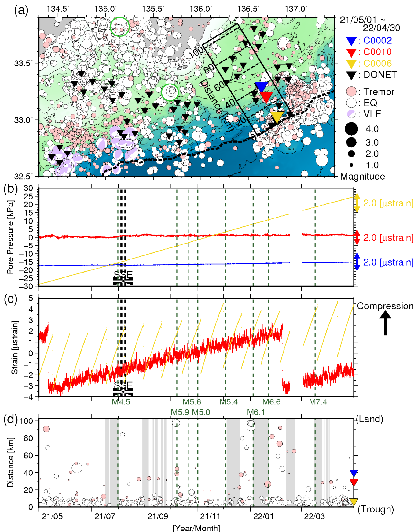
図4 直近1年間のSSE・低周波微動モニタリング(2021年5月1日~2022年4月30日)。(a) 低周波微動・通常地震・超低周波地震の震央分布。(b) 間隙水圧変化。(c) 体積歪変化。(d) 時空間分布。灰色はエアガン発振期間を示す。(b-d)の緑点線は、7月31日徳島県南部地震、10月7日千葉県北西部地震、10月21日東海道南方沖地震、11月1日和歌山県南方沖地震、12月3日紀伊水道地震、1月4日父島近海地震、1月22日日向灘地震、及び3月16日福島県沖地震。
