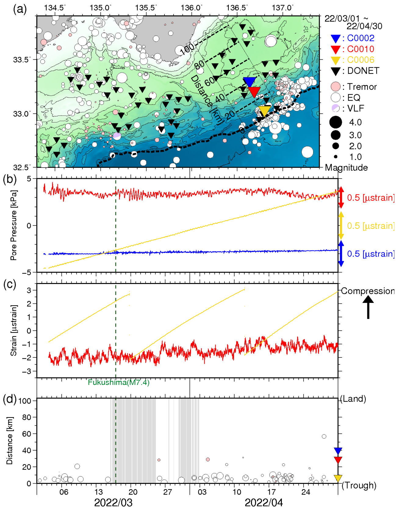
図3 直近2ヶ月間のSSE・低周波微動モニタリング(2022年3月1日~2022年4月30日)。(a) 震央分布図(●:低周波微動(深さ0~15km)、○:通常地震(深さ0~60km)、●:超低周波地震のメカニズム解)。▼▼▼▼は、それぞれC0002・C0010・C0006・DONET観測点。破線はトラフ軸。(b)長期孔内観測点における間隙水圧変化(—:C0002、—:C0010、—:C0006)。(c)長期孔内観測点における体積歪変化(—:C0010、—:C0006)。(d)図3a中に実線で示した矩形領域内における、低周波微動・通常地震・超低周波地震の時空間分布。灰色はエアガン発振期間。縦軸は、トラフ軸からの距離(km)。(b-d)の緑点線は、3月16日福島県沖地震。
