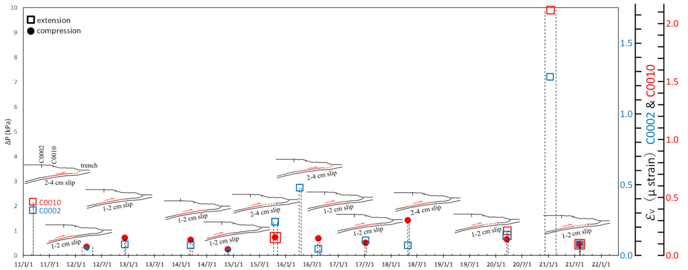
図7 孔内観測点において観測された SSE 発生時の間隙水圧変化 (Araki et al., 2017; Ariyoshi et al. 2021) を加筆・修正)。間隙水圧変化 ( \Delta P ) とそれらを体積歪 ( \varepsilon_v ) に換算したスケールを縦軸に示している。●・□は、それぞれ圧縮・伸長方向の間隙水圧変化を示す。青・赤のシンボルは、それぞれ C0002・C0010 の間隙水圧変化を示す。
