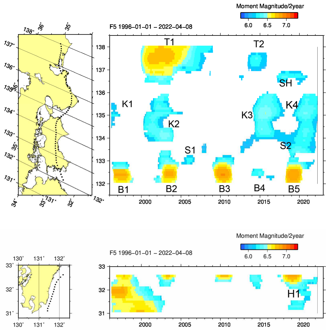
第2図 長期的スロースリップの規模分布（1996年から2022年4月） 2年間あたりの変化量から推定したモーメントマグニチュード。地域略号は第1図と同じ。
