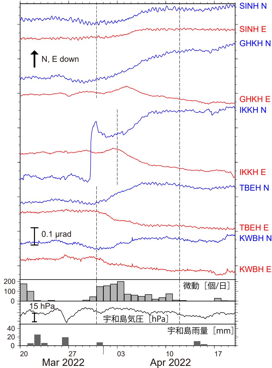
図1: 2022年3月20日~4月19日の傾斜時系列。上方向への変化が北・東下がりの傾斜変動を表し、BAYTAP-Gにより潮汐・気圧応答成分を除去した。3月31日 (IKKHは4月3日) ~ 4月11日の傾斜変化ベクトルを図2に示す。四国中西部での微動活動度・気象庁宇和島観測点の気圧・雨量をあわせて示す。
