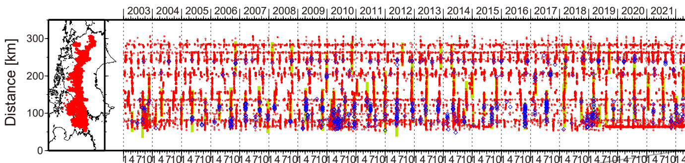
図1. 四国における2003年1月～2022年5月8日までの深部低周波微動の時空間分布(上図). 赤丸はエンベロープ相関・振幅ハイブリッド法 (Maeda and Obara, 2009) およびクラスタ処理 (Obara et al., 2010) によって1時間毎に自動処理された微動分布の重心である. 青菱形は
