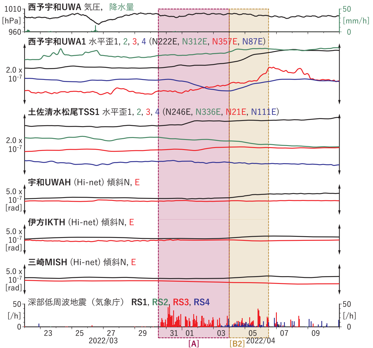
図2 歪・傾斜の時間変化(2) (2022/03/22 00:00-2022/04/11 00:00 (JST))
