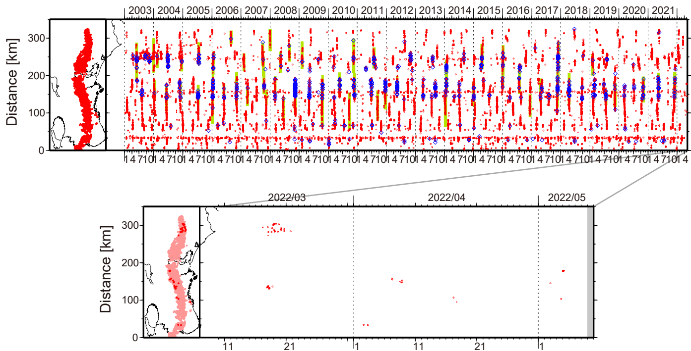
図1. 紀伊半島・東海地域における2003年1月～2022年5月8日までの深部低周波微動の時空間分布(上図)。赤丸はエンベロープ相関・振幅ハイブリッド法(Maeda and Obara, 2009)およびクラスタ処理(Obara et al., 2010)によって1時間毎に自動処理された微動分布の重心である。青菱形は周期20秒に卓越する超低周波地震(Ito et al., 2007)である。黄緑色の太線はこれまでに検出された短期的スロースリップイベント(SSE)を示す。下図は2022年4月を中心とした期間の拡大図である。4月以降の期間について顕著な活動はとくにみられなかったものの、4月8日頃に三重県中部において、5月5日頃に三重県北部において、それぞれごく小規模な活動がみられた。
