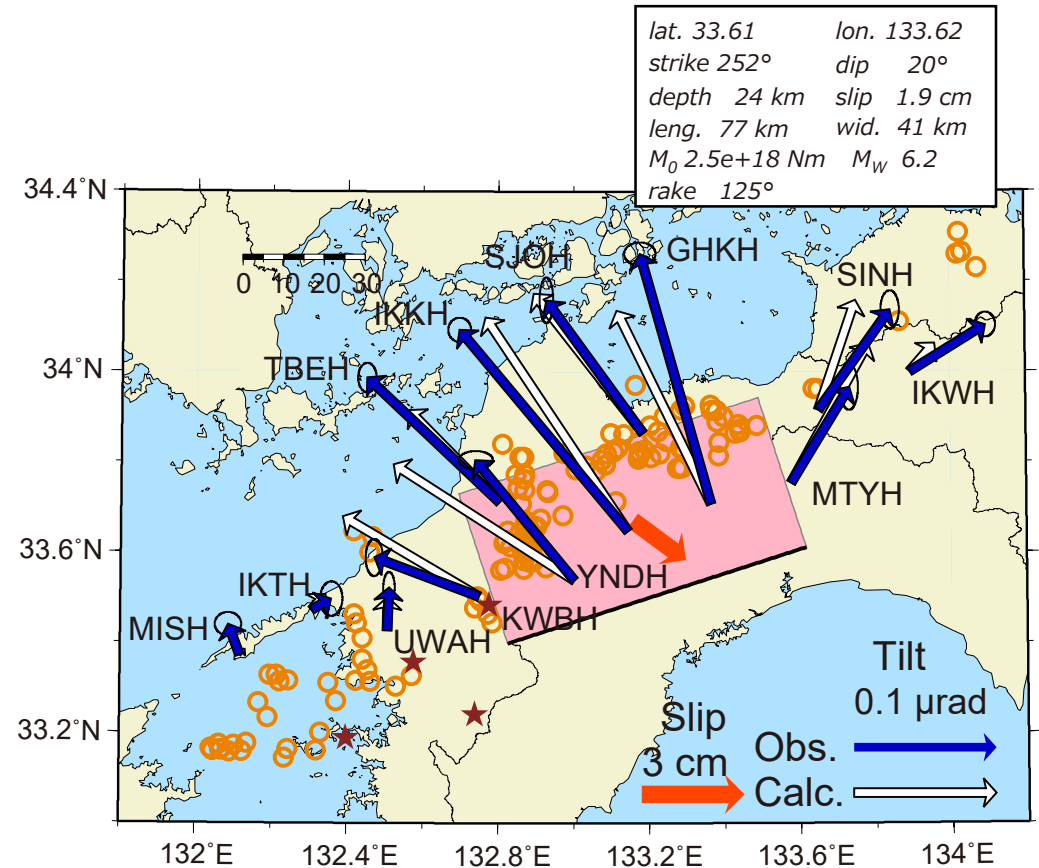
図2: 3月31日 (IKKHは4月3日) ~ 4月11日に観測された傾斜変化ベクトル(青矢印), 推定されたスロースリップイベントの断層モデル(赤矩形・矢印), モデルから計算される傾斜変化ベクトル(白抜き矢印)を示す。1時間ごとの微動エネルギーの重心位置(橙丸)もあわせて示す。すべり角はプレート相対運動方向に固定している。
