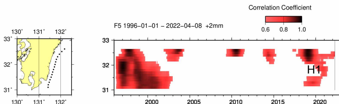
第1図 長期的スロースリップ客観検知図（1996年から2022年4月）
