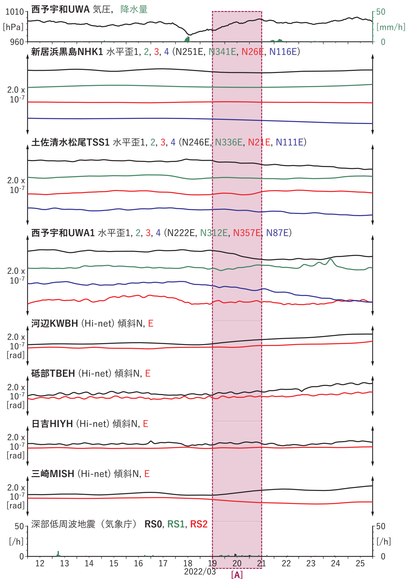
図8 歪・傾斜の時間変化 (2022/03/12 00:00-2022/03/26 00:00 (JST))
