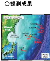
東北地方太平洋沖地震時の海底の変動
