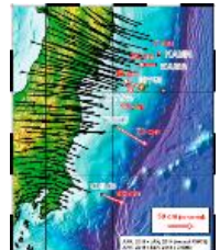
東北地方太平洋沖地震後の海底の余効変動
