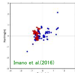
初期アレイ形状を修正することで、任意の位置からの測距ではRMS 0.5m以下の精度が得た。
