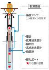
孔内観測装置構成図
