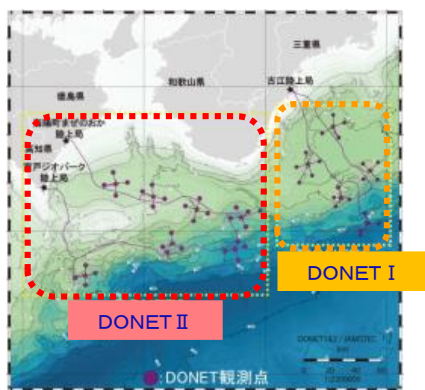
DONET1: 地震計・津波計等を22点設置
