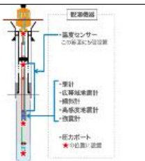
孔内観測装置構成図
