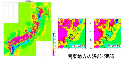
全国深部地盤モデル(地震基盤面深さ)
