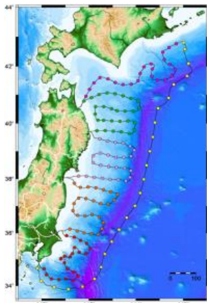
日本海溝海底地震津波観測網 (S-net) 地震計・津波計等を150点設置
