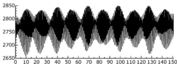
海底局の水圧計によって観測されたデータ (横軸は日、縦軸はm)
