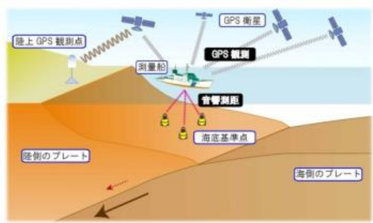
GNSS-音響測距結合方式による海底地殻変動観測
