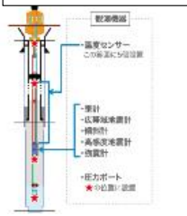
孔内観測装置構成図
