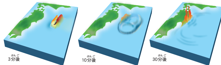
※上の図は1896年明治三陸地震の津波が伝わる様子のシミュレーションを示します。 古村孝志氏（東京大学地震研究所）らによる
