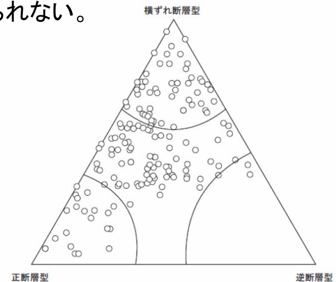
図9-2 発震機構の分布
