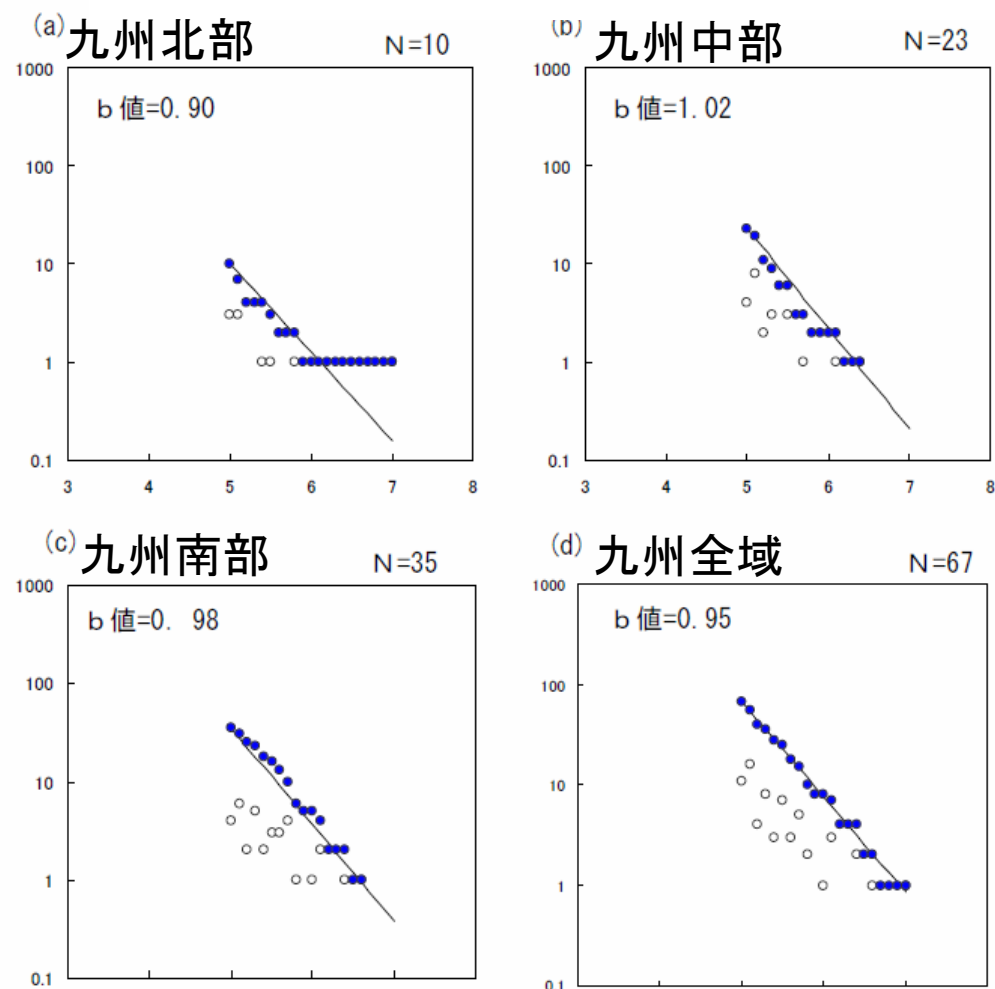
図21 図10に基づく1923ー2011年の88年間に観測されたM5.0以上の地震に対する地震規模と規模別頻度数の経験式(G-R式)の回帰結果
