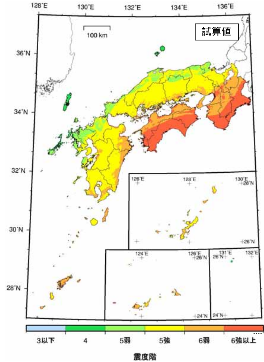
図 2b 今後 30 年以内に 3% の確率で一定の震度以上の揺れに見舞われる領域：再現期間 1000 年に相当*** (試算値)
