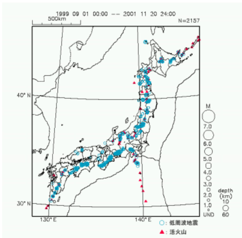
図 2 低周波地震の発生の分布(気象庁)
