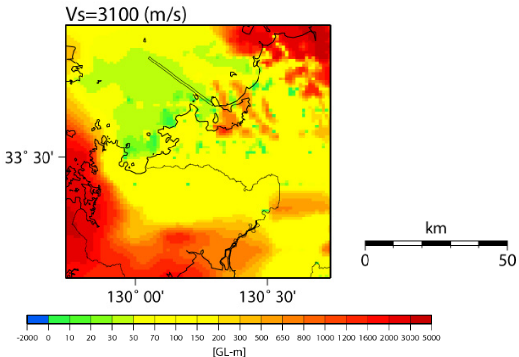
図 11 「深い地盤構造」の1次モデルの地震基盤層 ( V_s=3,000\text{m/s} ) 上面の深さ分布
