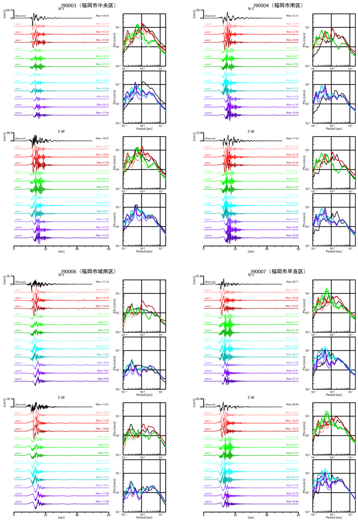
図 36-2 2005 年福岡県西方沖の地震の観測記録と計算結果との比較
