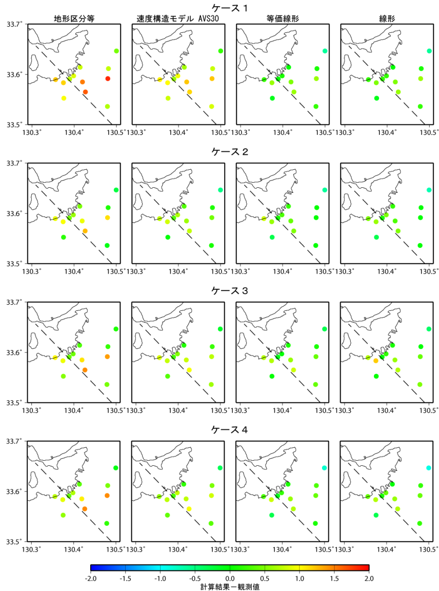
図 35 2005 年福岡県西方沖の地震の観測記録と計算結果との比較 (計測震度の差。観測点位置は図 36 を参照)
